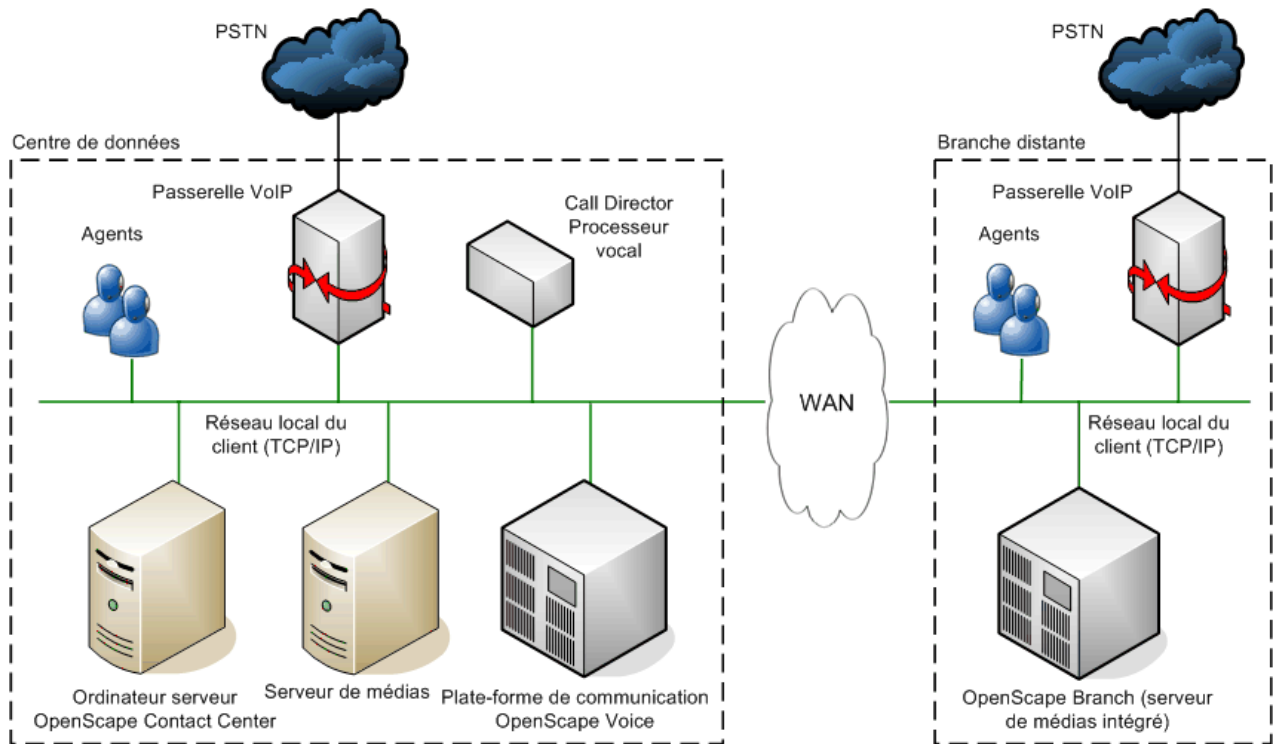
Figure 1 Configuration du réseau avec OpenScape Branch
