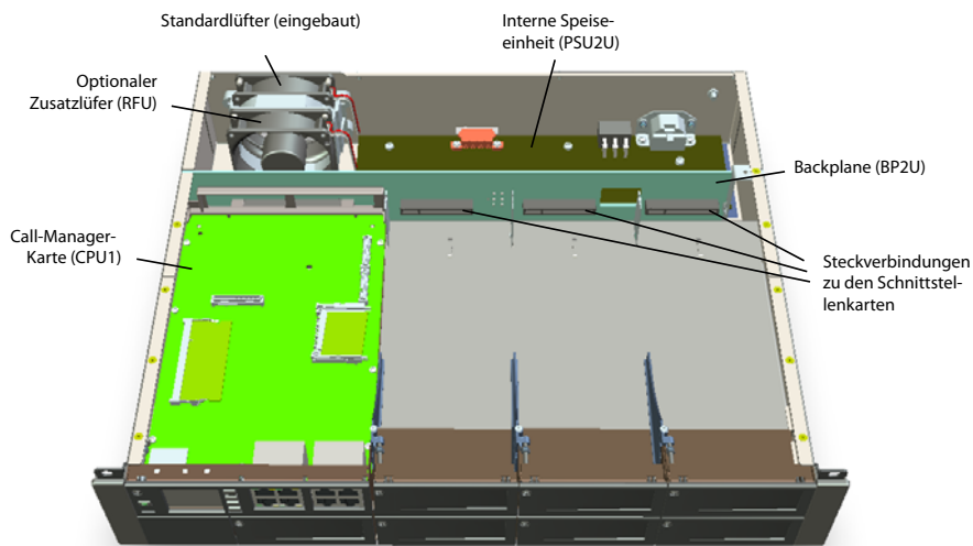
Fig. 7 Basissystem Mitel 470 mit bestücktem Zusatzlüfter
