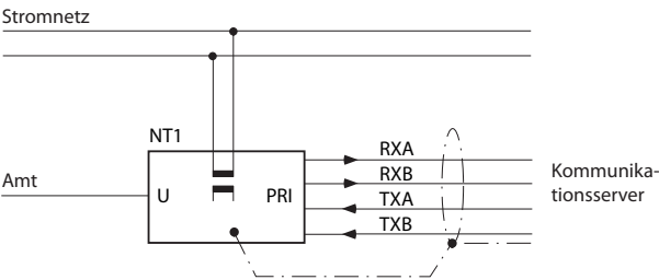
Fig. 40 Primärratenanschluss PRI am NT1
