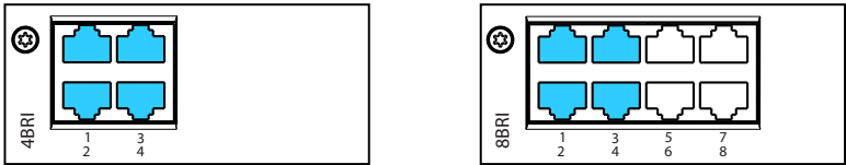
Fig. 49 Anschlussmöglichkeiten BRI-S-Endgeräteschnittstellen
