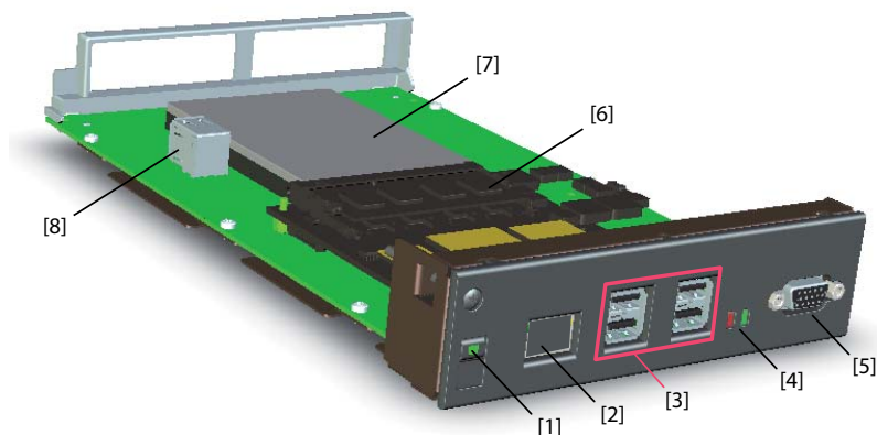
Fig. 16 Schnittstellen, Anzeige- und Bedienelemente der Applikationskarte
