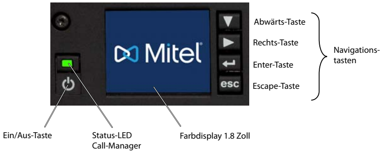
Fig. 84 Anzeige- und Bedienfeld Mitel 470
