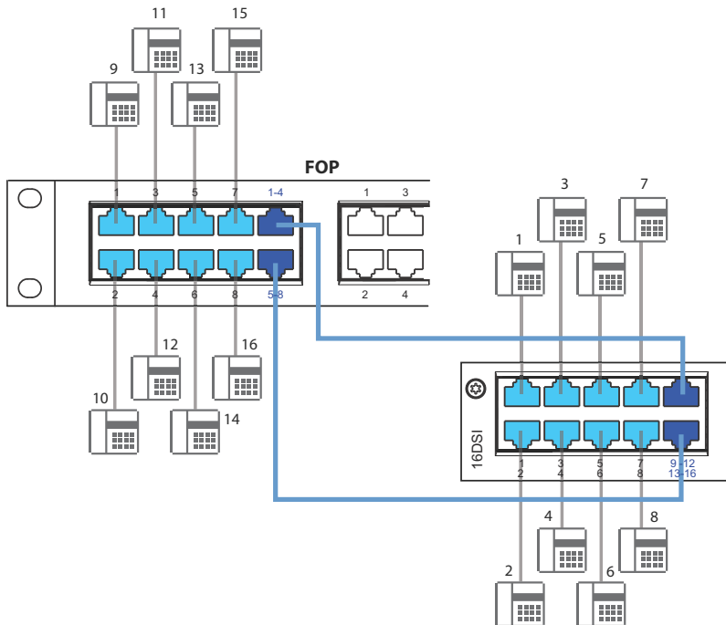
Fig. 65 Beschriftung von vierfach belegten Buchsen via Verteilpanel FOP
