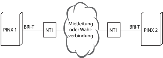
Fig. 38 Basisanschluss BRI-T Vernetzung mit Mietleitung oder Wählverbindung
