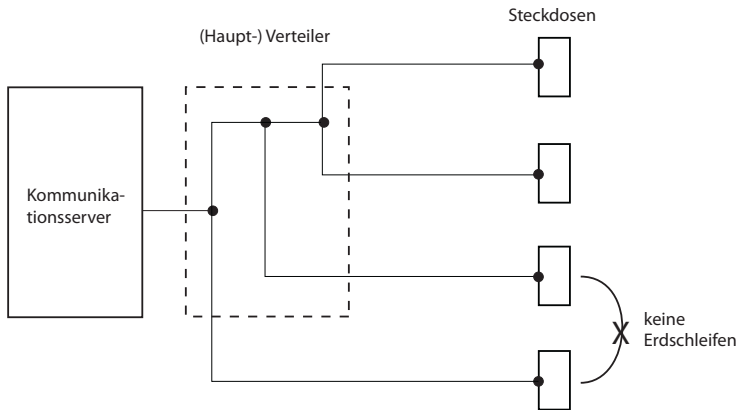
Fig. 23 Baumordnungsprinzip
