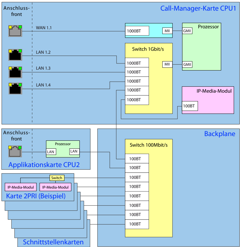
Fig. 11 Übersicht Ethernet-Konzept Mitel 470
