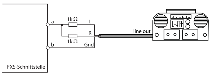
Fig. 60 Beschaltung für FXS-Modus: Externe Audioquelle
