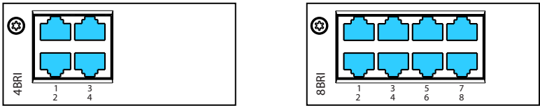
Fig. 35 Anschlussmöglichkeiten BRI-Netzschnittstellen
