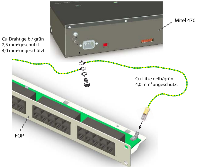
Fig. 66 Anschluss des Verteilpanels FOP an die Schutzterde
