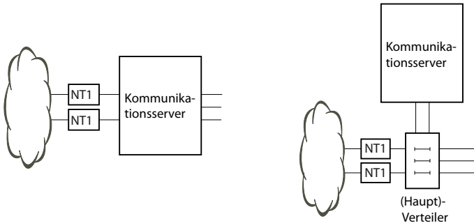
Fig. 29 Direktanschluss (links) und Indirektanschluss (rechts)
