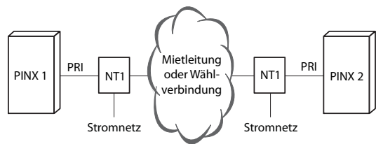
Fig. 43 Primärratenanschluss PRI Vernetzung mit Mietleitung oder Wählverbindung
