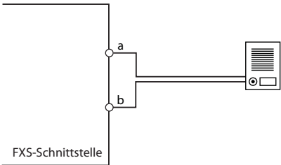
Fig. 59 Beschaltung für FXS-Modus: 2-Draht-Tür
