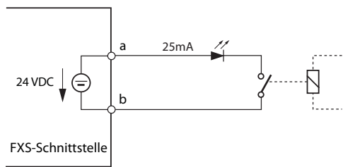
Fig. 62 Beschaltung für FXS-Modus: Steuereingang
