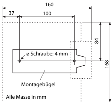
Fig. 72 Massbild für Wandmontage des Montagebügels
