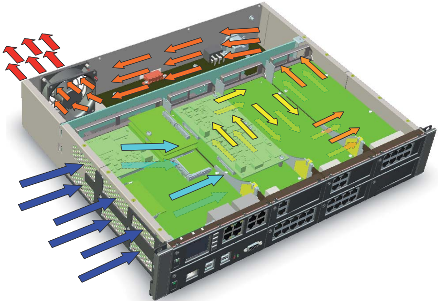
Fig. 18 Thermischer Luftstrom
