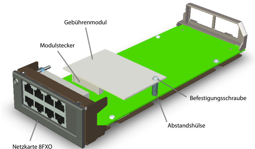
Fig. 28 Gebührenmodul auf Netzkarte 8FXO
