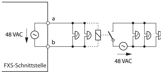
Fig. 63 Beschaltung für FXS-Modus: Zentralwecker
