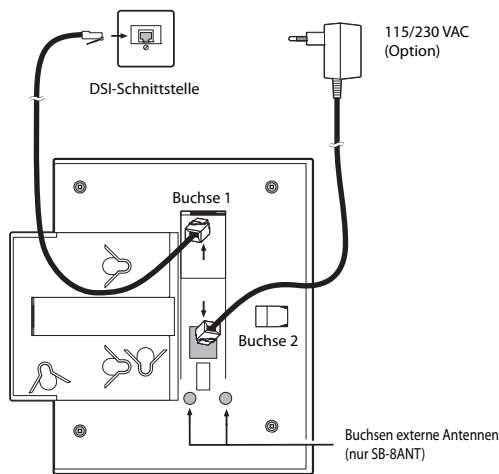
Fig. 74 Rückseite der Funkeinheiten mit Anschluss-Stellen
