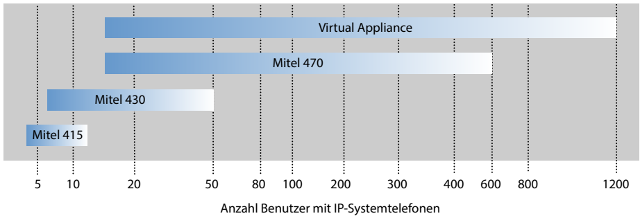
Fig. 2 MiVoice Office 400 Kommunikationsserver und ihre Ausbaupazität
