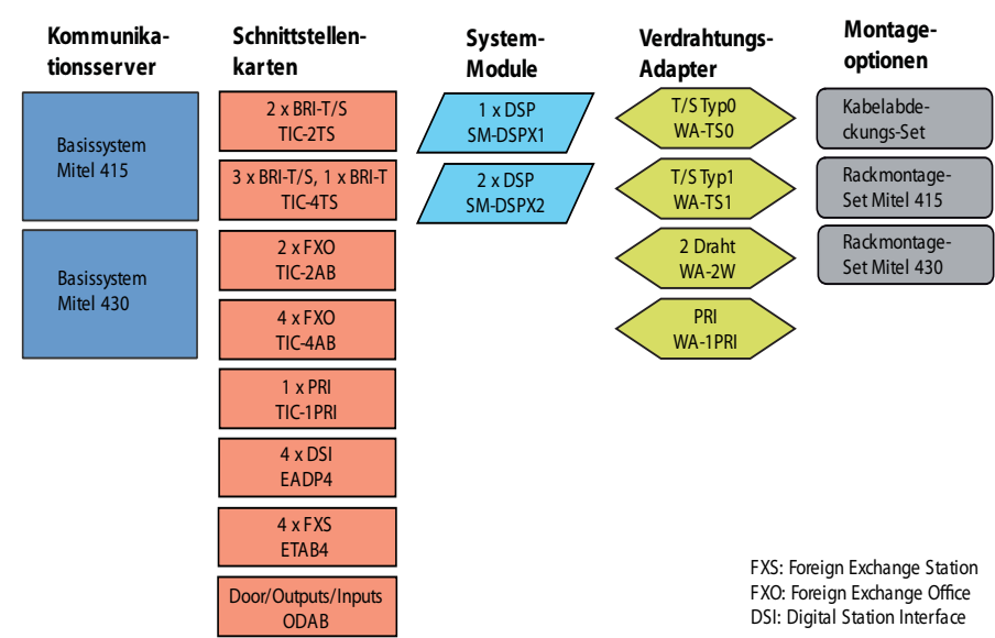
Fig. 5 Übersicht der Ausbaumöglichkeiten
