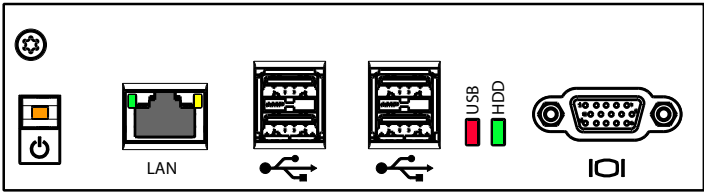
Fig. 86 Status-LEDs des Applikationsserver
