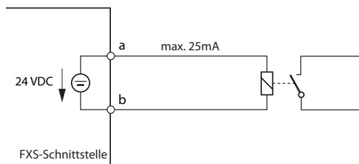
Fig. 61 Beschaltung für FXS-Modus: Steuerausgang
