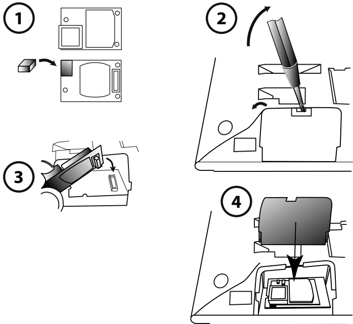
Fig. 69 Montage Bluetooth-Modul
