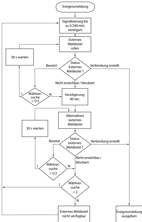
Fig. 88 Flussdiagramm Signalisierung einer Ereignismeldung an ein externes Meldeziel
