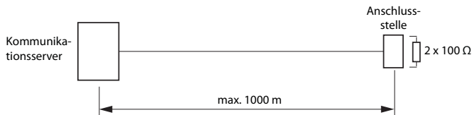
Fig. 53 S-Bus, Punkt-Punkt
