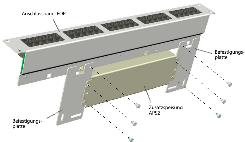
Fig. 25 Verteilpanel mit montierter Zusatzspeisung (Ansicht von unten)
