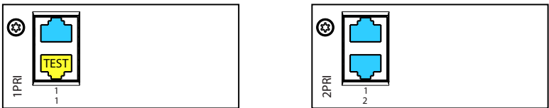
Fig. 39 Anschlussmöglichkeiten PRI-Netzschnittstellen
