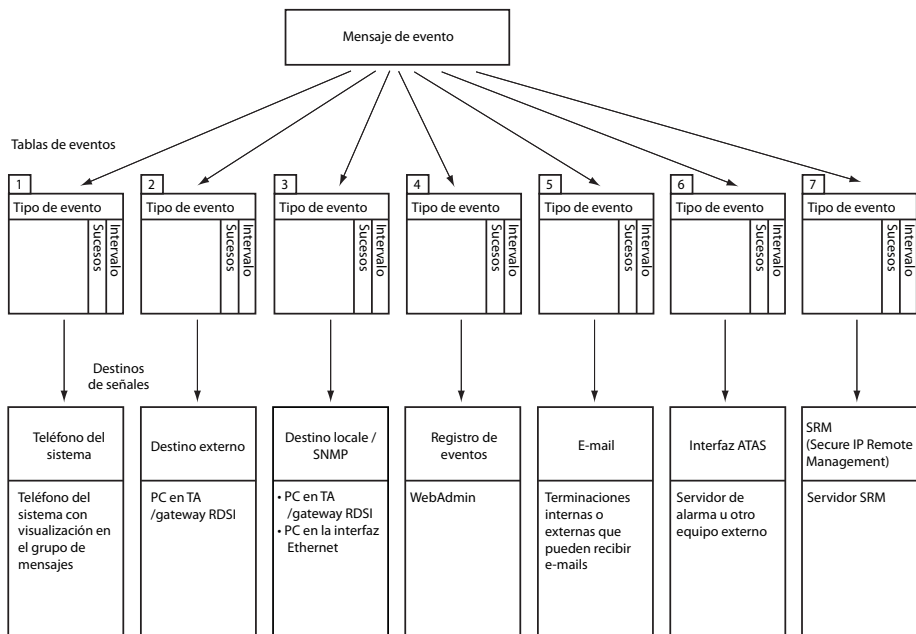
Fig. 10 Principio de distribución para un mensaje de evento
