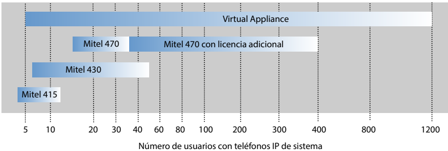
Fig. 2 Servidores de comunicaciones MiVoice Office 400 y su capacidad de expansión
