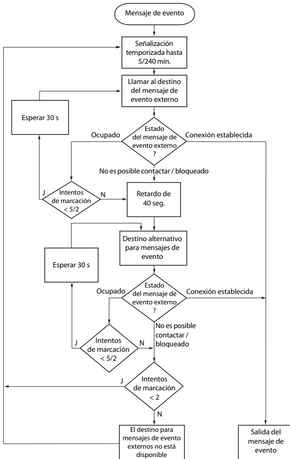
Fig. 11 Diagrama de flujo de la señalización de un mensaje de evento a un destino de señal externo
