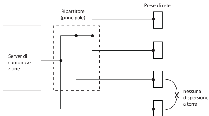
Fig. 21 Principio della struttura ad albero
