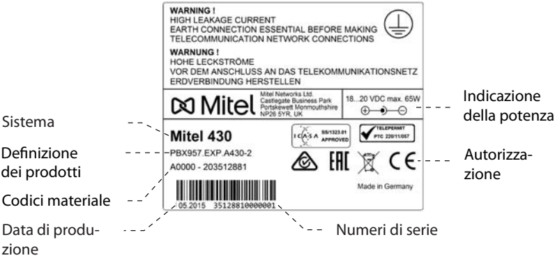
Fig. 82 Targhetta di identificazione (esempio del server di comunicazione Mitel 430)
