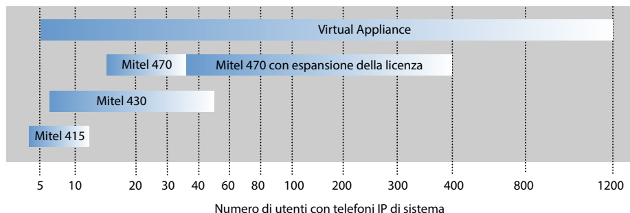
Fig. 3 Server di comunicazione MiVoice Office 400 e loro capacità
