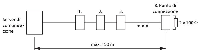
Fig. 46 Bus S corto
