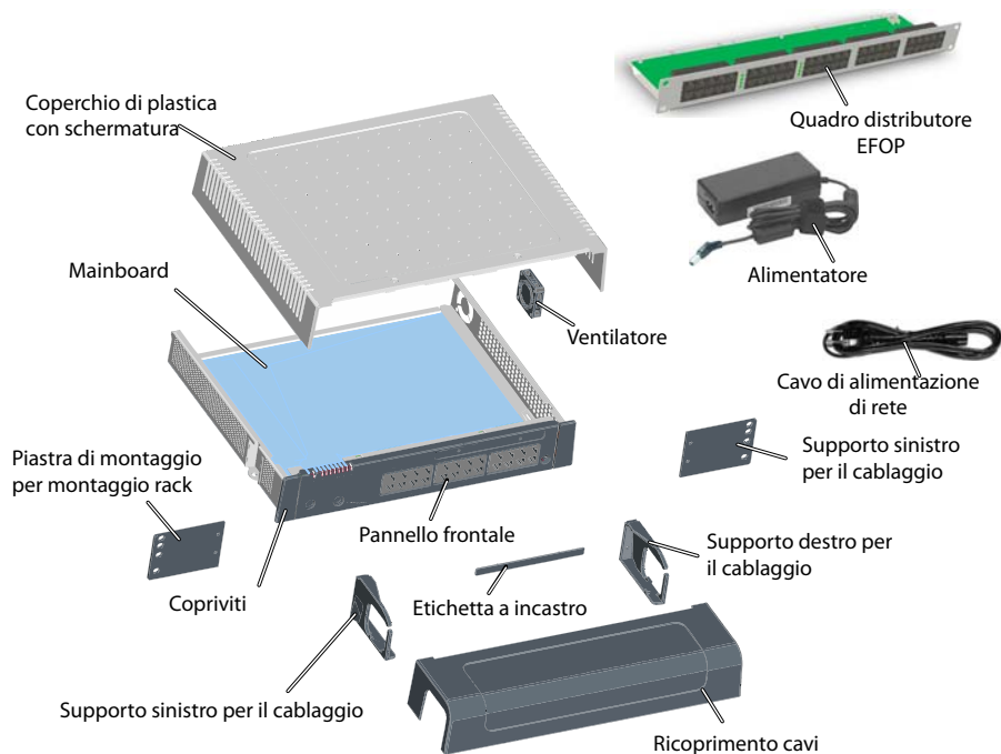
Fig. 11 Componenti del sistema con opzioni di montaggio
