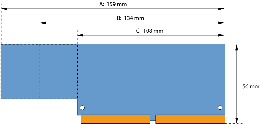
Fig. 84 Dimensioni schede di interfaccia (struttura A, B, C)
