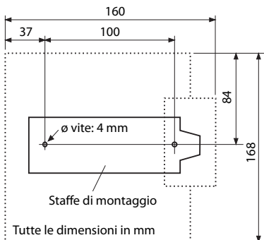
Fig. 67 Disegno e quote per il montaggio a parete della staffa
