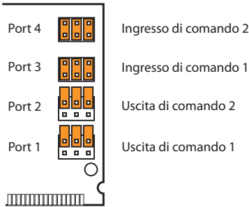
Fig. 61 Configurazione dei jumper per uscite e ingressi di comando
