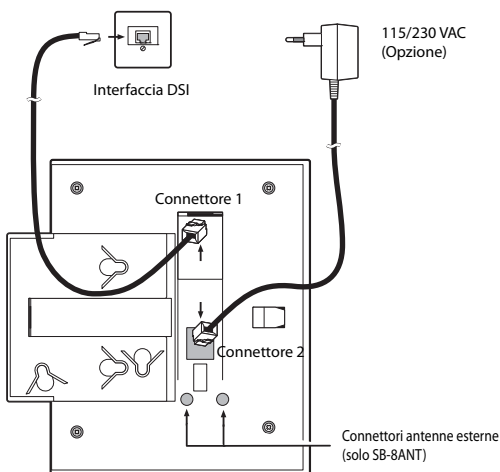
Fig. 69 Retro della base radio con punti di collegamento
