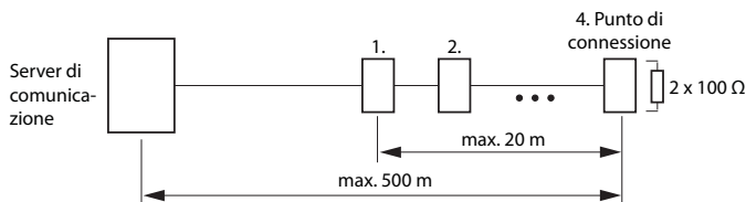
Fig. 48 Bus S, lungo
