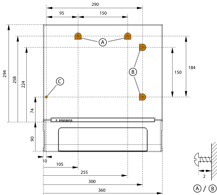
Fig. 14 Schema di foratura per montaggio a parete Mitel 415/430
