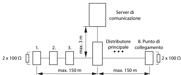
Fig. 47 Bus S corto, a V
