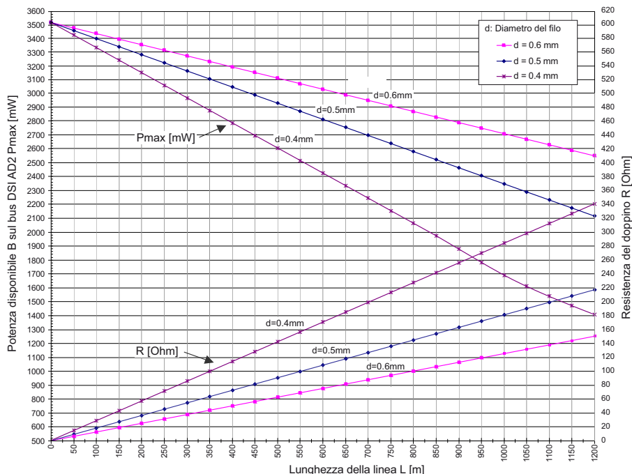
Fig. 44 Potenza disponibile B sul bus DSI AD2
