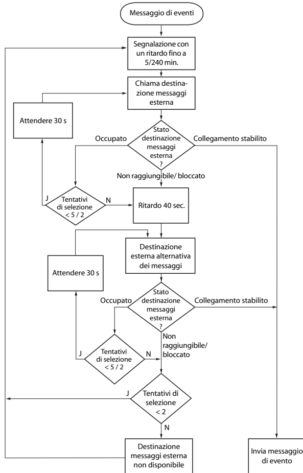
Fig. 81 Diagramma di flusso per la segnalazione di un messaggio di evento ad una destinazione esterna dei messaggi
