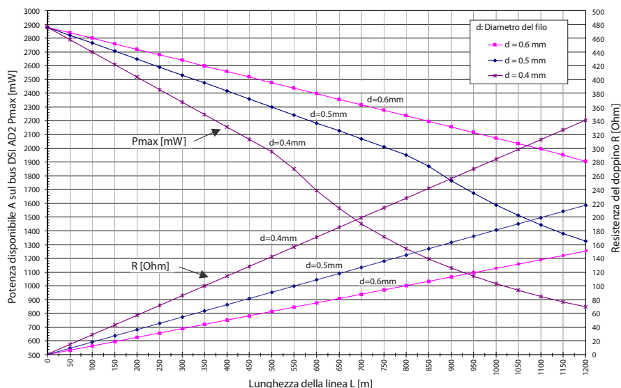
Fig. 43 Potenza disponibile A sul bus DSI AD2
