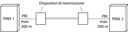
Fig. 38 Accesso primario, collegamento in rete con dispositivo di trasmissione
