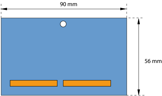
Fig. 85 Dimensioni del modulo di sistema (struttura D)
