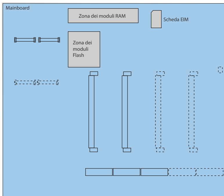
Fig. 75 Memorie sulla Mainboard Mitel 415/430
