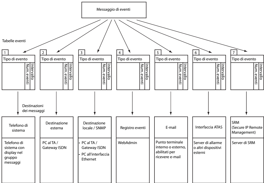
Fig. 80 Principio di distribuzione di un messaggio di evento
