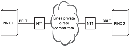
Fig. 34 Accesso base BRI-T, collegamento in rete con linea privata o rete commutata
