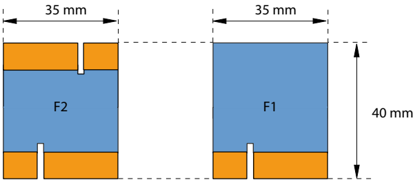
Fig. 86 Dimensioni adattatore wiring (struttura F)
