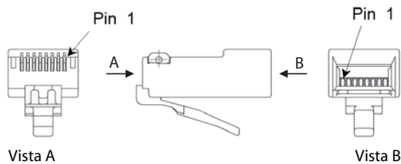
Fig. 27 Numerazione dei pin del connettore RJ45
