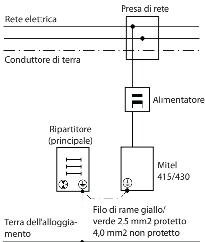
Fig. 20 Collegamento di terra del server di comunicazione in caso di collegamento indiretto e collegamento diretto
