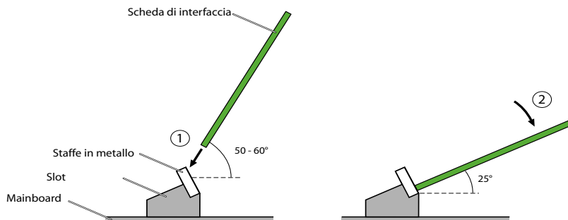
Fig. 23 Inserimento di una scheda di interfaccia
