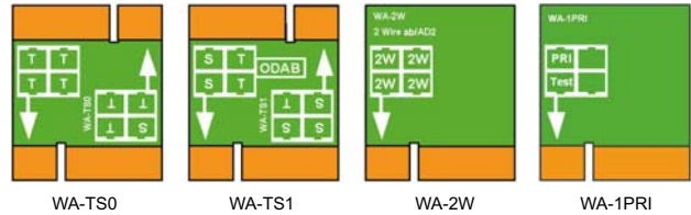
Fig. 10 Tipi di adattatori wiring
