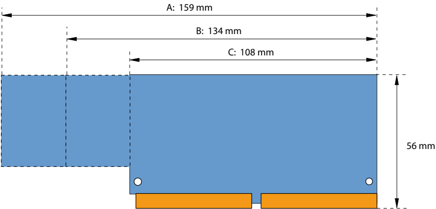
Fig. 82 Abmessungen Schnittstellenkarten (Bauform A, B, C)
