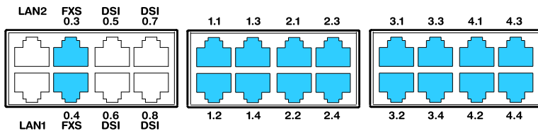
Fig. 52 Anschlussmöglichkeiten FXS-Endgeräteschnittstellen
