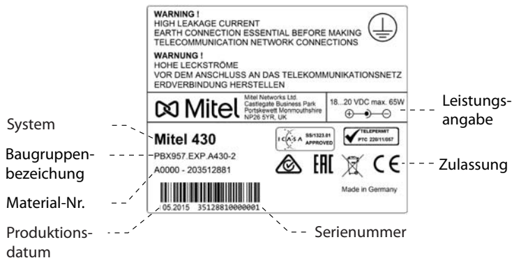
Fig. 80 Typenschild (Beispiel Kommunikationsserver Mitel 430)
