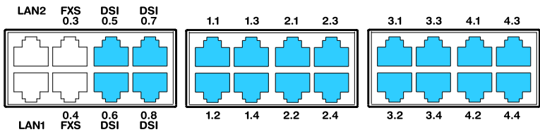
Fig. 41 Anschlussmöglichkeiten DSI-Endgeräteschnittstellen
