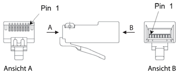
Fig. 27 Pin-Nummerierung RJ45-Stecker
