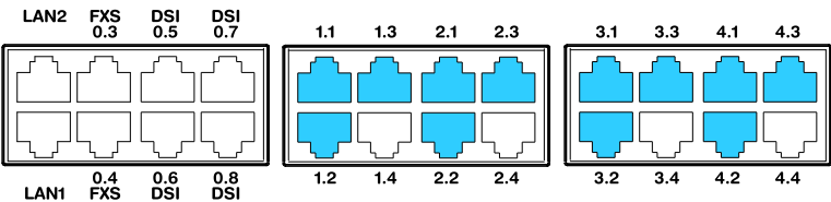
Fig. 45 Anschlussmöglichkeiten BRI-S-Endgeräteschnittstellen
