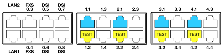
Fig. 35 Anschlussmöglichkeiten PRI-Netzchnittstellen
