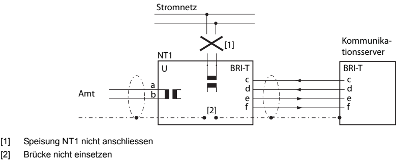
Fig. 32 Basisanschluss am NT1
