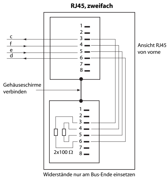
Fig. 51 Anschluss RJ45, Zweifachdose
