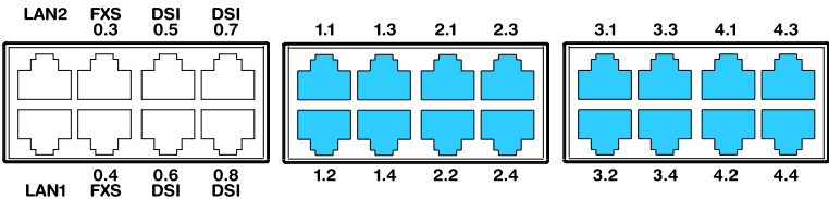
Fig. 31 Anschlussmöglichkeiten BRI-Netzschnittstellen
