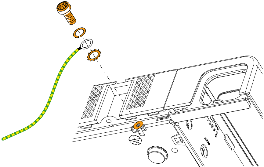
Fig. 19 Erdungsanschluss
