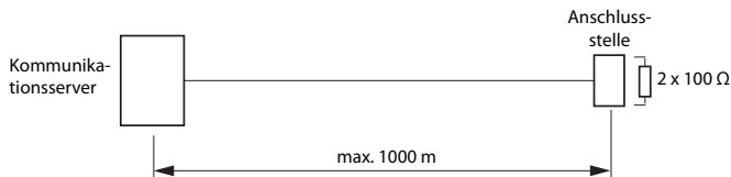
Fig. 49 S-Bus, Punkt-Punkt
