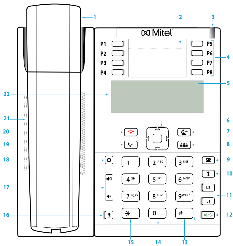
Mitel 6865 SIP
