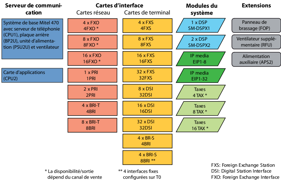
Fig. 5 Vue d'ensemble des possibilités d'extension
