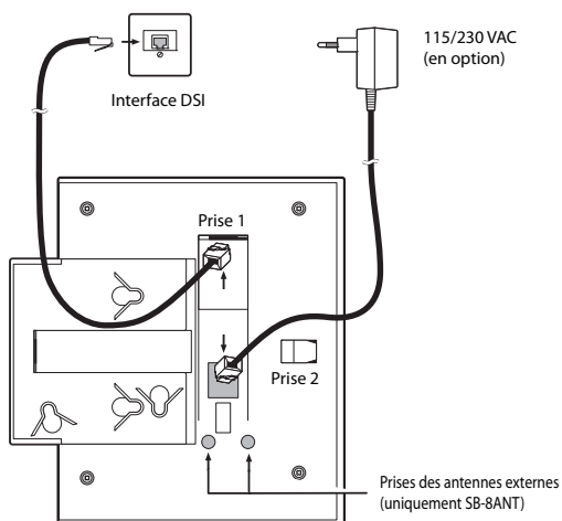
Fig. 72 Dos des unités radio avec points de raccordement
