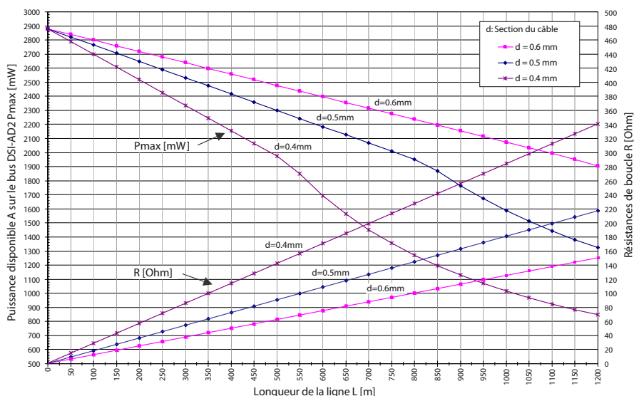
Fig. 47 Puissance disponible cas A sur le bus DSI-AD2
