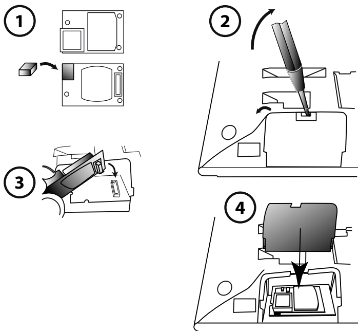
Fig. 69 Montage du module Bluetooth
