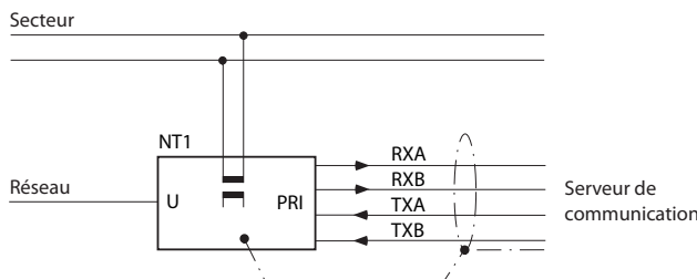
Fig. 40 Accès primaire RNIS T2 sur NT1
