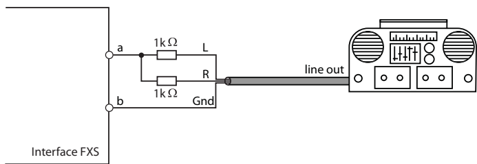
Fig. 61 Connexion pour le mode FXS : Source audio externe
