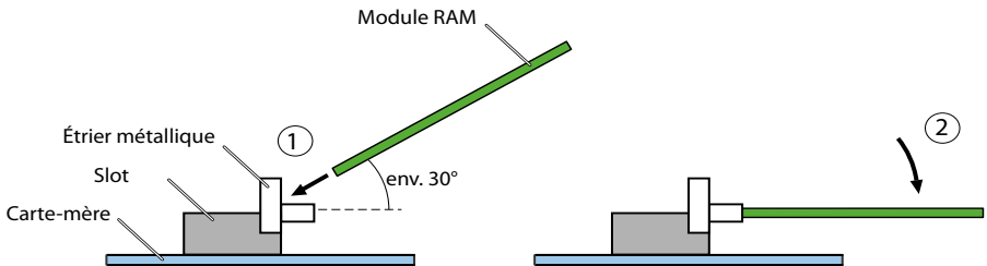
Fig. 79 Remplacer le module RAM
