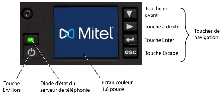
Fig. 82 Panneau d'affichage et de commande Mitel 470
