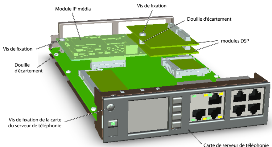
Fig. 27 Fonctions DSP fixes sur la carte de serveur de téléphonie
