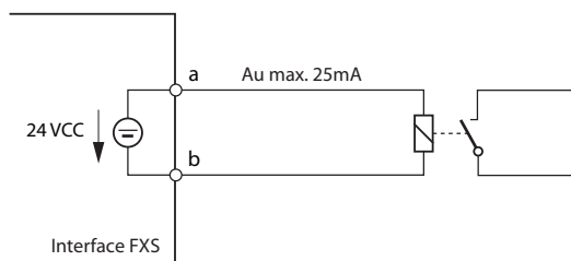
Fig. 62 Connexion pour le mode FXS : Sortie de commande
