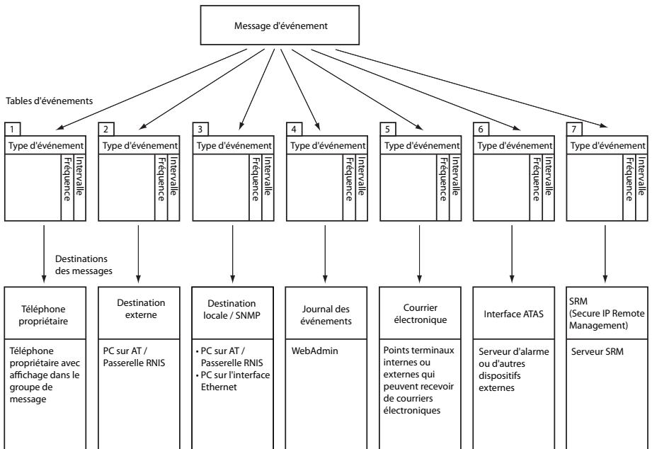
Fig. 85 Principe de distribution d'un message d'événement
