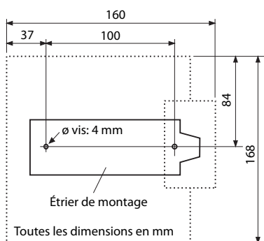
Fig. 70 Croquis pour le montage mural de l'étrier de montage
