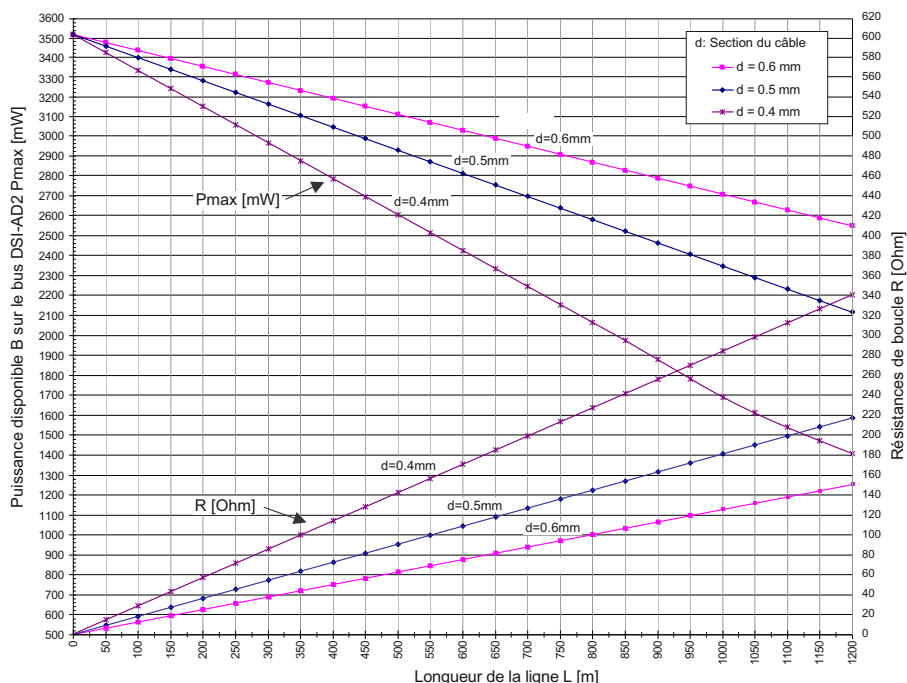
Fig. 48 Puissance disponible cas B sur le bus DSI-AD2
