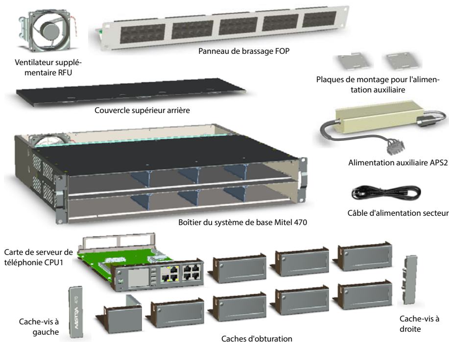
Fig. 17 Composants système avec options de montage
