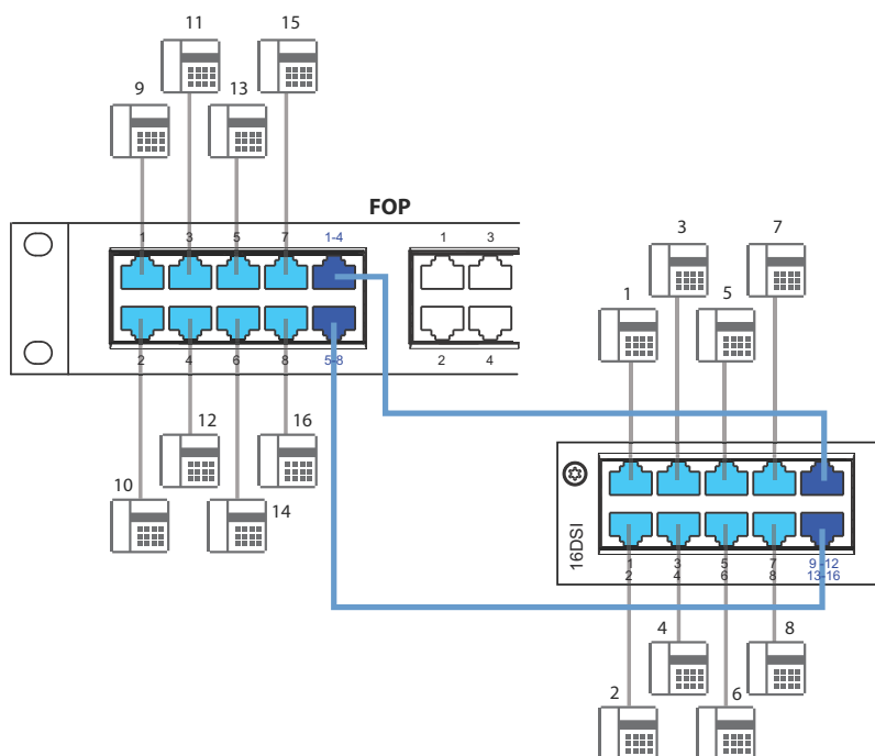
Fig. 66 Connexion de prises à quadruple affectation via le panneau de brassage FOP
