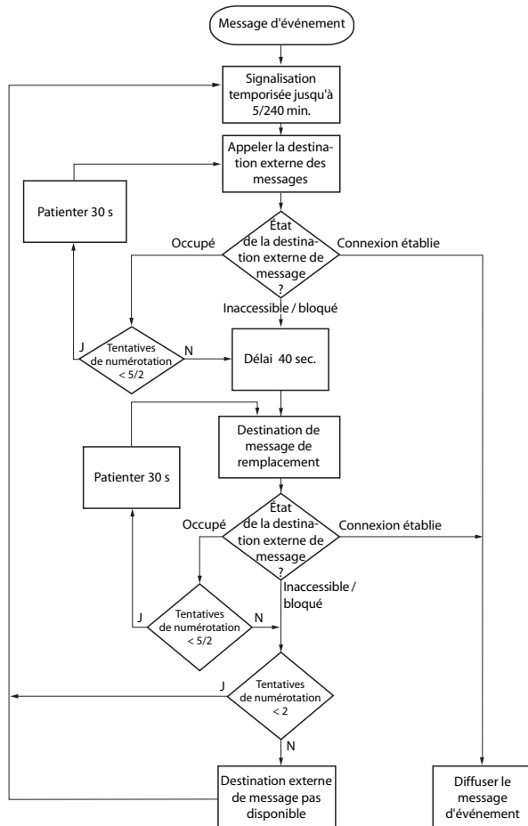
Fig. 86 Diagramme fonctionnel de la signalisation d'un message d'événement à une destination externe
