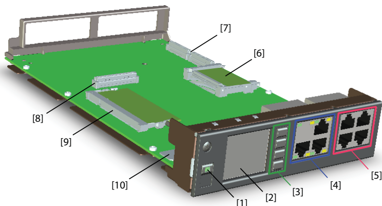
Fig. 9 Interfaces, éléments d'exploitation et d'affichage de la carte de serveur de téléphonie CPU1
