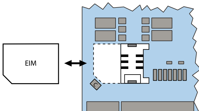
Fig. 80 Carte EIM
