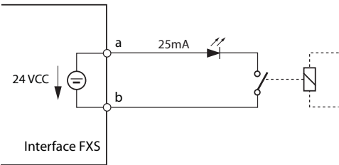
Fig. 63 Connexion pour le mode FXS : Entrée de commande
