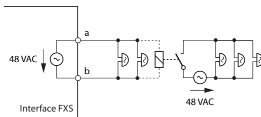
Fig. 64 Connexion pour le mode FXS : Sonnerie d'appel général
