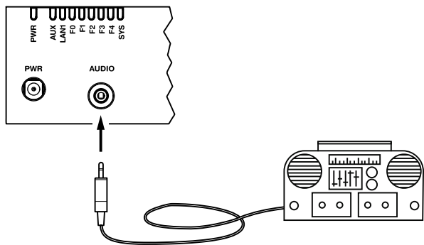
Fig. 62 Interfaccia audio
