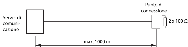
Fig. 49 Bus S, punto-punto
