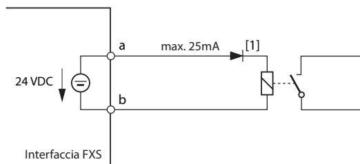
Fig. 55 Cablaggio per modo FXS: Uscita di comando
