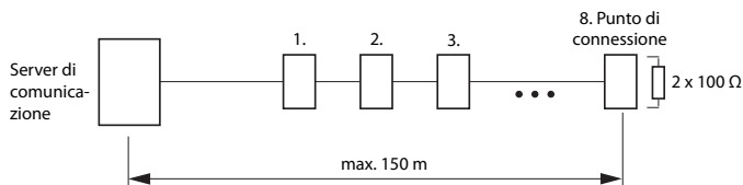
Fig. 46 Bus S corto
