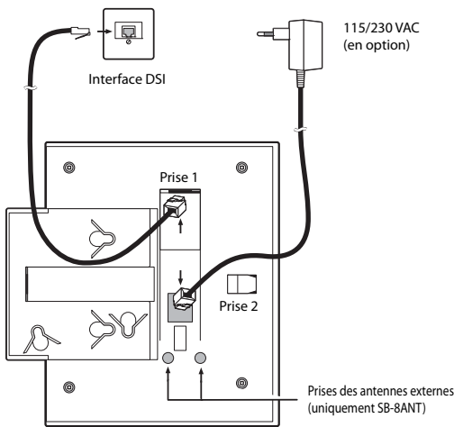
Fig. 67 Dos des unités radio avec points de raccordement
