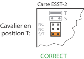
Fig. 24 Position du cavalier sur la carte ESST
