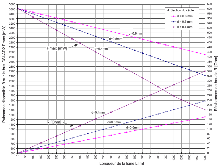
Fig. 44 Puissance disponible cas B sur le bus DSI-AD2
