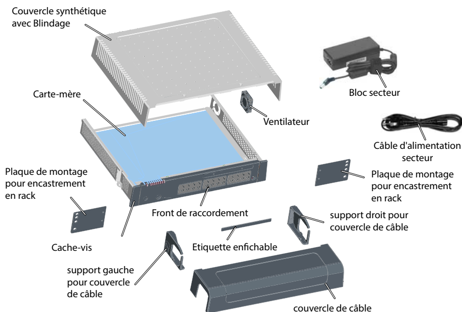
Fig. 11 Composants système avec options de montage
