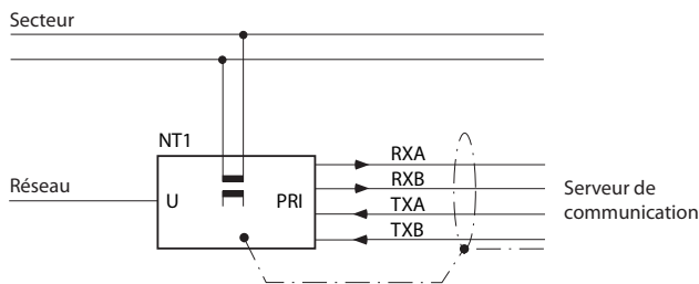
Fig. 36 Accès primaire RNIS T2 sur NT1
