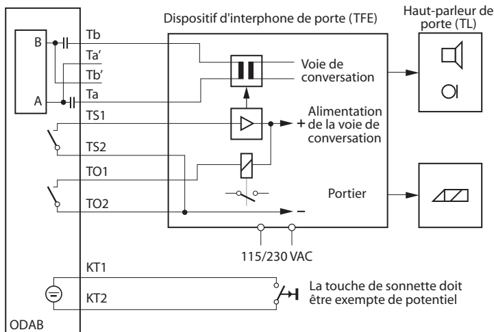
Fig. 60 Schéma de principe
