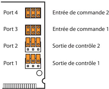
Fig. 61 Configuration du cavalier pour les sorties de commande et les entrées de commande
