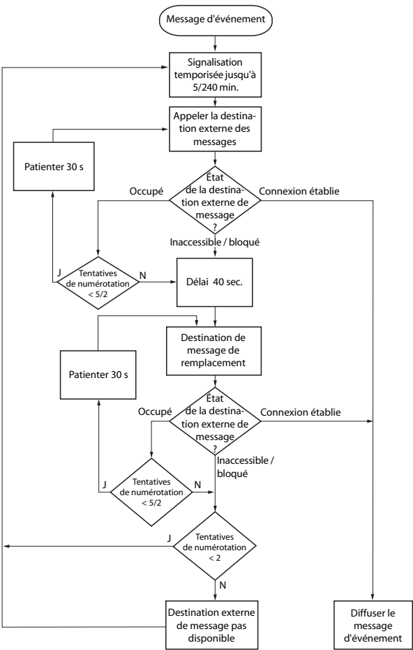
Fig. 79 Diagramme fonctionnel de la signalisation d'un message d'événement à une destination externe
