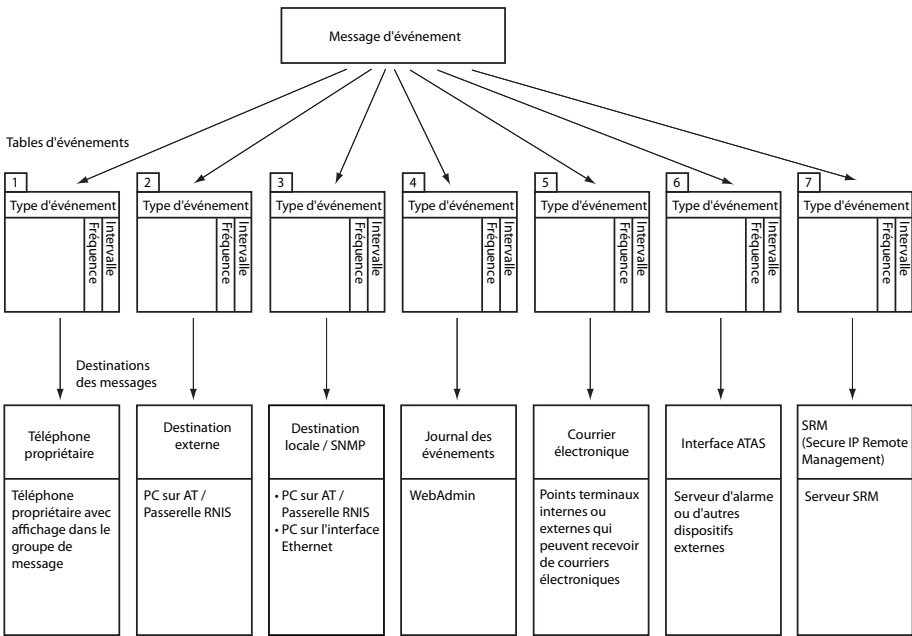
Fig. 78 Principe de distribution d'un message d'événement
