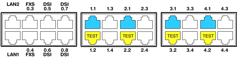
Fig. 35 Possibilités de raccordement des interfaces réseau T2
