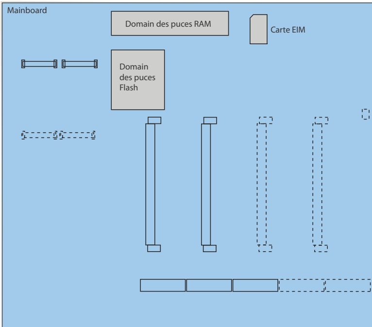
Fig. 73 Mémoire sur la carte-mère Mitel 415/430
