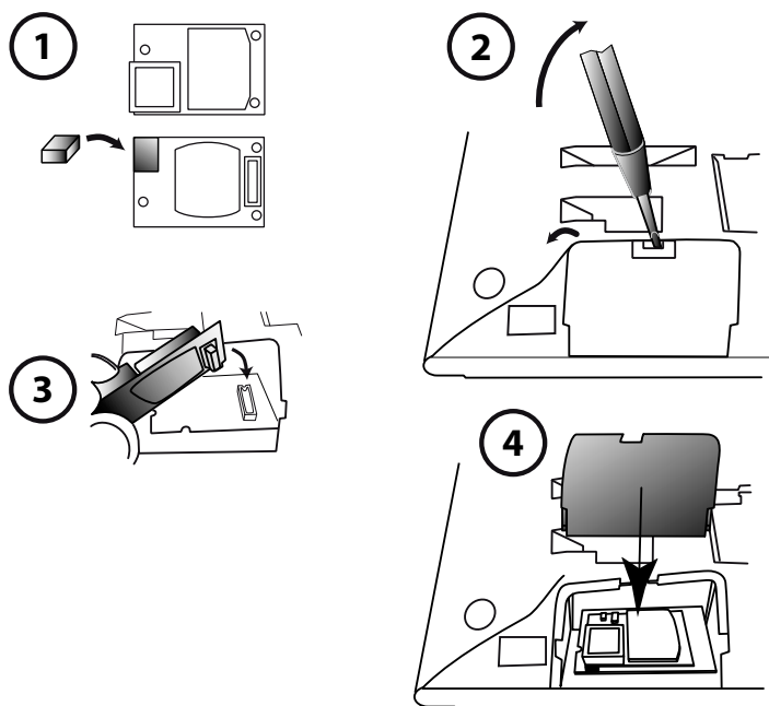
Fig. 64 Montage du module Bluetooth
