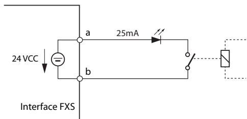
Fig. 56 Connexion pour le mode FXS : Entrée de commande
