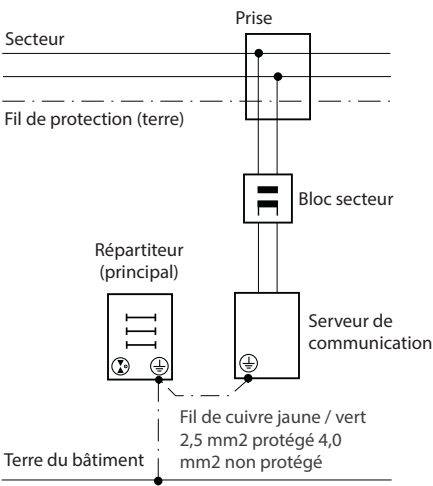
Fig. 20 Mise à terre du serveur de communication en cas de raccordement indirect et de raccordement direct
