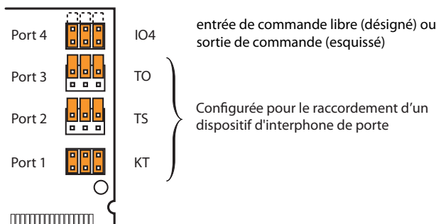
Fig. 59 Configuration du cavalier pour le raccordement d'un dispositif d'interphone de porte
