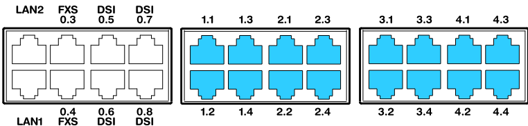
Fig. 31 Possibilités de raccordement des interfaces réseau S0/T0
