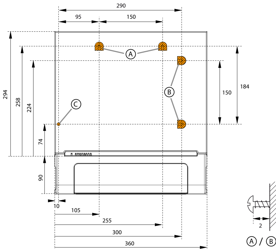
Fig. 14 Plan de perçage pour montage mural de l'
