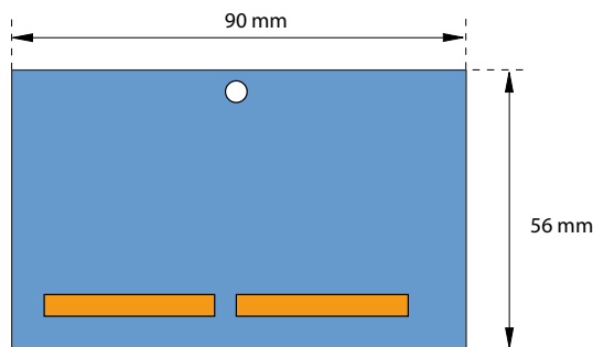
Fig. 83 Dimension des modules système (forme de construction D)
