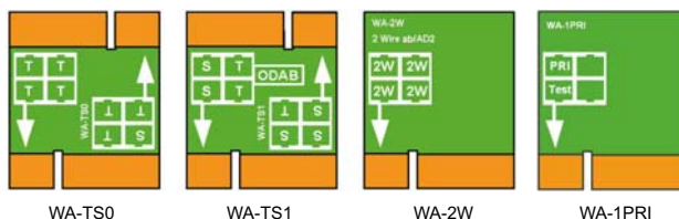
Fig. 10 Types d'adaptateur de câblage
