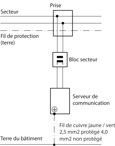
Fig. 20 Mise à terre du serveur de communication en cas de raccordement indirect et de raccordement direct
