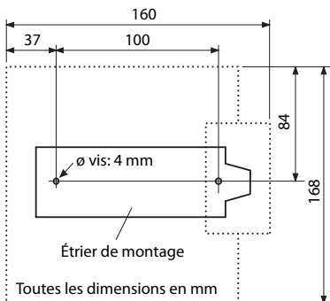
Fig. 65 Croquis pour le montage mural de l'étrier de montage
