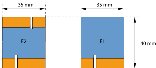
Fig. 84 Dimensions de l'adaptateur de câblage (forme de construction F)
