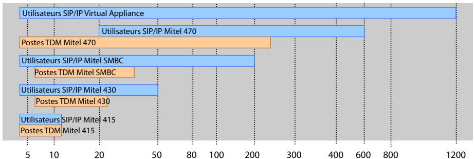
Fig. 3 La capacité d'extension max. pour les utilisateurs disposant des téléphones SIP/IP et des postes TDM (FXS, DSI, BRI-S)
