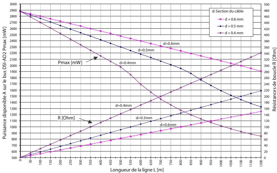
Fig. 43 Puissance disponible cas A sur le bus DSI-AD2
