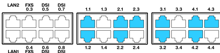
Fig. 58 Interfaces de la carte optionnelle ODAB
