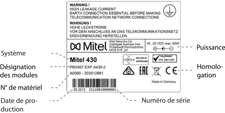
Fig. 80 Plaquette signalétique (exemple du serveur de communication Mitel 430)
