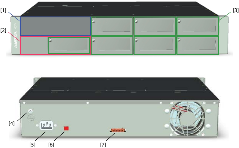
Fig. 8 Posizione delle interfacce del sistema base
