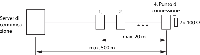
Fig. 52 Bus S, lungo
