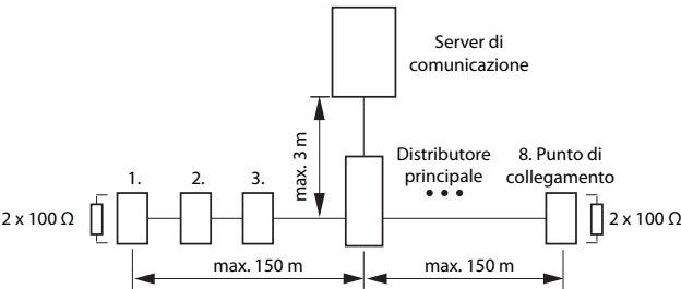
Fig. 51 Bus S corto, a V
