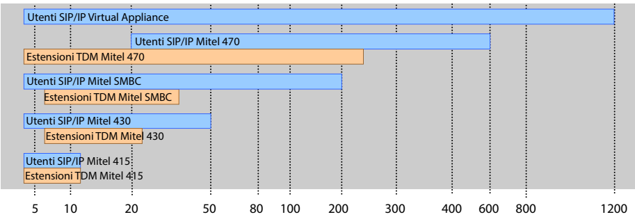
Fig. 2 Capacità di espansione massima per utenti con telefoni SIP/IP ed estensioni TDM (FXS, DSI, BRI-S)
