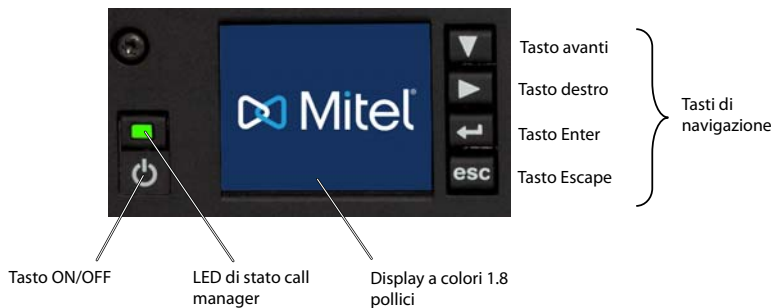
Fig. 82 Pannello di visualizzazione e di comando Mitel 470
