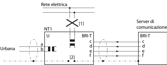
Fig. 36 Accesso base su NT1
