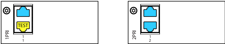
Fig. 39 Possibilità di collegamento delle interfacce di rete PRI
