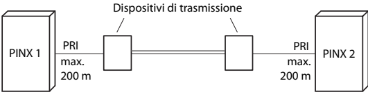
Fig. 42 Accesso primario, collegamento in rete con dispositivo di trasmissione
