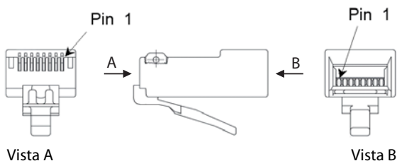
Fig. 31 Numerazione dei pin del connettore RJ45
