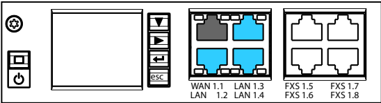
Fig. 67 Possibilità di collegamento delle interfacce Ethernet
