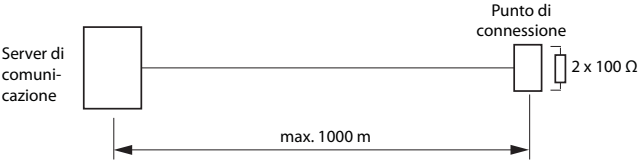
Fig. 53 Bus S, punto-punto
