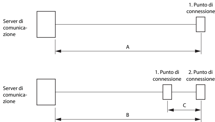
Fig. 46 Bus DSI-AD2
