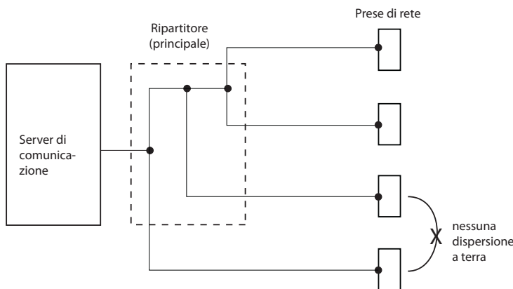
Fig. 23 Principio della struttura ad albero
