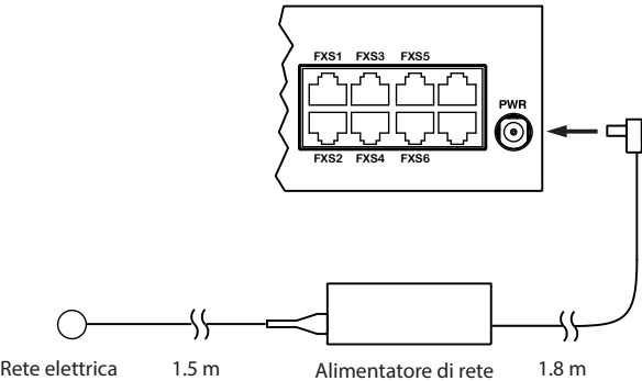
Fig. 21 Alimentazione del server di comunicazione dalla rete elettrica
