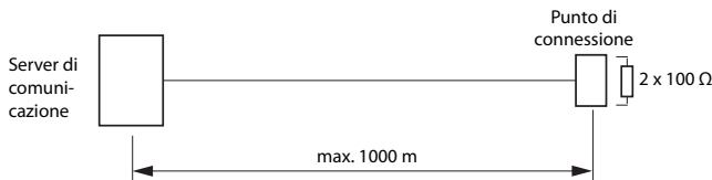
Fig. 48 Bus S, punto-punto
