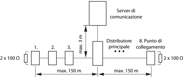
Fig. 46 Bus S corto, a V
