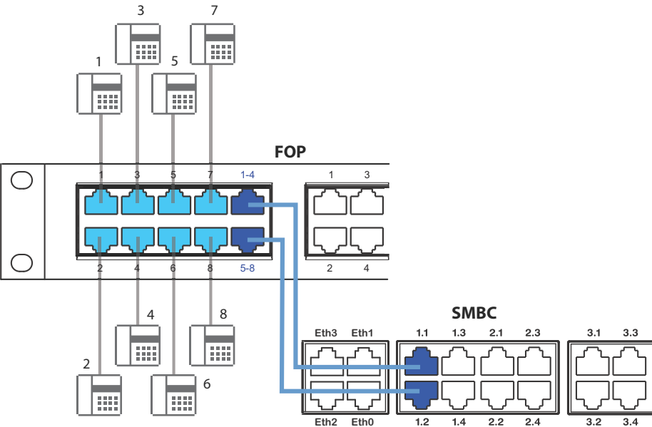
Fig. 58 Cablaggio di connettori a quattro poli tramite quadro distributore FOP
