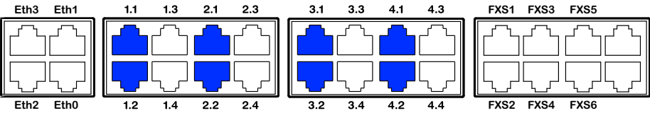
Fig. 40 Possibilità di collegamento delle interfacce di terminale DSI su connettori RJ45 ad un solo polo
