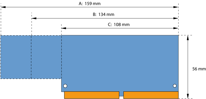
Fig. 80 Dimensioni schede di interfaccia (struttura A, B, C)
