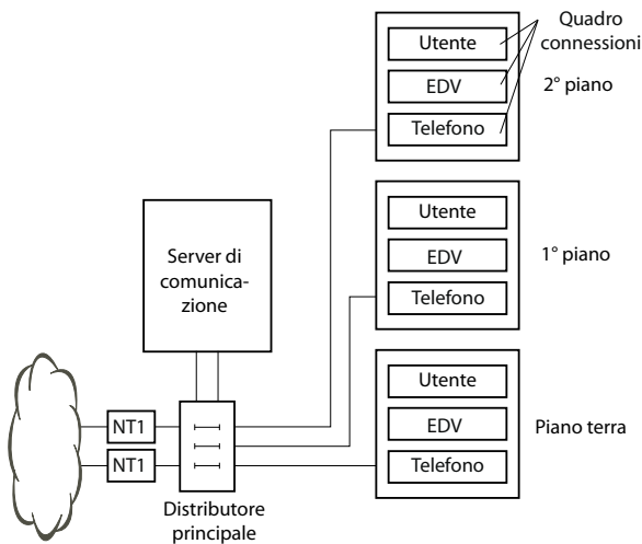
Fig. 26 Collegamento al CS attraverso il distributore principale (esempio)
