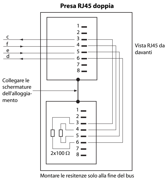
Fig. 50 Collegamento RJ45, presa doppia
