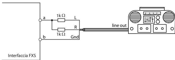
Fig. 54 Cablaggio per modo FXS: Origine audio esterna
