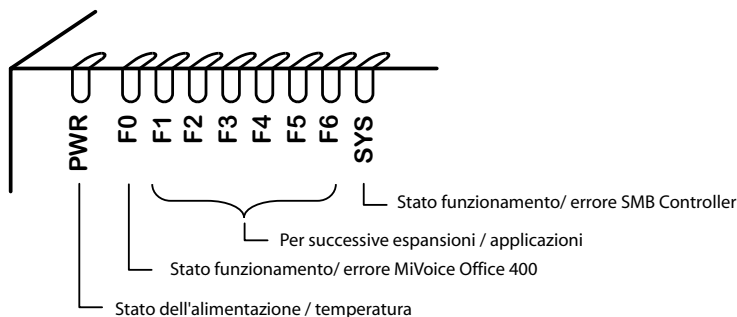
Fig. 74 Campi di segnalazione LED
