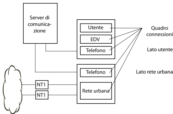
Fig. 27 Collegamento al CS attraverso il Wiring Center (esempio)
