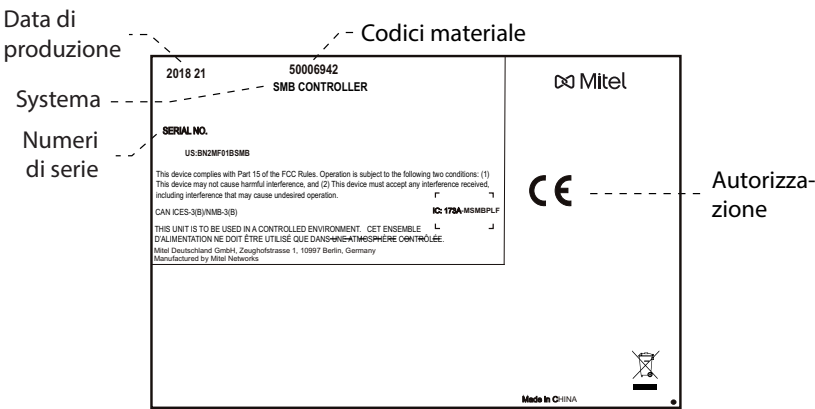
Fig. 78 Targhetta di identificazione Mitel SMBC server di comunicazione
