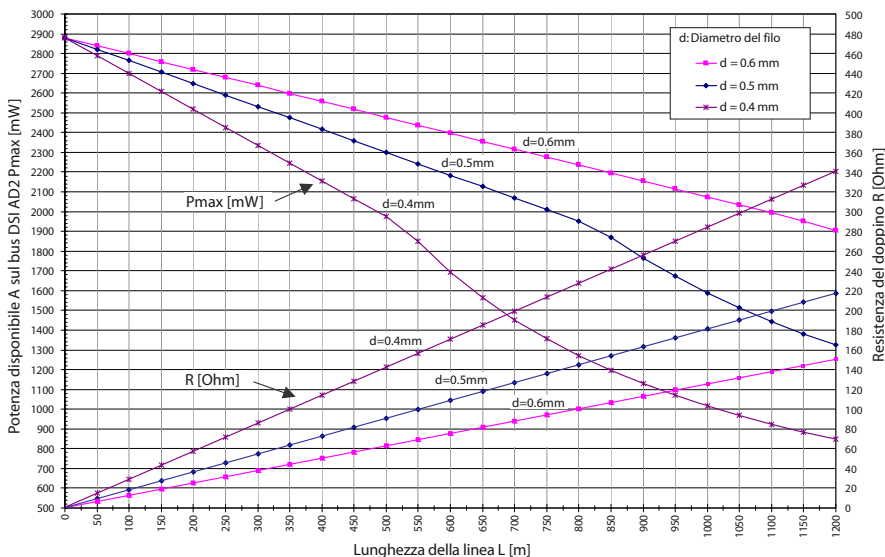
Fig. 42 Potenza disponibile caso A sul bus DSI AD2
