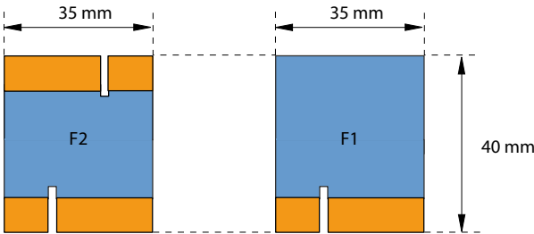
Fig. 82 Dimensioni adattatore wiring (struttura F)
