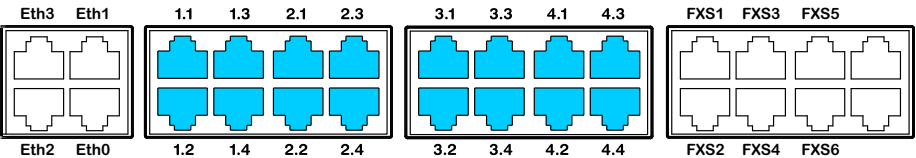
Fig. 38 Possibilità di collegamento delle interfacce di rete FXO
