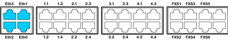
Fig. 59 Possibilità di collegamento delle interfacce Ethernet
