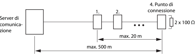
Fig. 47 Bus S, lungo
