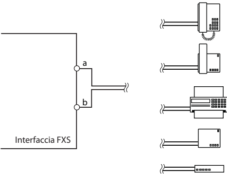
Fig. 52 Cablaggio per modo FXS: Telefono/Fax
