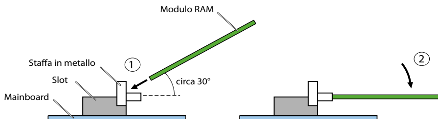
Fig. 72 Sostituzione del modulo DSP
