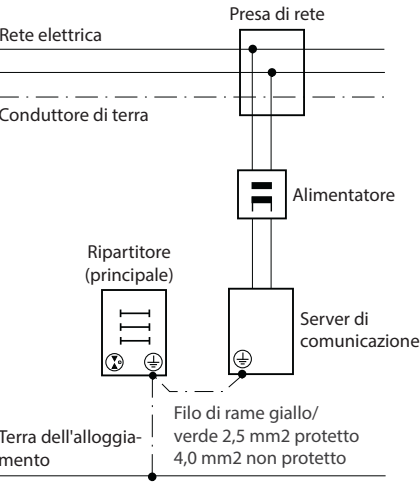
Fig. 19 Collegamento di terra del server di comunicazione in caso di collegamento indiretto e collegamento diretto
