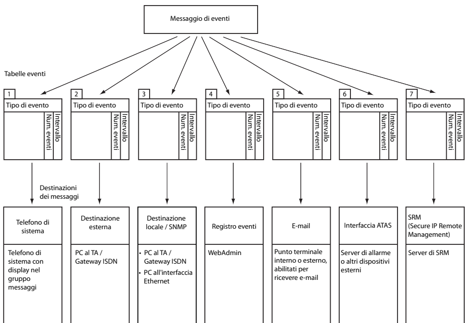
Fig. 76 Principio di distribuzione di un messaggio di evento
