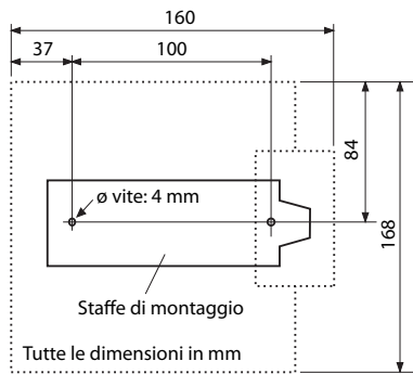
Fig. 62 Disegno e quote per il montaggio a parete della staffa
