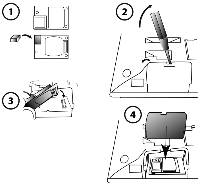
Fig. 61 Montaggio del modulo Bluetooth
