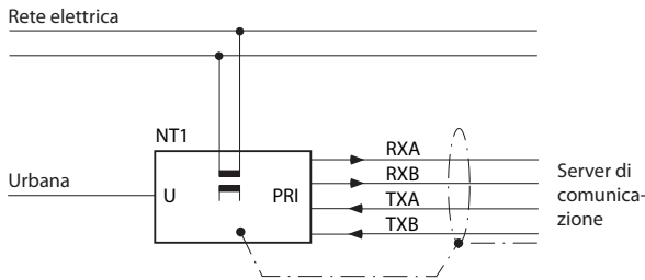
Fig. 34 Accesso primario PRI su NT1
