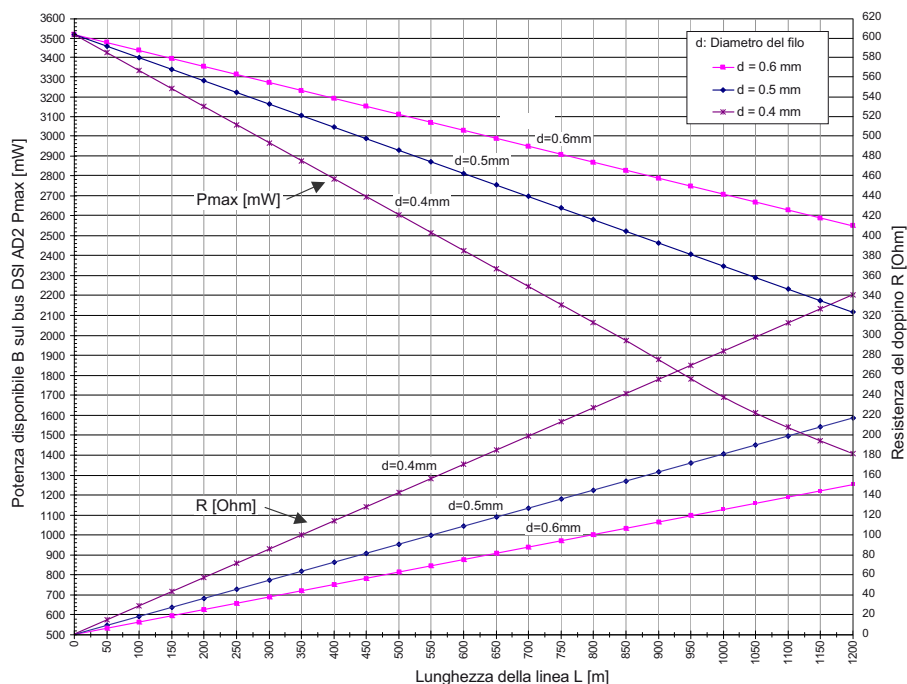
Fig. 43 Potenza disponibile caso B sul bus DSI AD2
