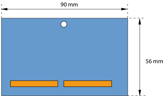
Fig. 81 Dimensioni del modulo di sistema (struttura D)
