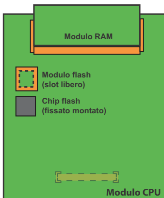
Fig. 71 Memorie sul modulo CPU del SMB Controller
