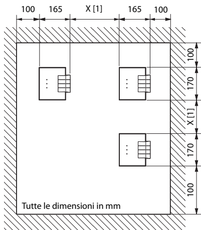
Fig. 62 Disegno e quote per il montaggio a parete della staffa
