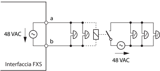
Fig. 56 Cablaggio per modo FXS: Suoneria centralizzata
