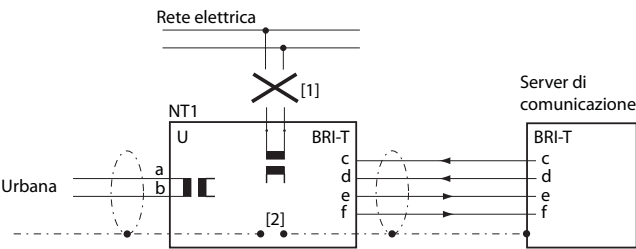
Fig. 30 Accesso base su NT1
