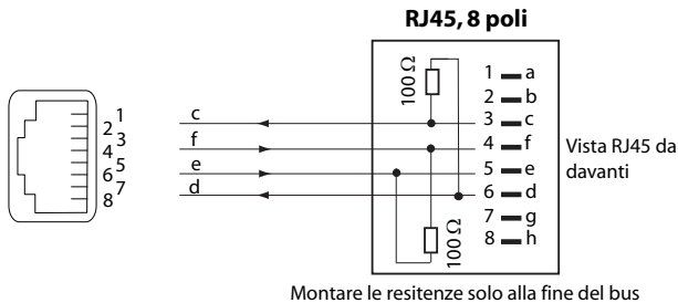
Fig. 49 Collegamento RJ45, presa semplice
