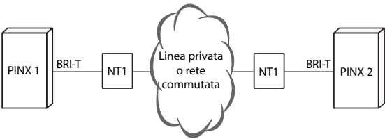
Fig. 32 Accesso base BRI-T, collegamento in rete con linea privata o rete commutata
