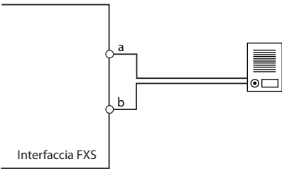
Fig. 53 Cablaggio per modo FXS: Collegamento 2 fili
