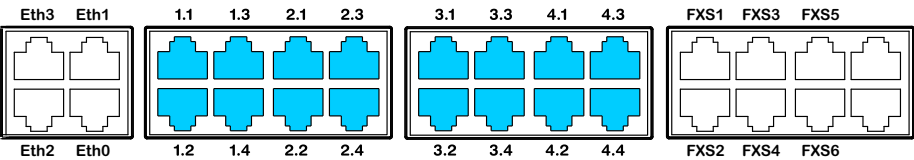
Fig. 39 Possibilità di collegamento delle interfacce di terminale DSI su connettori RJ45 ad un solo polo
