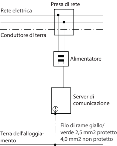
Fig. 19 Collegamento di terra del server di comunicazione in caso di collegamento indiretto e collegamento diretto
