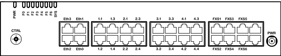
Fig. 28 Interfacce del pannello frontale con denominazione delle porte (Mitel SMBC)
