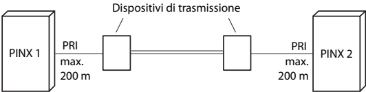
Fig. 36 Accesso primario, collegamento in rete con dispositivo di trasmissione
