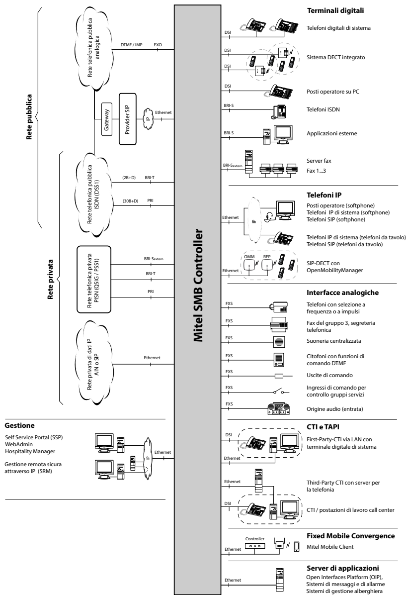
Fig. 5 Schema delle interfacce con i terminali possibili
