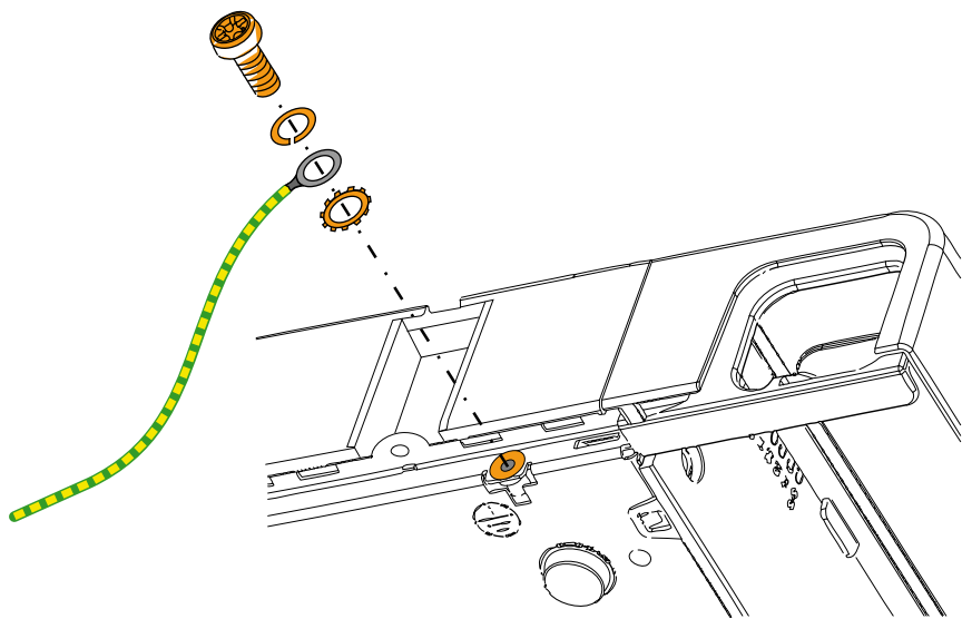
Fig. 18 Collegamento di terra
