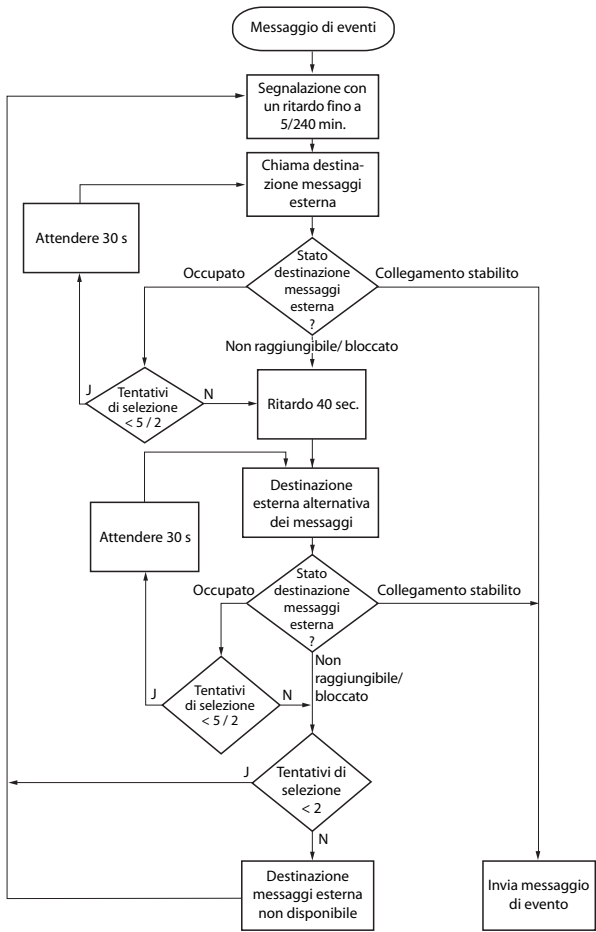
Fig. 77 Diagramma di flusso per la segnalazione di un messaggio di evento ad una destinazione esterna dei messaggi
