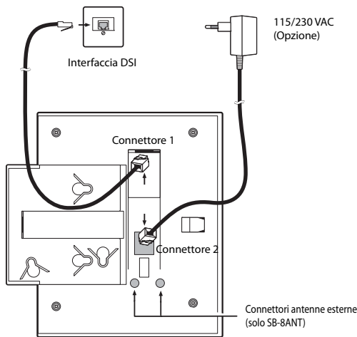
Fig. 64 Retro della base radio con punti di collegamento
