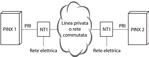
Fig. 37 Accesso primario PRI, collegamento in rete con linea privata o rete commutata
