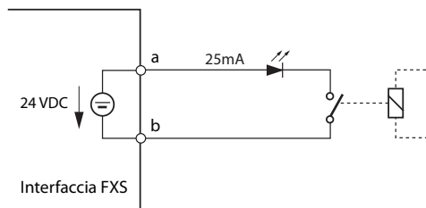
Fig. 55 Cablaggio per modo FXS: Ingresso di comando
