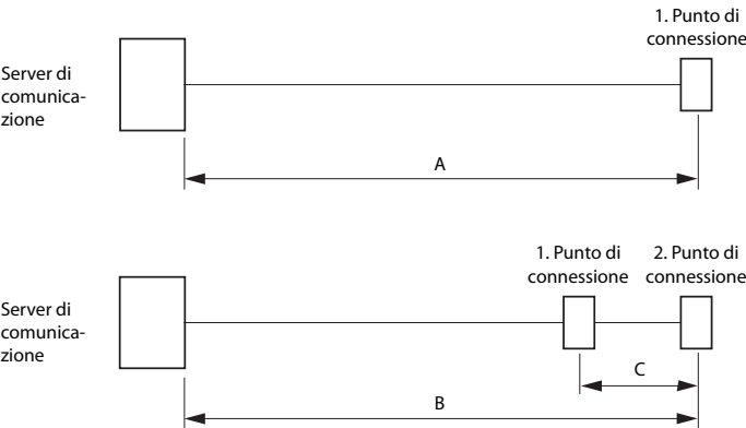
Fig. 41 Bus DSI-AD2
