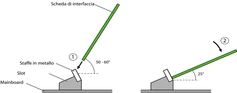
Fig. 22 Inserimento di una scheda di interfaccia
