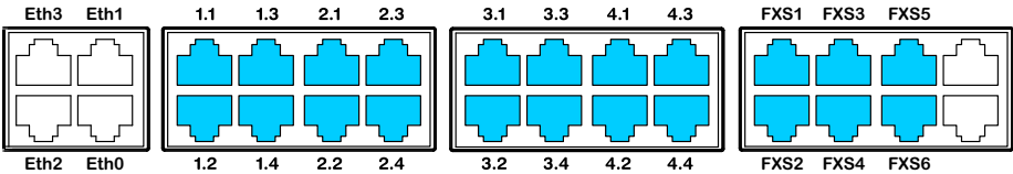
Fig. 51 Possibilità di collegamento delle interfacce di terminale FXS
