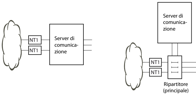
Fig. 23 Collegamento diretto (sinistra) e collegamento indiretto (destra)
