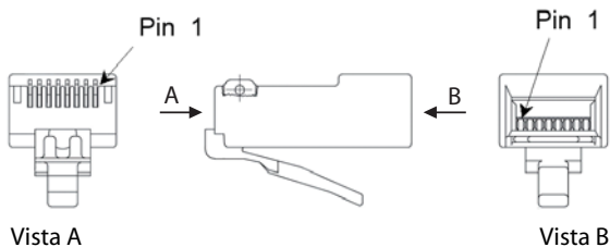
Fig. 25 Numerazione dei pin del connettore RJ45
