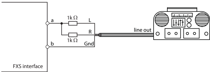
Fig. 61 Aansluiting voor FXS modus: Externe audiobron
