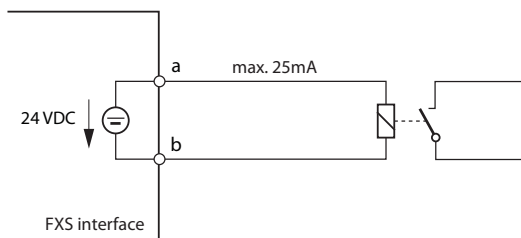
Fig. 62 Aansluiting voor FXS modus: Controle output
