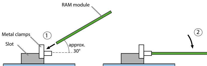
Fig. 79 Verwisselen van de RAM-module
