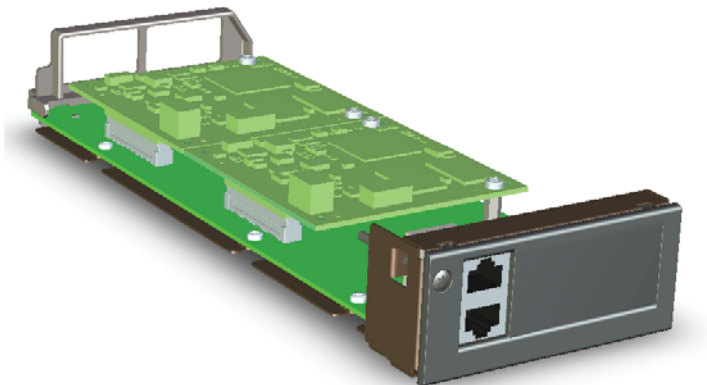
Fig. 15 Voorbeeld van een interfacekaart (2PRI met 2 IP mediamodules geïnstalleerd)
