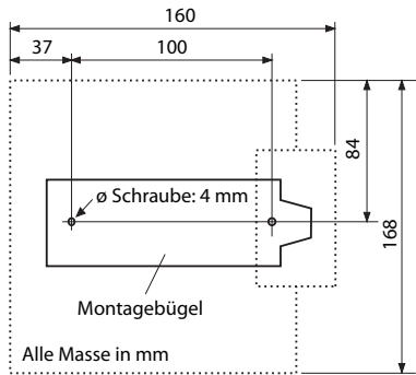
Fig. 62 Massbild für Wandmontage des Montagebügels
