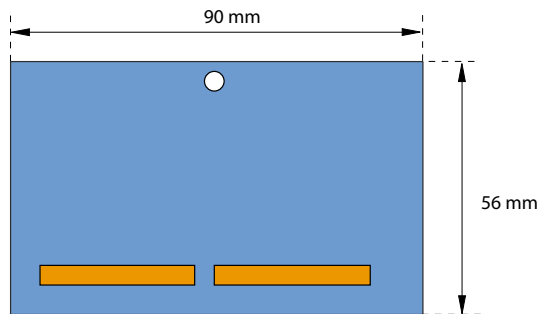
Fig. 81 Abmessungen Systemmodul (Bauform D)
