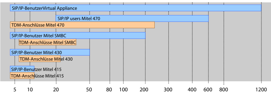
Fig. 3 Maximale Erweiterungskapazität für Benutzer mit SIP/IP-Telefonen und TDM-Erweiterungen (FXS, DSI, BRI-S)
