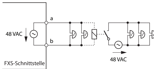
Fig. 56 Besaltung für FXS-Modus: Zentralwecker
