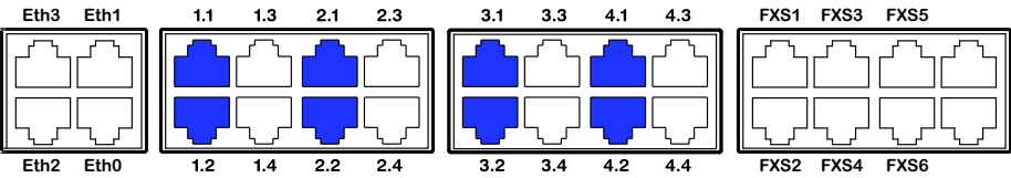
Fig. 40 Anschlussmöglichkeiten für DSI-Klemmschnittstellen auf mehrfach belegten RJ45-Buchsen
