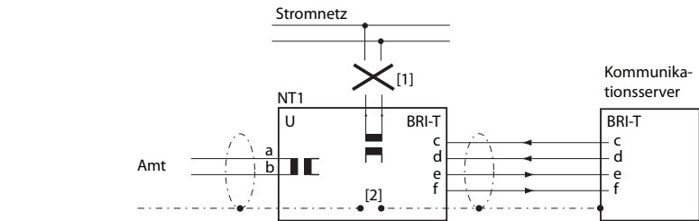
Fig. 30 Basisanschluss am NT1
