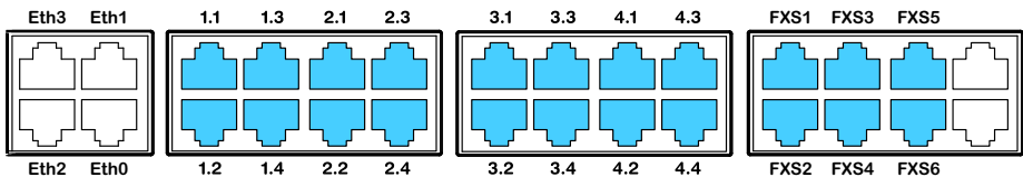
Fig. 51 Anschlussmöglichkeiten FXS-Endgeräteschnittstellen
