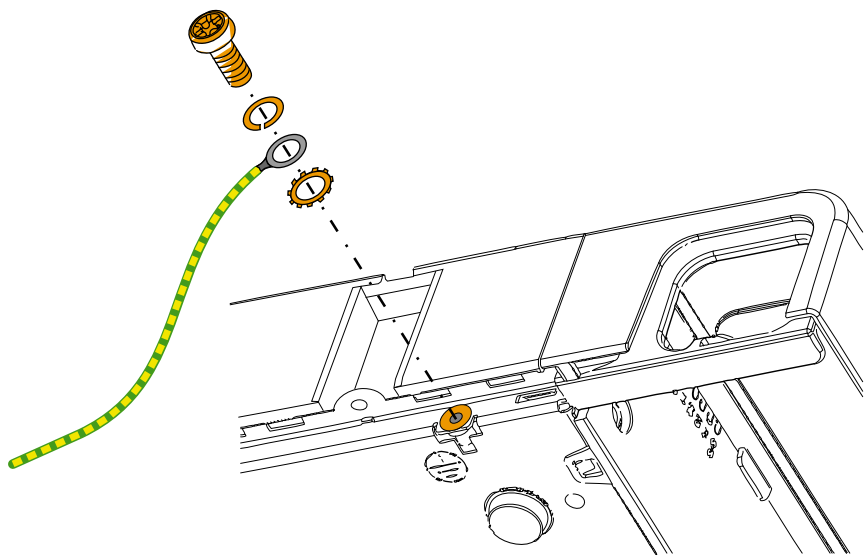
Fig. 18 Erdungsanschluss
