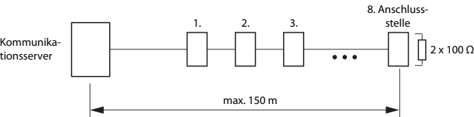
Fig. 45 S-Bus kurz
