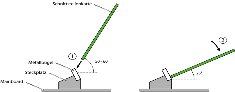
Fig. 22 Schnittstellenkarte bestücken
