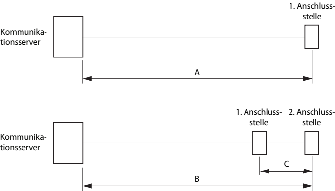
Fig. 41 DSI-AD2-Bus
