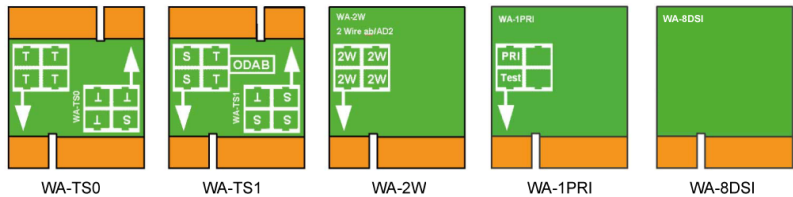
Fig. 10 Verdrahtungsadapter-Typen
