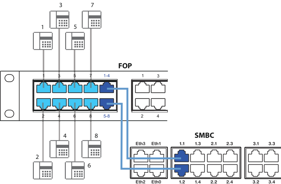
Fig. 58 Beschaltung von vierfach belegten Buchsen via Verteilpanel FOP
