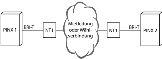
Fig. 32 Basisanschluss BRI-T Vernetzung mit Mietleitung oder Wählverbindung
