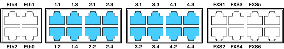
Fig. 29 Anschlussmöglichkeiten BRI-Netzschnittstellen
