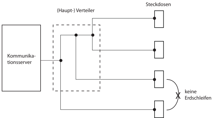
Fig. 20 Baumordnungsprinzip
