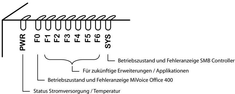
Fig. 74 LED-Anzeigefeld
