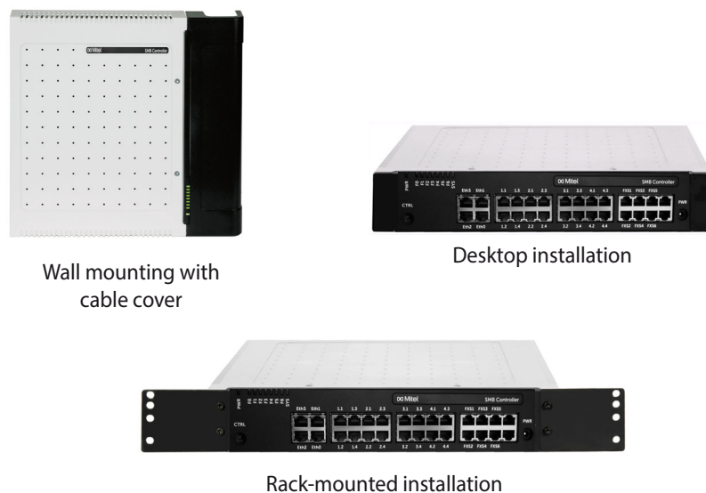
Fig. 2 Installatieversies
