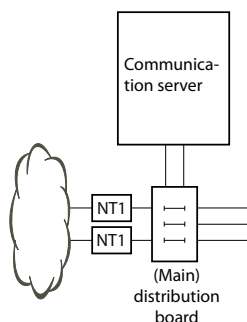
Fig. 24 Aansluiting via het hoofdverdelerbord
