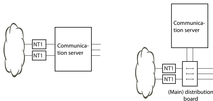
Fig. 23 Directe bekabeling (links) en indirecte bekabeling (rechts)
