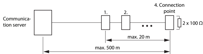
Fig. 47 S-bus, lang
