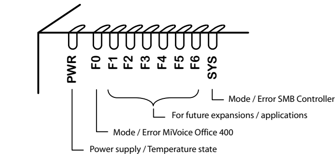
Fig. 74 LED-display
