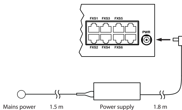
Fig. 21 De communicatieserver voeden vanuit het stroomnet
