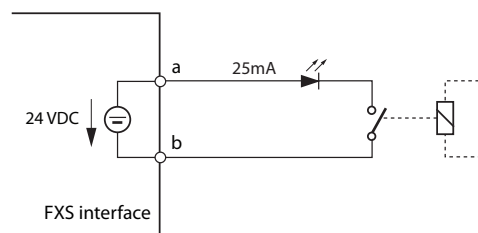
Fig. 55 Aansluiting voor FXS modus: Controle input
