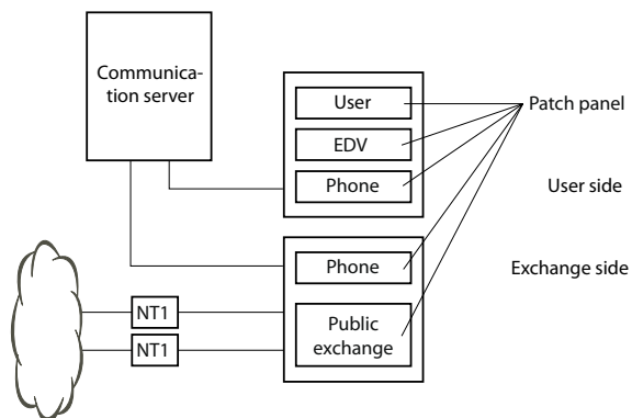
Fig. 27 Aansluiten op een UBC via een bedradingscentrum (voorbeeld)
