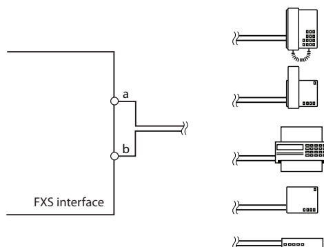
Fig. 52 Aansluiting voor FXS modus: Telefoon/fax
