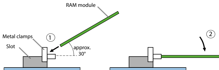
Fig. 72 Verwisselen van de RAM-module
