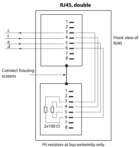
Fig. 50 RJ45 aansluiting, dubbel aansluitpunt
