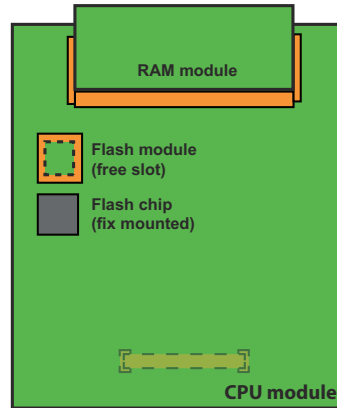
Fig. 71 Geheugens op de CPU-module van de SMB Controller
