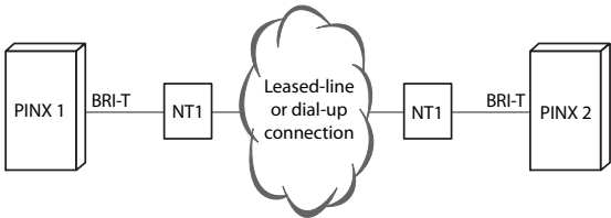
Fig. 32 Basissnelheid-interface BRI-T, in een netwerk met gehuurde lijnen of kiesverbinding
