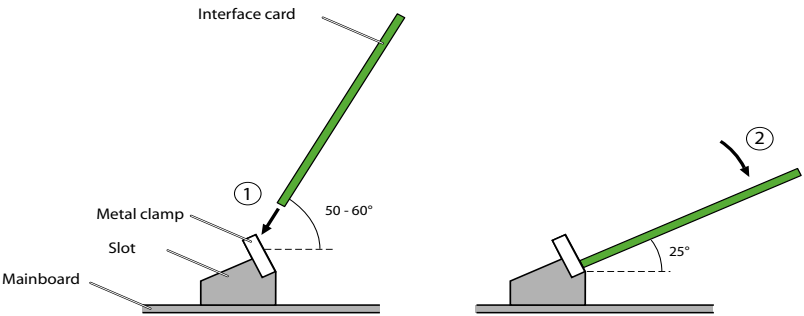
Fig. 22 Installeren van een interfacekaart
