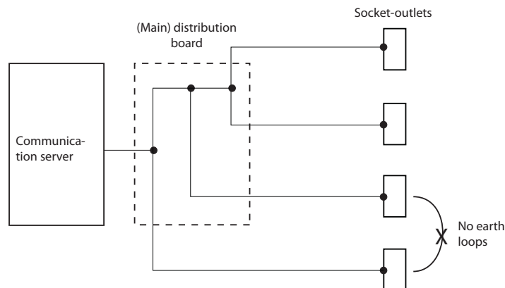
Fig. 20 Boomstructuurprincipe
