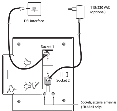
Fig. 64 Onderkant van de radio-units met aansluitpunten
