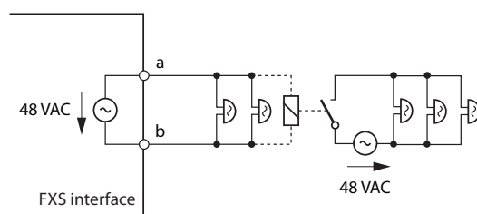
Fig. 56 Aansluiting voor FXS modus: Algemene beltoon
