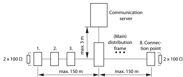
Fig. 46 S-bus, kort, V-vormig
