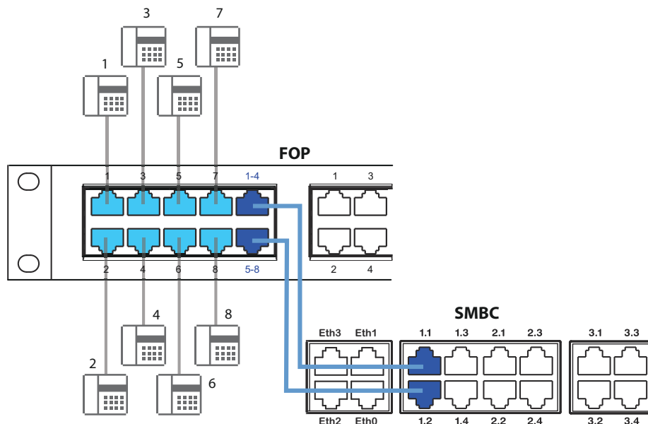
Fig. 58 Aansluiting van viervoudig toegewezen aansluitpunten via FOP connectorstrip
