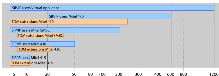
Fig. 3 Max. uitbreidingscapaciteit voor gebruikers met SIP/IP-telefoons en TDM-uitbreidingen (FXS, DSL, BRI-S)
