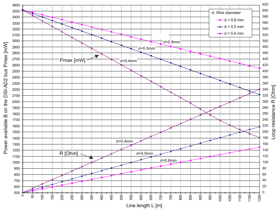
Fig. 43 Beschikbaar vermogen geval B op de DSI-AD2 bus
