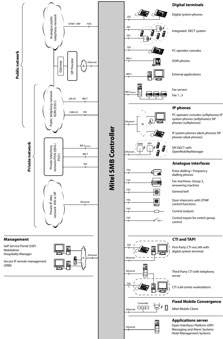
Fig. 5 Overzicht van interfaces met mogelijke eindstationapparatuur
