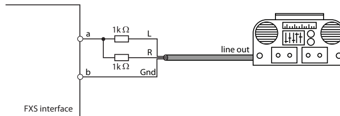
Fig. 54 Aansluiting voor FXS modus: Externe audiobron
