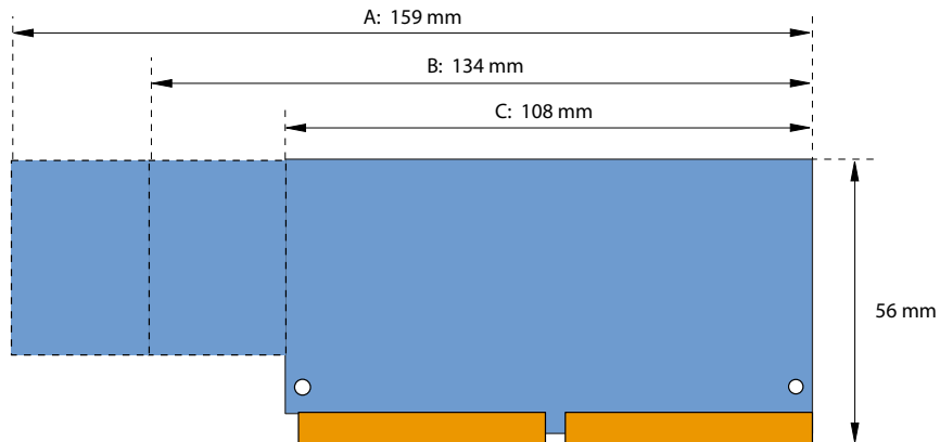
Fig. 80 Afmetingen van interfacekaarten (ontwerp A, B, C)
