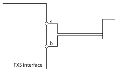
Fig. 53 Aansluiting voor FXS modus: 2-draads deur
