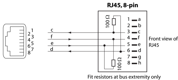
Fig. 49 RJ45 aansluiting, enkel aansluitpunt
