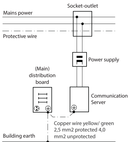
Fig. 19 Aarding van de communicatieserver in het geval van een indirecte bekabeling en een directe bekabeling
