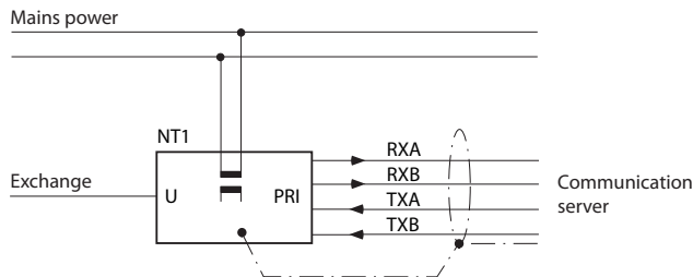
Fig. 34 PRI basissnelheid-interface op NT1
