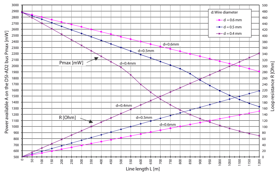
Fig. 42 Beschikbaar vermogen geval A op de DSI-AD2 bus
