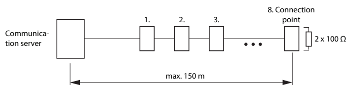
Fig. 45 S-bus, kort
