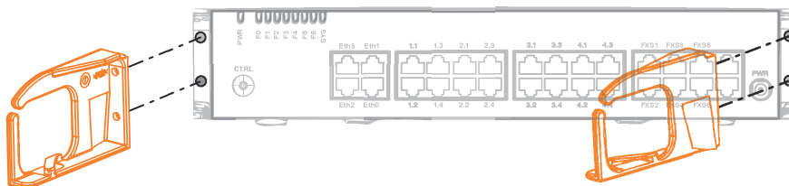
Fig. 17 Installeren van de beugels voor de kabelafdekking
