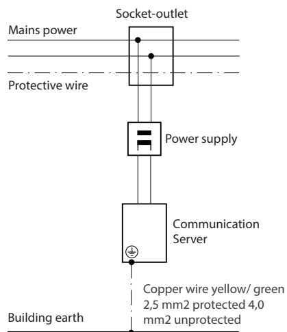
Fig. 19 Aarding van de communicatieserver in het geval van een indirecte bekabeling en een directe bekabeling
