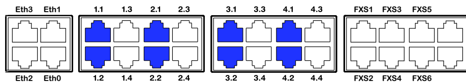
Fig. 40 Aansluitmogelijkheden voor DSI eindstationinterfaces op meervoudig toegewezen RJ45 aansluitpunten
