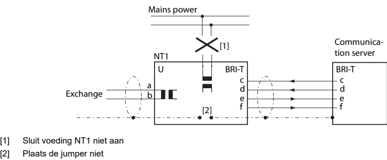
Fig. 30 Basale toegang op NT1
