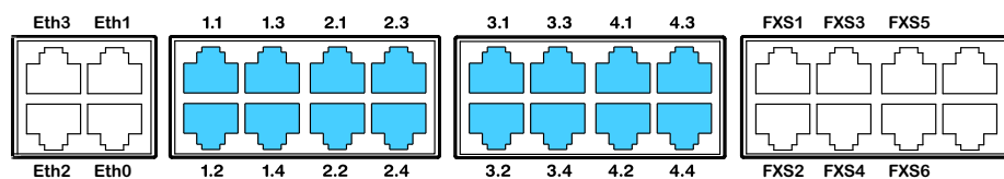
Fig. 39 Aansluitmogelijkheden voor DSI eindstationinterfaces op afzonderlijk toegewezen RJ45 aansluitpunten
