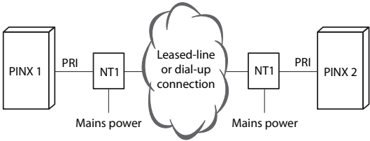
Fig. 37 Toegang met primaire snelheid PRI, in een netwerk met gehuurde lijnen of kiesverbinding
