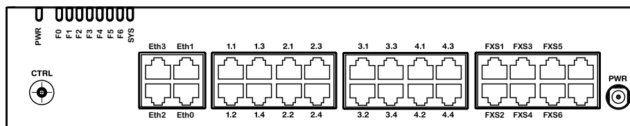
Fig. 28 Interfaces op het voorpaneel met poort aanduiding (Mitel SMBC)
