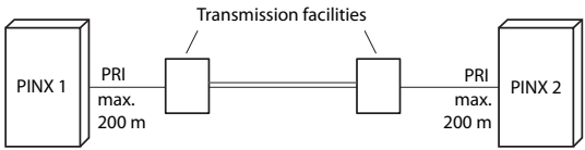
Fig. 36 Primaire snelheid-interface, in netwerk met transmissie-apparatuur
