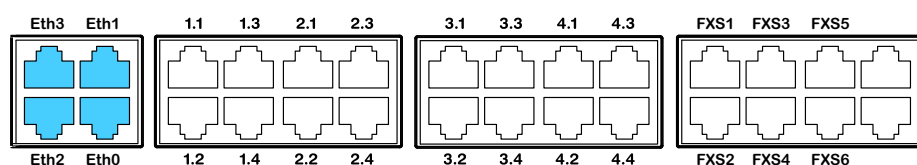
Fig. 59 Aansluitmogelijkheden voor Ethernet-interfaces
