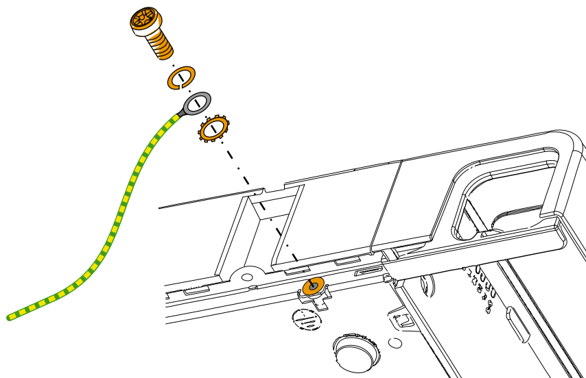
Fig. 18 Aardeaansluiting
