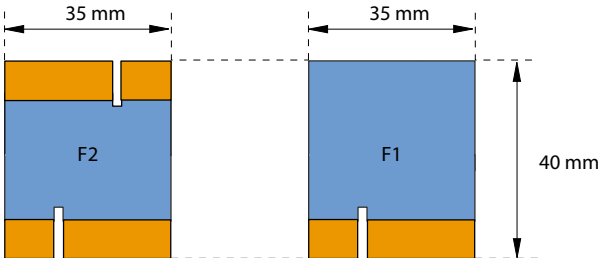
Fig. 82 Afmetingen van bedradingsadapter (ontwerp F)
