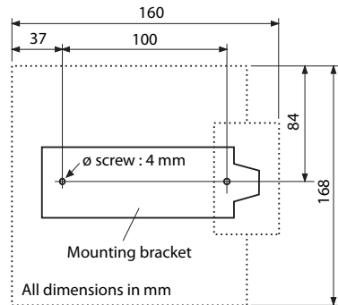
Fig. 62 Dimensionale tekening voor wandmontage van de montagebeugel
