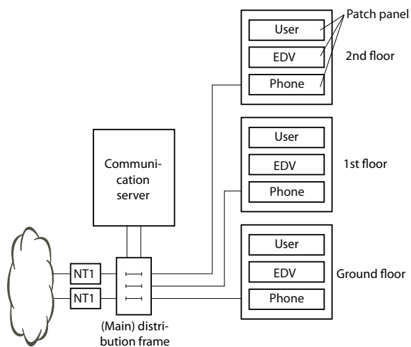
Fig. 26 Aansluiten op een UBC via een (hoofd) verdelerbord (voorbeeld)
