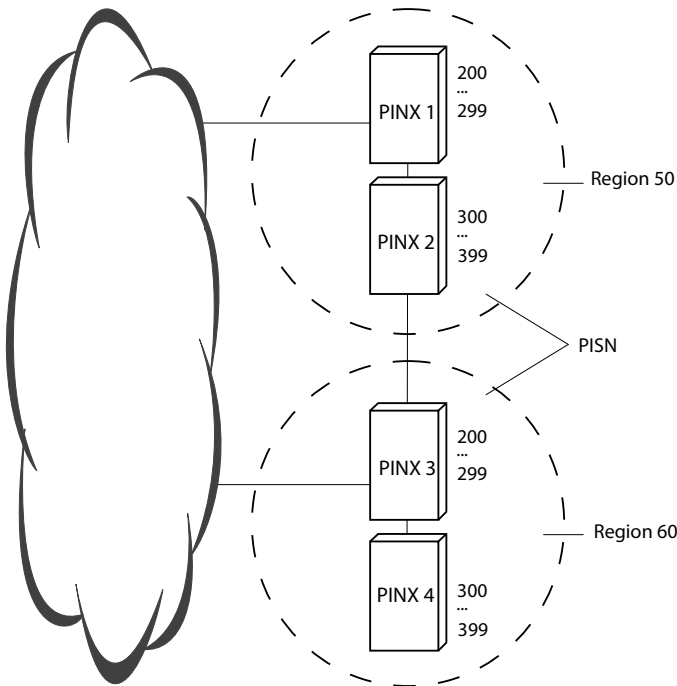
Fig. 25 PISN met twee regio's
