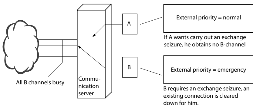
Fig. 97 Netwerktogangsrechten voor gebruikers met en zonder Prioriteitsexchangetoewijzing
