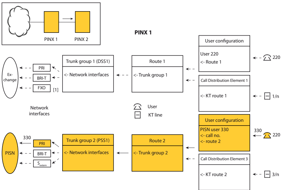
Fig. 99 Een oproep routeren naar het privé-huurlijnennetwerk
