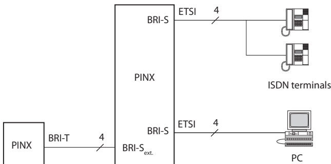
Fig. 18 Aansluitingsinterface BRI-S
