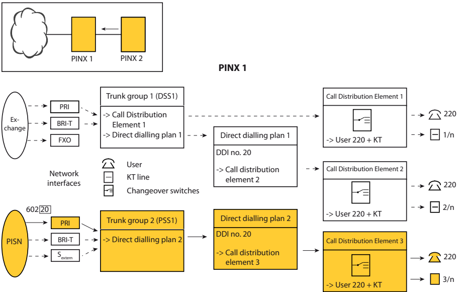
Fig. 86 Een oproep van het privé-huurlijnennetwerk routeren met snelkiezen
