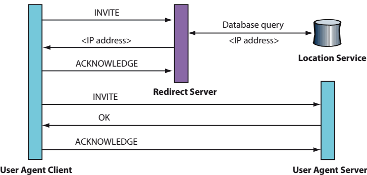
Fig. 14 Verbindingssetup met behulp van een Omleidingsserver
