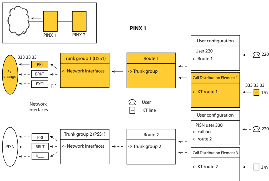
Fig. 95 Een oproep naar het openbare network via een lijntoets van een toetsentelefoon routeren
