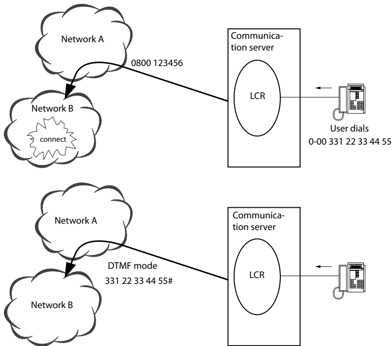
Fig. 108 Voorbeeld 2: Netwerkprovider B is niet geïntegreerd in het nummerschema van netwerkprovider A
