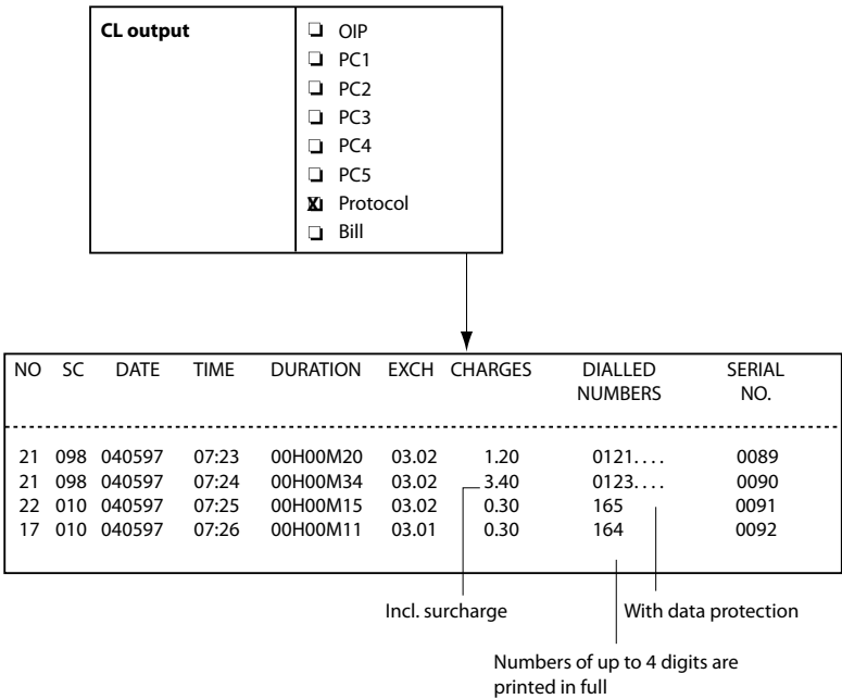
Fig. 174 CL-uitvoer in protocolindeling
