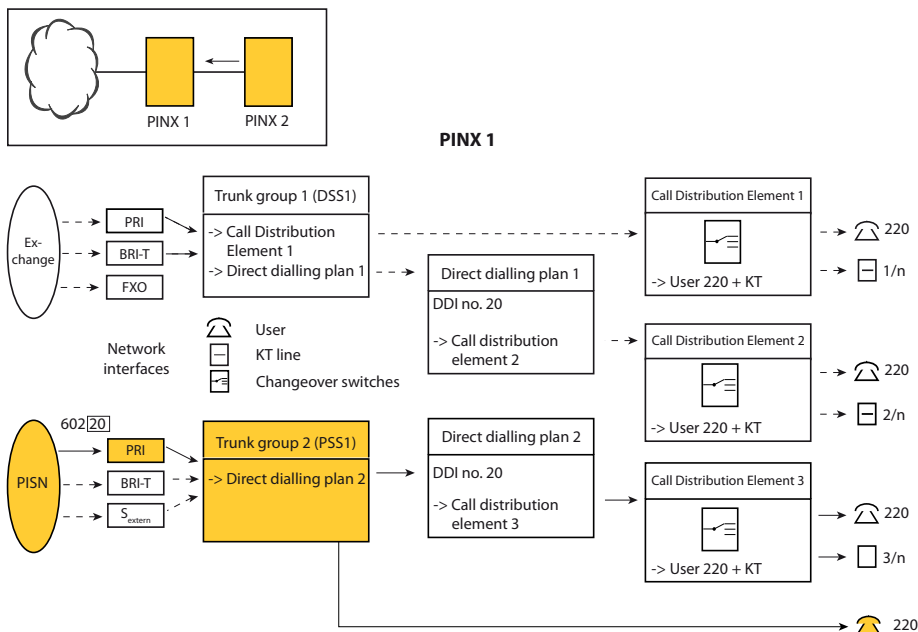
Fig. 87 Een oproep van het privé-huurlijnnennetwerk routeren zonder snelkiezen
