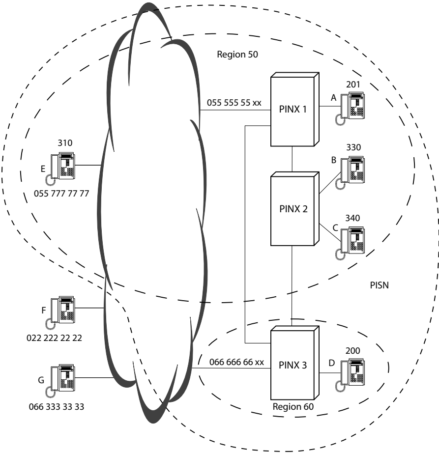
Fig. 40 Voorbeeldnetwerk: PISN met twee regio's en één virtuele netwerkgebruiker
