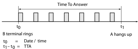
Fig. 164 Duur van de TTA-overgaan-fase
