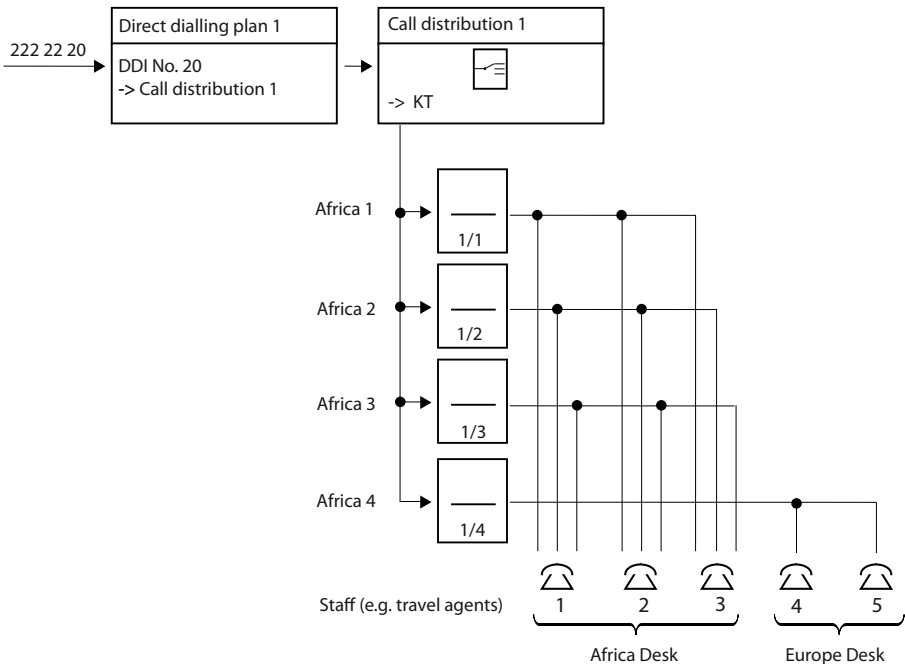
Fig. 75 Vervangingscircuit
