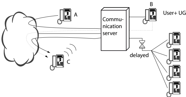
Fig. 187 DDI-nummer naar gebruiker + UG bezet
