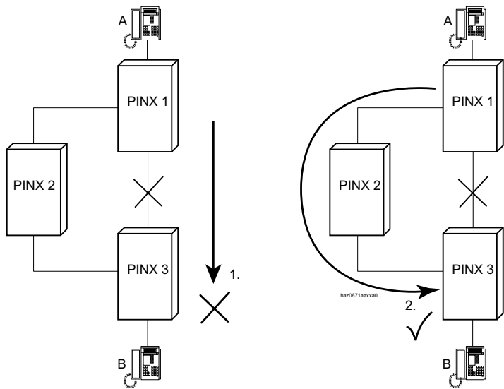
Fig. 122 Overflowrouting in het privé-huurlijnnetwerk via specifiek lijnen
