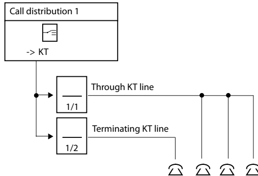
Fig. 73 Doorgaande- en KT-eindlijnen
