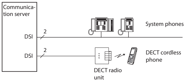
Fig. 19 DSI eindstationinterfaces
