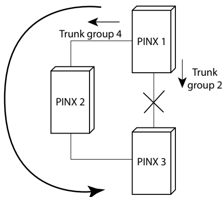
Fig. 123 Overflowrouting in het privé-huurlijnnennetwerk met behulp van een verstandige trunk-groep-toewijzing in de routeconfiguratie
