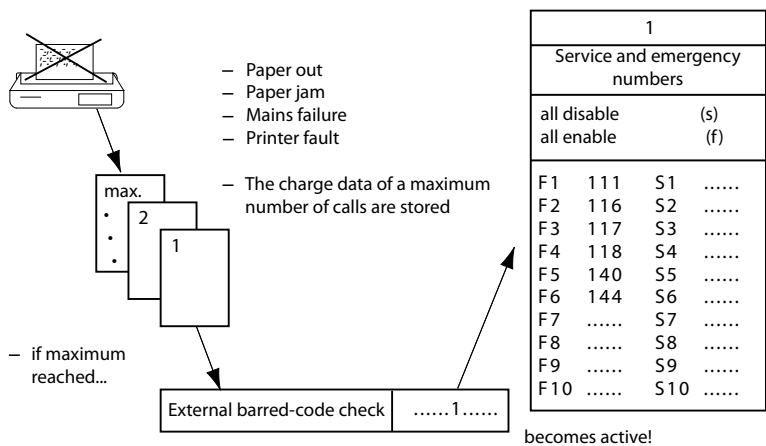
Fig. 148 Situatie als uitvoer geblokkeerd wordt
