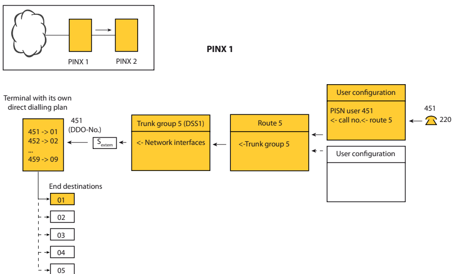
Fig. 100 Oproep naar een aansluiting met eigen snelkiesschema
