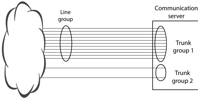
Fig. 51 Een lijngroep opnieuw creëren in de communicatieserver
