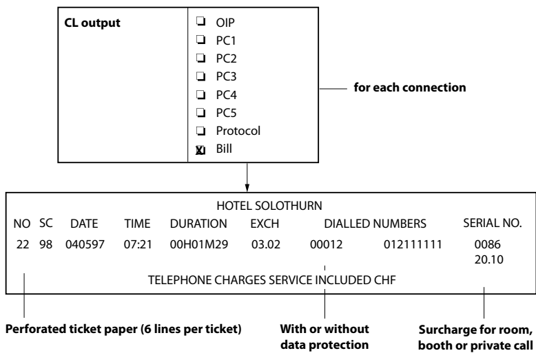
Fig. 175 CL-uitvoer in factuurindeling
