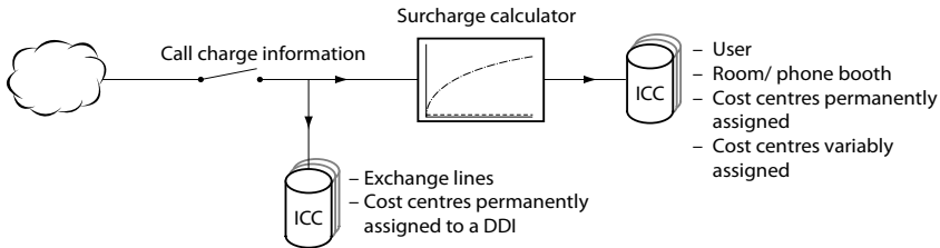
Fig. 135 Toewijzing van gesprekskosten
