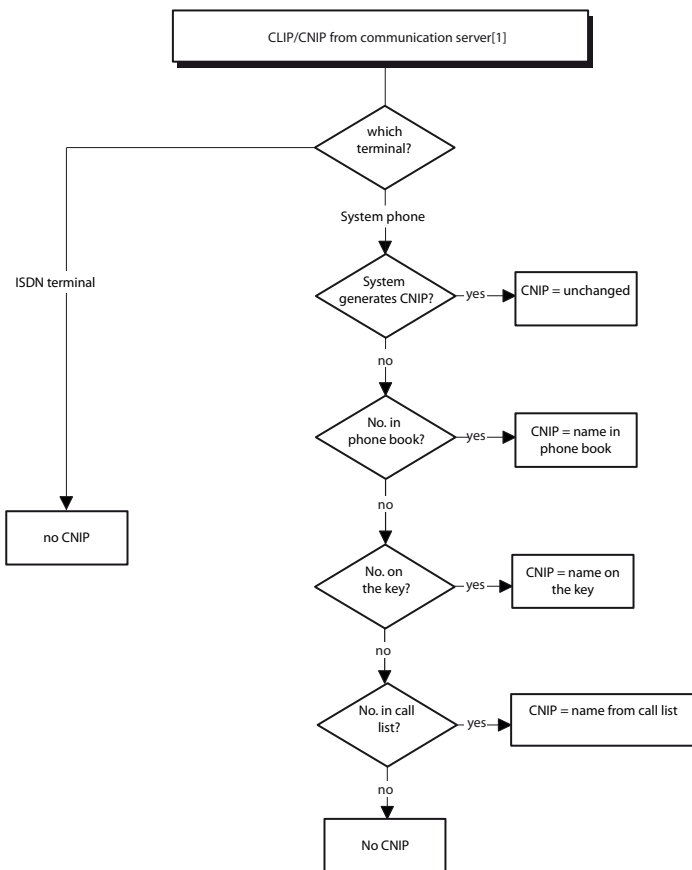
Fig. 34 Presentatie van de CLIP / CNIP van een inkomende oproep op de aansluiting
