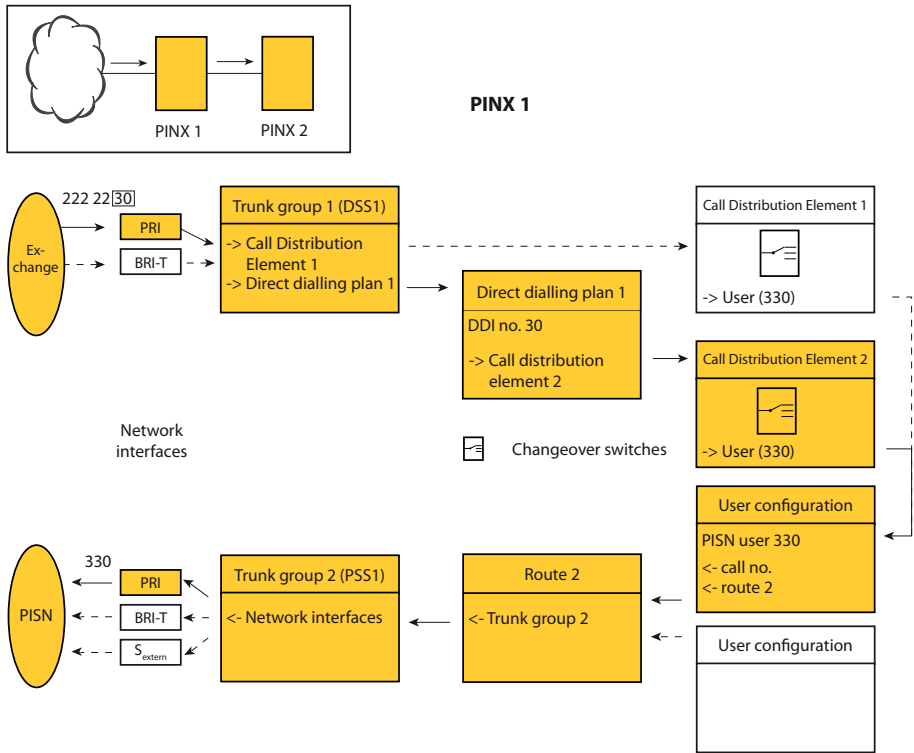
Fig. 117 Transitierouting van het openbare netwerk naar het privé-huurlijnnennetwerk met snelkiezen
