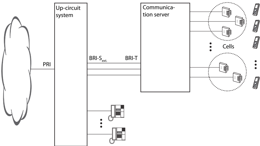
Fig. 9 Digitale down-circuitverbinding met QSIG
