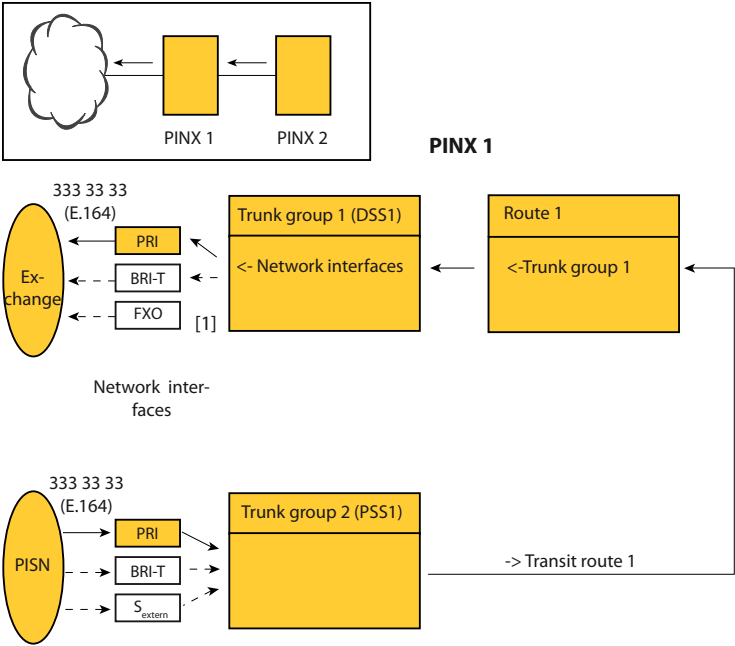
Fig. 119 Transitierouting van privé-huurlijnnetwerk → openbaar netwerk met NPI = E.164
