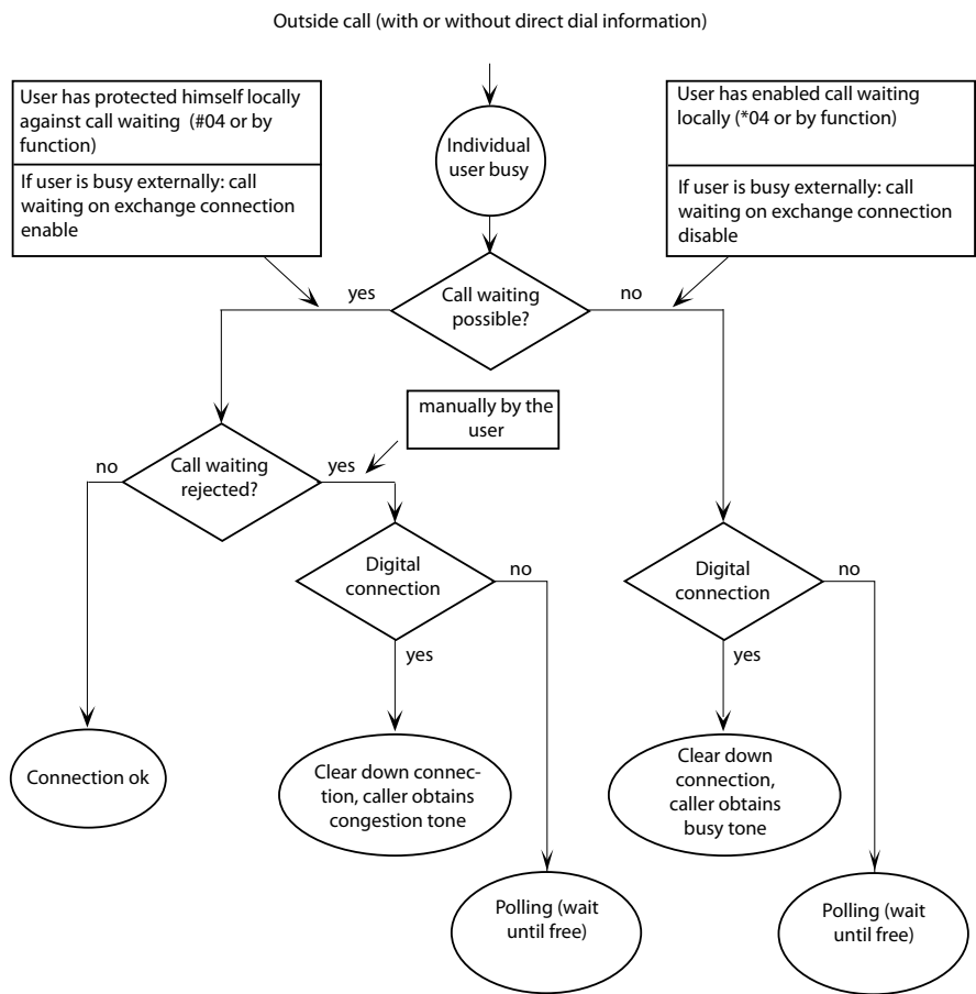
Fig. 89 Oproepdistributie als gebruiker bezet is
