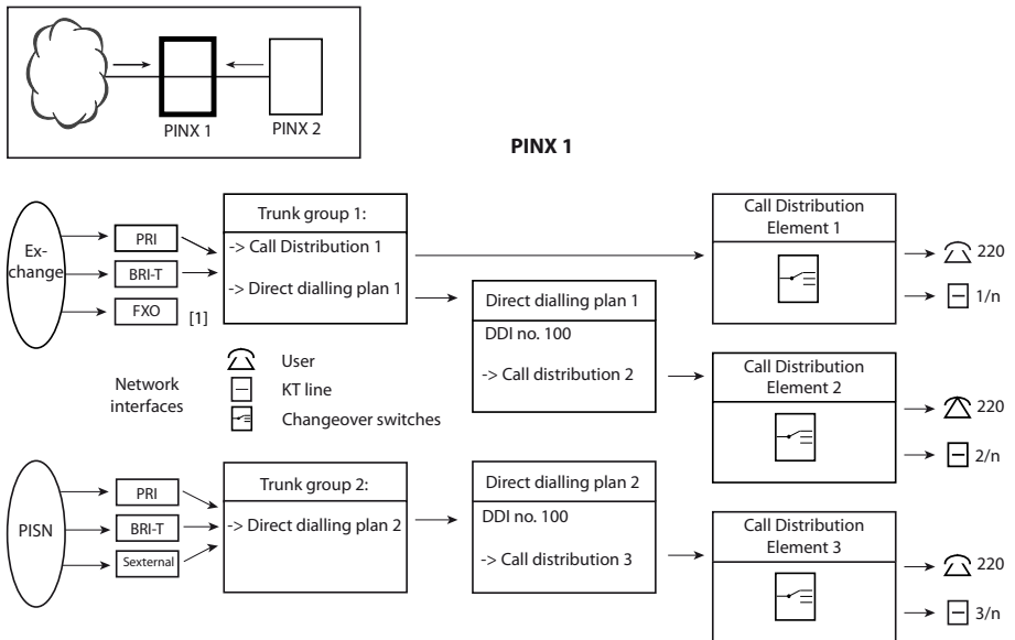
Fig. 82 Routing en bestemmingen van een inkomende oproep
