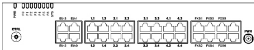
Figure 25: Interfaces op het voorpaneel met poortaanduiding (Mitel SMBC)
