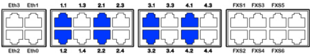
Figure 37: Aansluitmogelijkheden voor DSI eindstationinterfaces op meervoudig toegewezen RJ45 aansluitpunten
