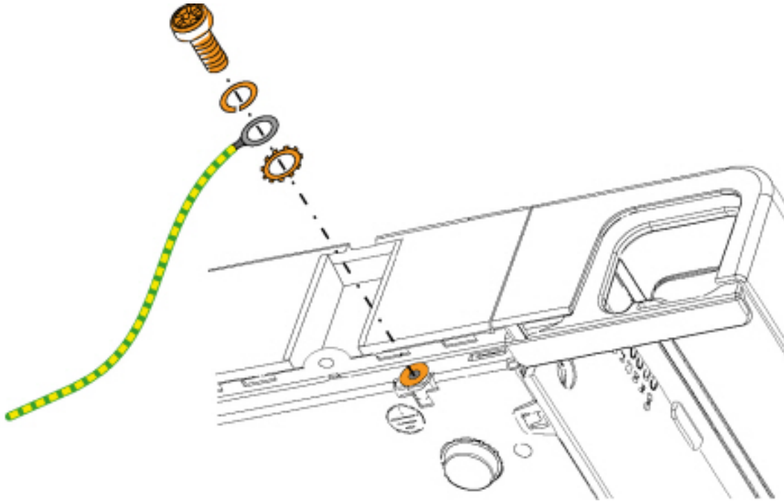
Figure 18: Aarding van de communicatieserver in het geval van een indirecte bekabeling en een directe bekabeling
