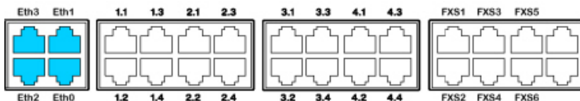
Figure 59: Aansluitmogelijkheden voor Ethernet-interfaces
