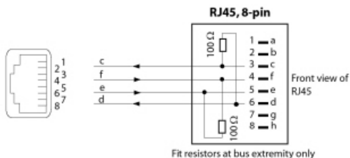
Figure 46: RJ45 aansluiting, enkel aansluitpunt
