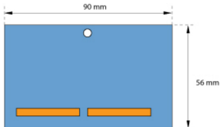
Figure 79: Afmetingen van systeemmodule (ontwerp D)
