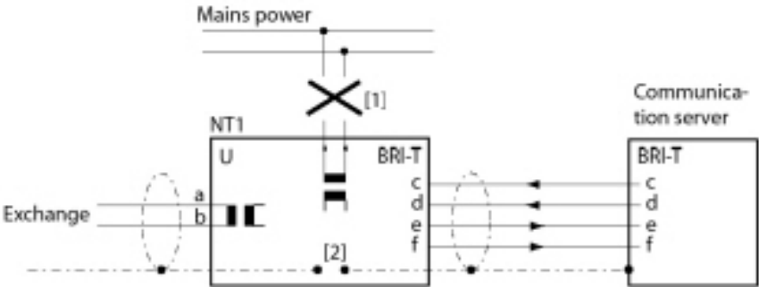
Figure 27: Basale toegang op NT1
