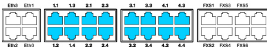
Figure 35: Aansluitmogelijkheden voor FXO netwerkinterfaces
