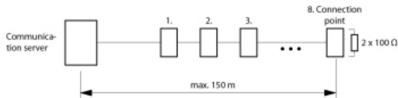
Figure 42: S-bus, kort
