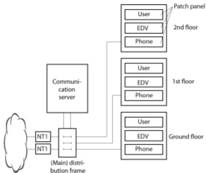
Figure 24: Aansluiten op een UBC via een bedradingscentrum (voorbeeld)
