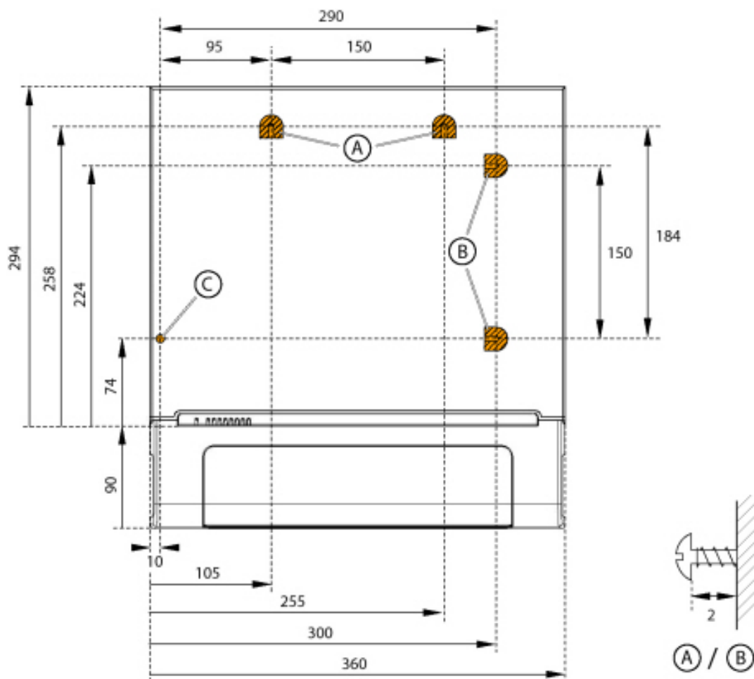
Figure 12: Boorschema voor wandmontage
