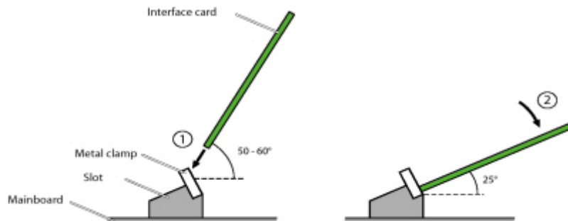
Figure 20: Installeren van een interfacekaart
