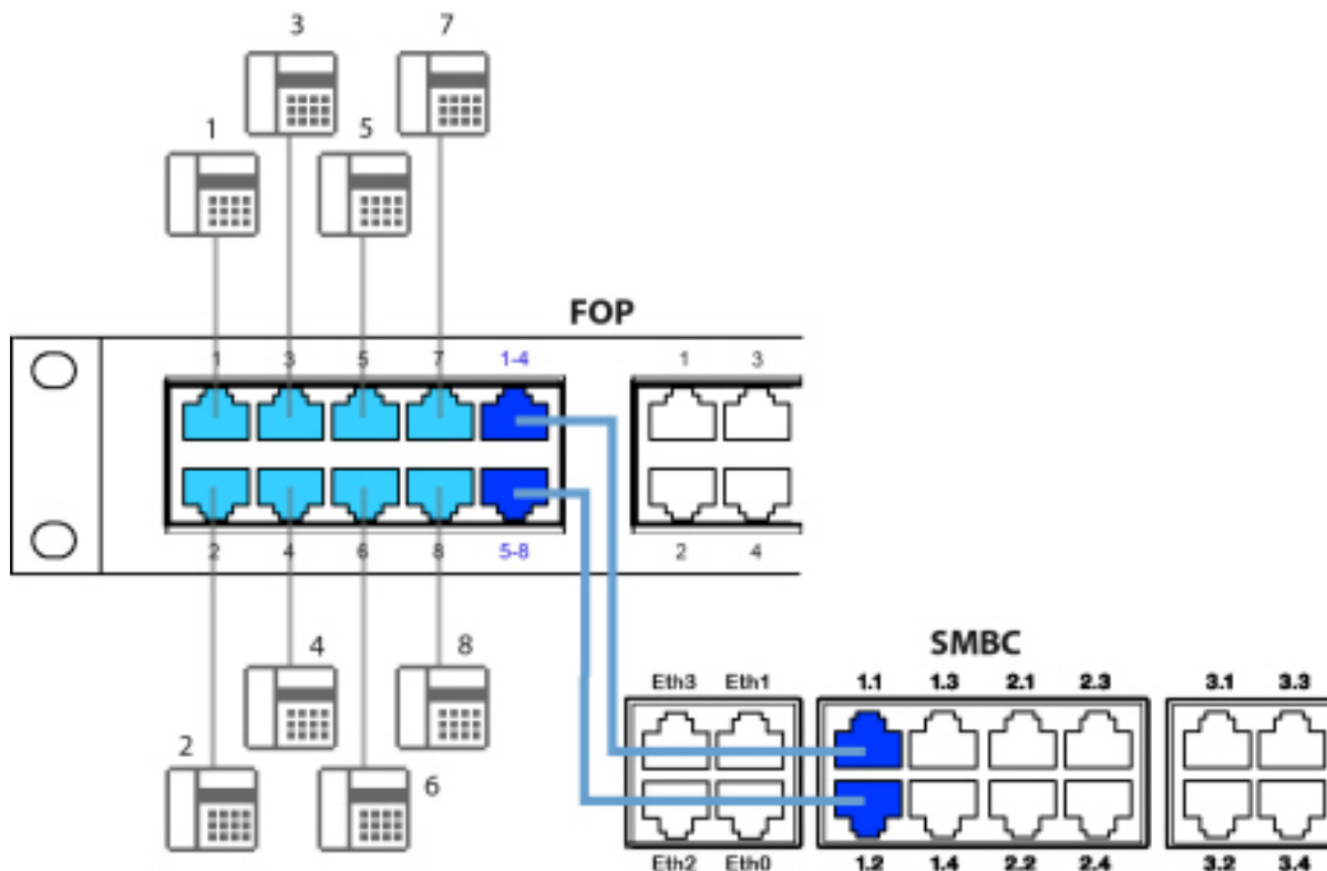
Figure 58: Aansluiting van viervoudig toegewezen aansluitpunten via FOP connectorstrip
