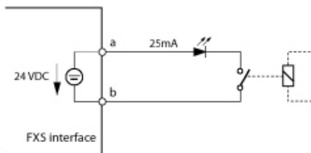
Figure 55: Aansluiting voor FXS modus: Regelingang
