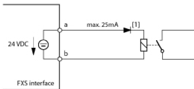
Figure 53: Aansluiting voor FXS modus: Stuuruitgang
