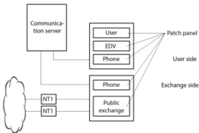
Figure 24: Aansluiten op een UBC via een bedradingscentrum (voorbeeld)
