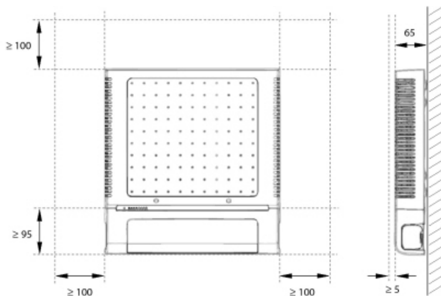
Figure 11: Minimale afstanden voor wandmontage (voorpaneel naar onder gericht)
