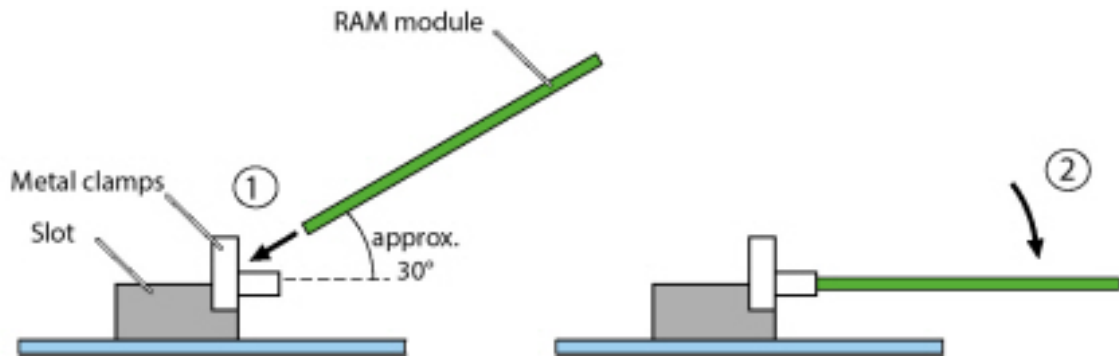
Figure 70: Verwisselen van de RAM-module
