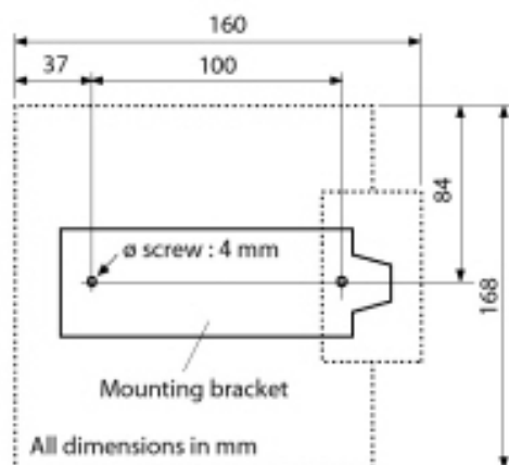
Figure 62: Dimensionale tekening voor wandmontage van de montagebeugel
