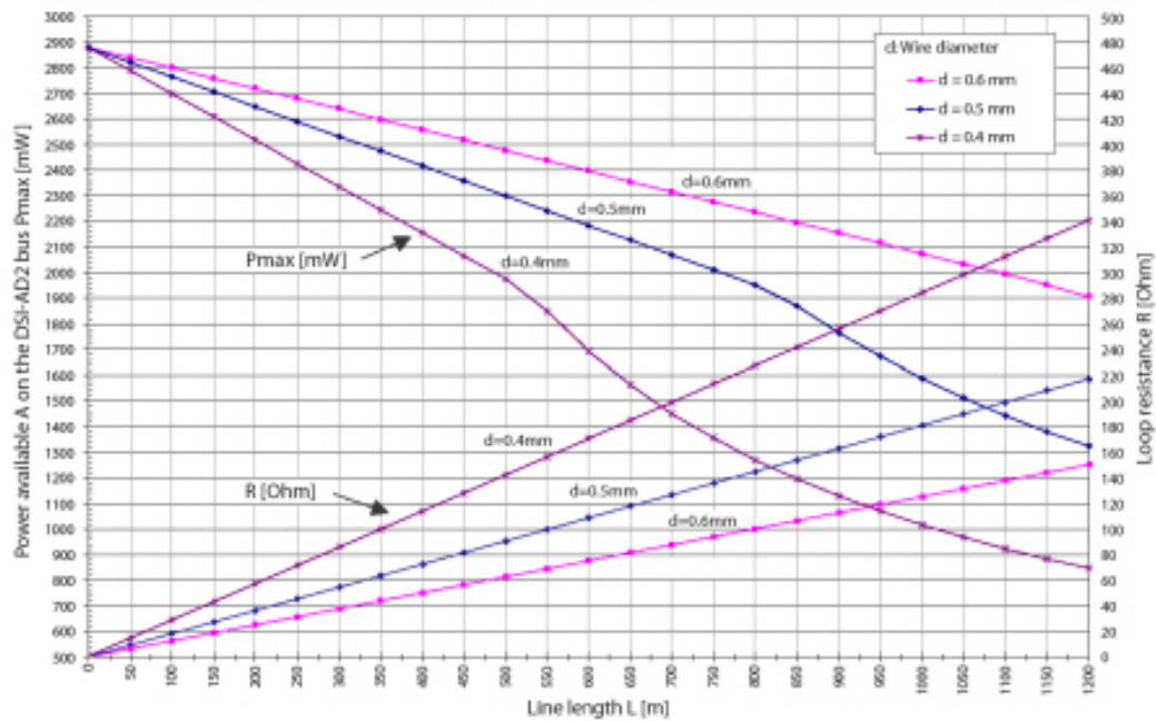
Figure 39: Beschikbaar vermogen geval A op de DSI-AD2 bus
