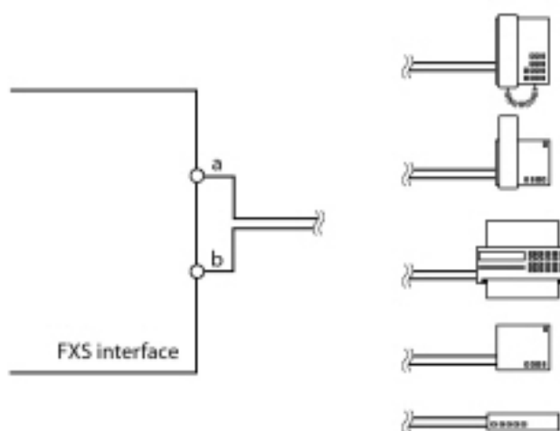
Figure 49: Aansluiting voor FXS modus: Telefoon/fax
