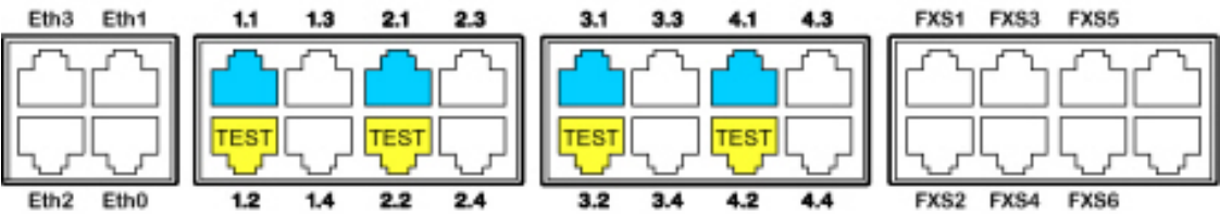
Figure 30: Aansluitmogelijkheden voor PRI netwerkinterfaces
