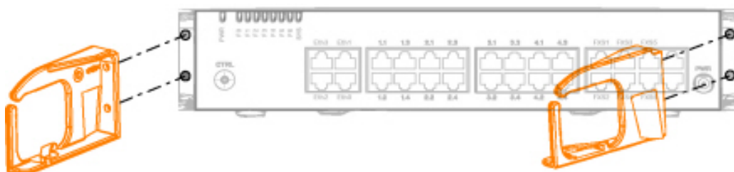
Figure 15: Installeren van de beugels voor de kabelafdekking
