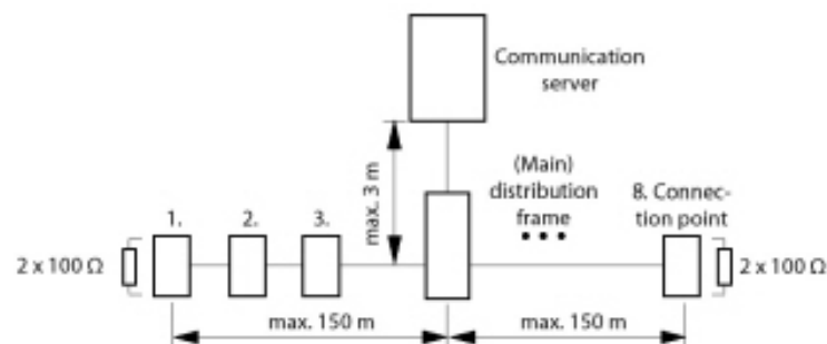
Figure 43: S-bus, kort, V-vormig
