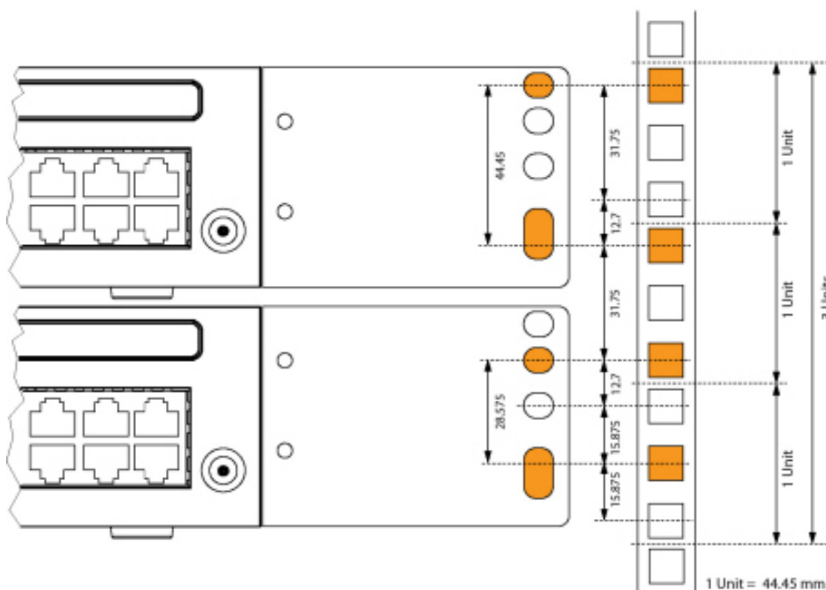
Figure 14: Het plaatsen van twee communicatieserver boven elkaar in een 19" rek
