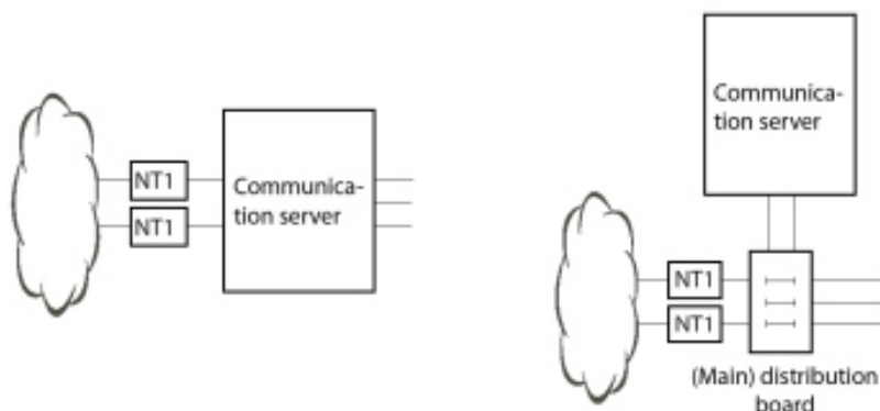
Figure 28: Directe bekabeling (links) en indirecte bekabeling (rechts)
