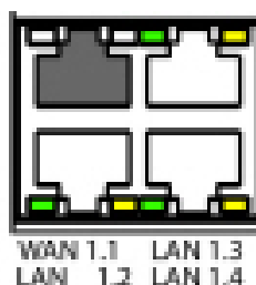
Figure 46: Status-LED op de Ethernet-interfaces
