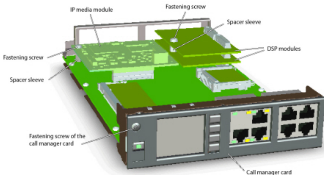
Figure 26: Systeemmodules op de gespreksmanagerkaart
