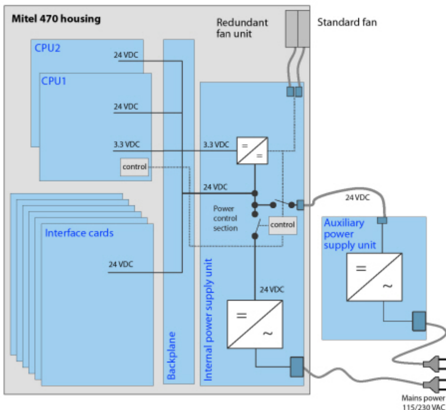
Figure 8: Overzicht van het Mitel 470 stroomvoorzieningsconcept
