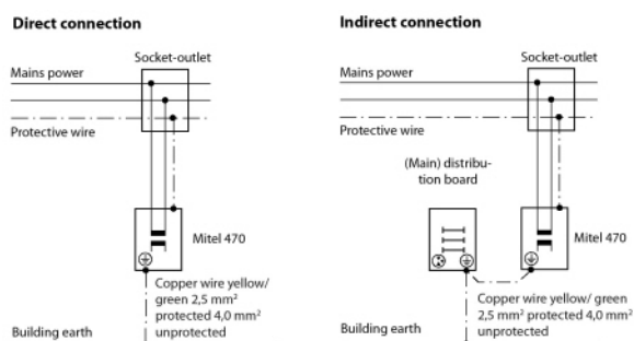
Figure 21: Aarding van de communicatieserver in het geval van een directe bekabeling en een indirecte bekabeling
