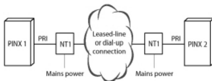
Figure 40: Toegang met primaire snelheid PRI, in een netwerk met gehuurde lijnen of kiesverbinding
