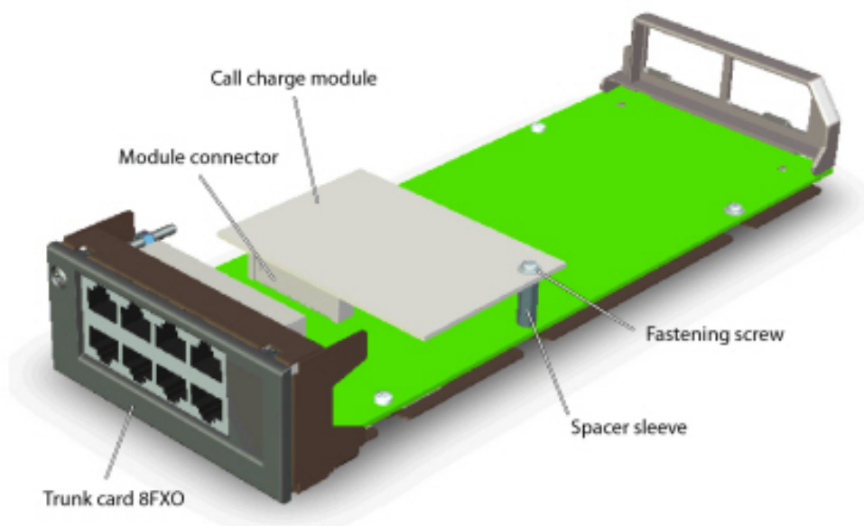
Figure 27: Gesprekskostenmodule op een 8FXO trunk-kaart
