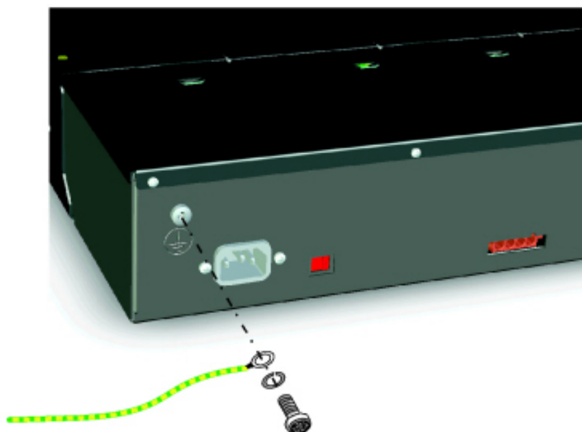
Figure 20: Aardeaansluiting
