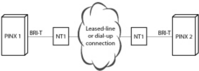
Figure 35: Basissnelheid-interface BRI-T, in een netwerk met gehuurde lijnen of kiesverbinding
