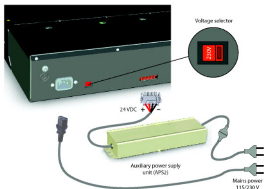
Figure 23: Stroomtoevoer naar de communicatieserver
