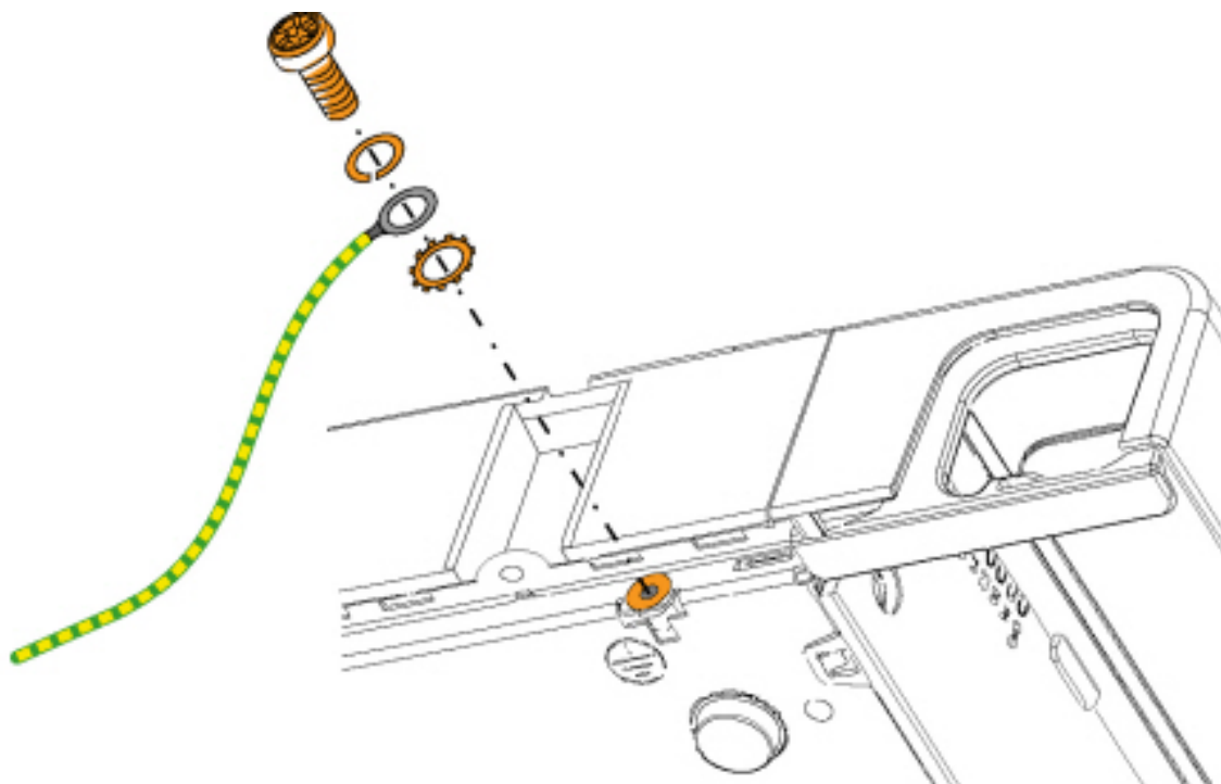
Figure 19: Aarding van de communicatieserver in het geval van een indirecte bekabeling en een directe bekabeling
