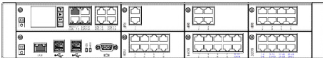
Figure 31: Interfaces op het voorpaneel met poort aanduiding (voorbeeld)
