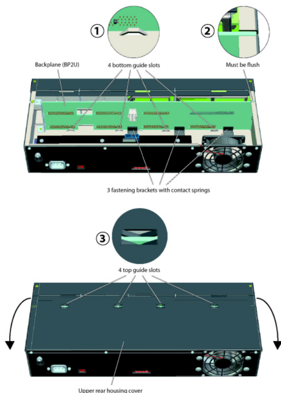
Figure 17: Correct zitten van BP2U op het achterpaneel
