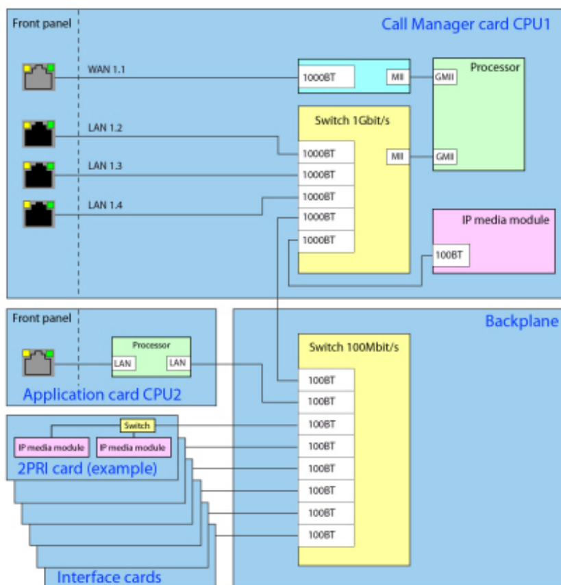
Figure 9: Overzicht van het Mitel 470 Ethernet-concept
