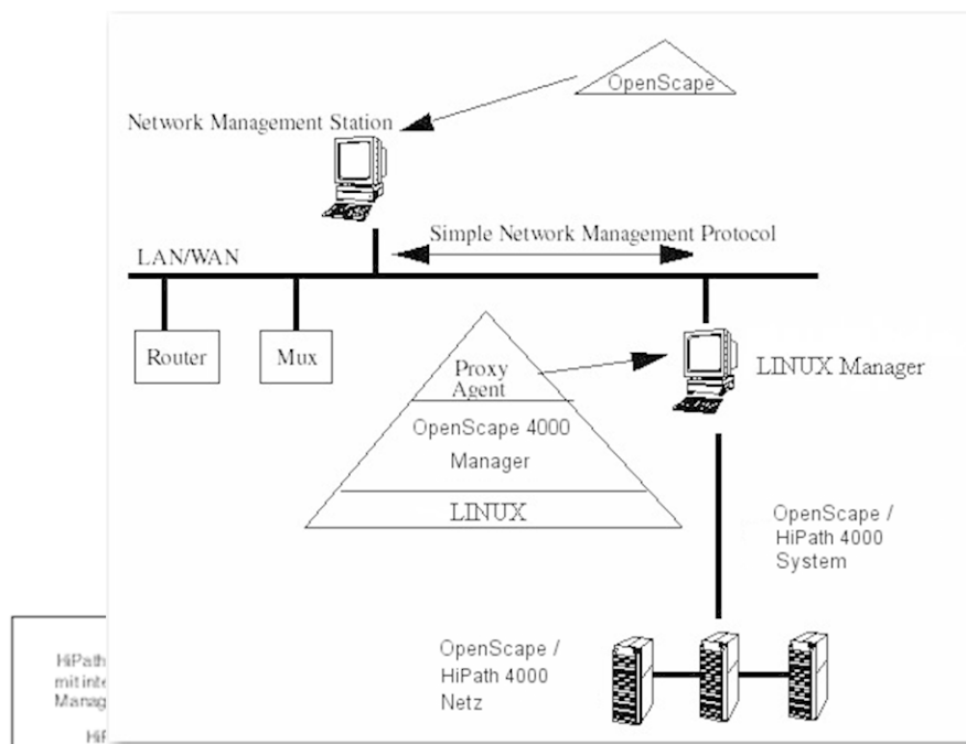
Figure 108: Komponentenstruktur des OpenScape SNMP Managements
