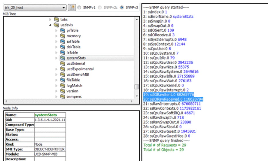
Figure 147: systemStats (sslORawSent.0 und sslORawRecieved.0)
