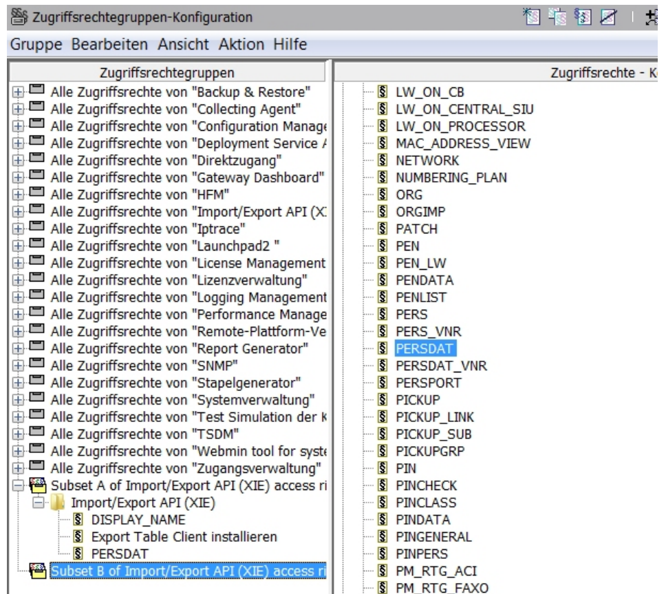
Abbildung 6: Benutzerspezifische Zugriffsrechtegruppen erzeugen
