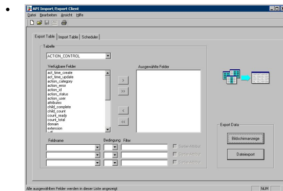
Abbildung 11: Hauptbildschirm von OpenScope 4000 Manager Import/Export Client
