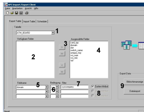
Abbildung 17: Das Register "Export Table"
