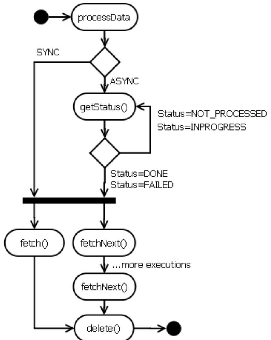
Abbildung 37: Reihenfolge der Operationen im Benutzerszenario
