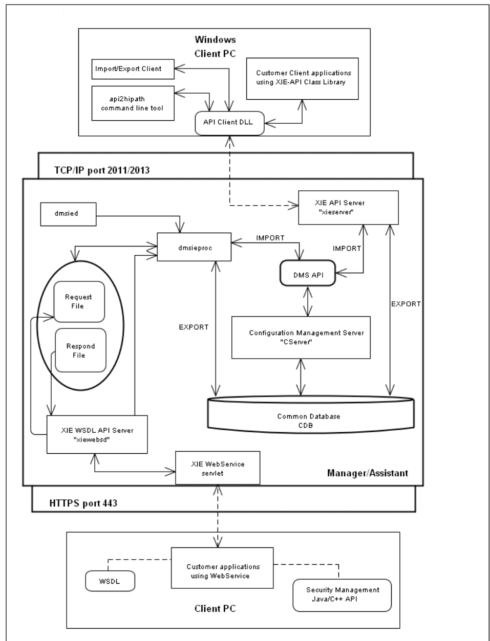
Abbildung 1: Datenaustausch über die XIE-API-Schnittstelle
