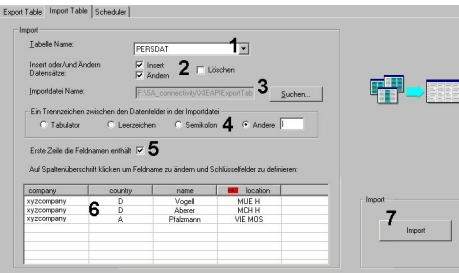
Abbildung 23: Import Table Property Page
