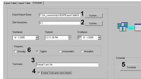
Abbildung 30: Scheduler Property Page
