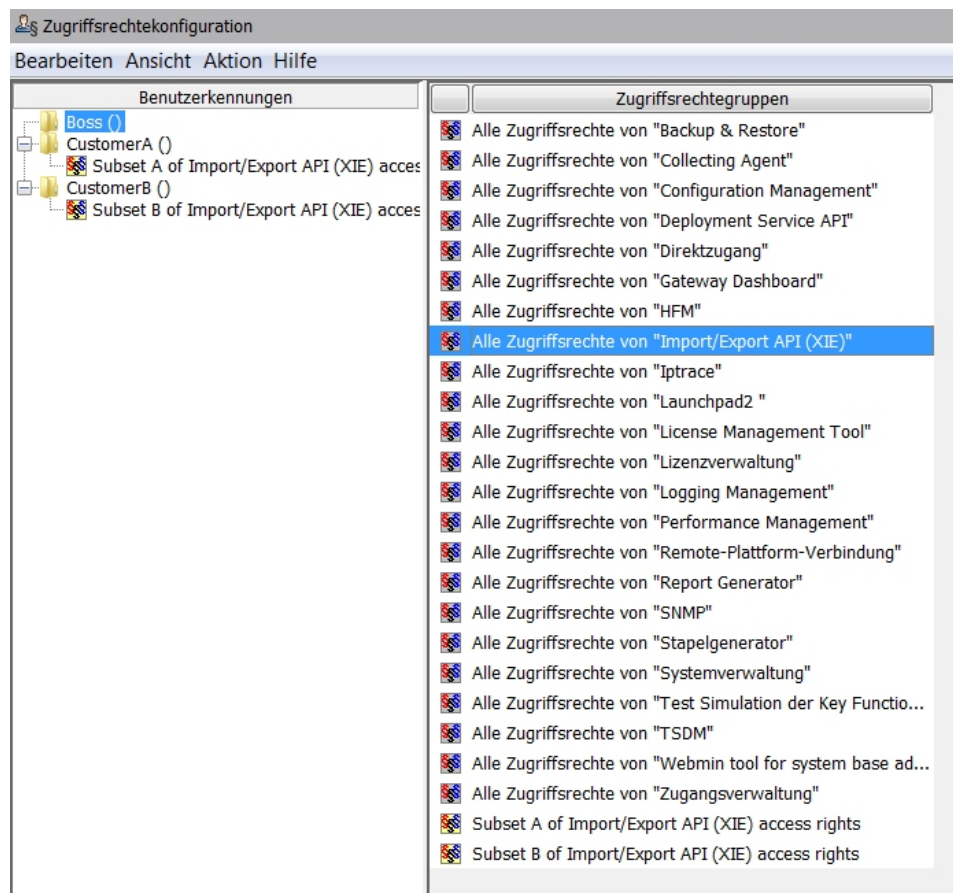
Abbildung 7: Bestimmten Benutzern Zugriffsrechte zuweisen
