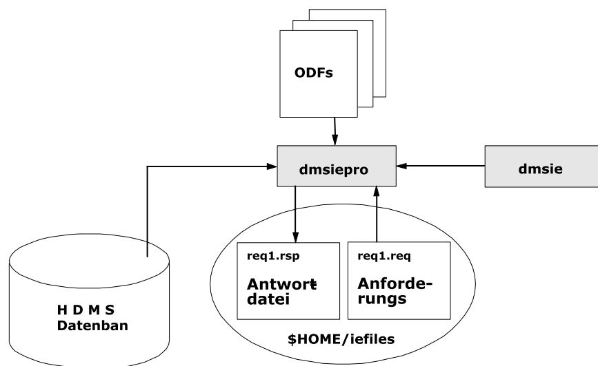
Abbildung 8: XIE-API Datenaustausch über Datei-Schnittstellen
