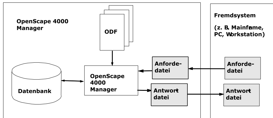
Abbildung 9: Anforderungs- und Antwortdateien
