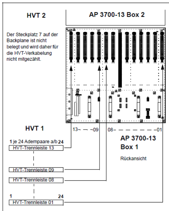
Abbildung 187: Kabelführung zwischen Box AP 3700-13 und HVT MDFHX6
