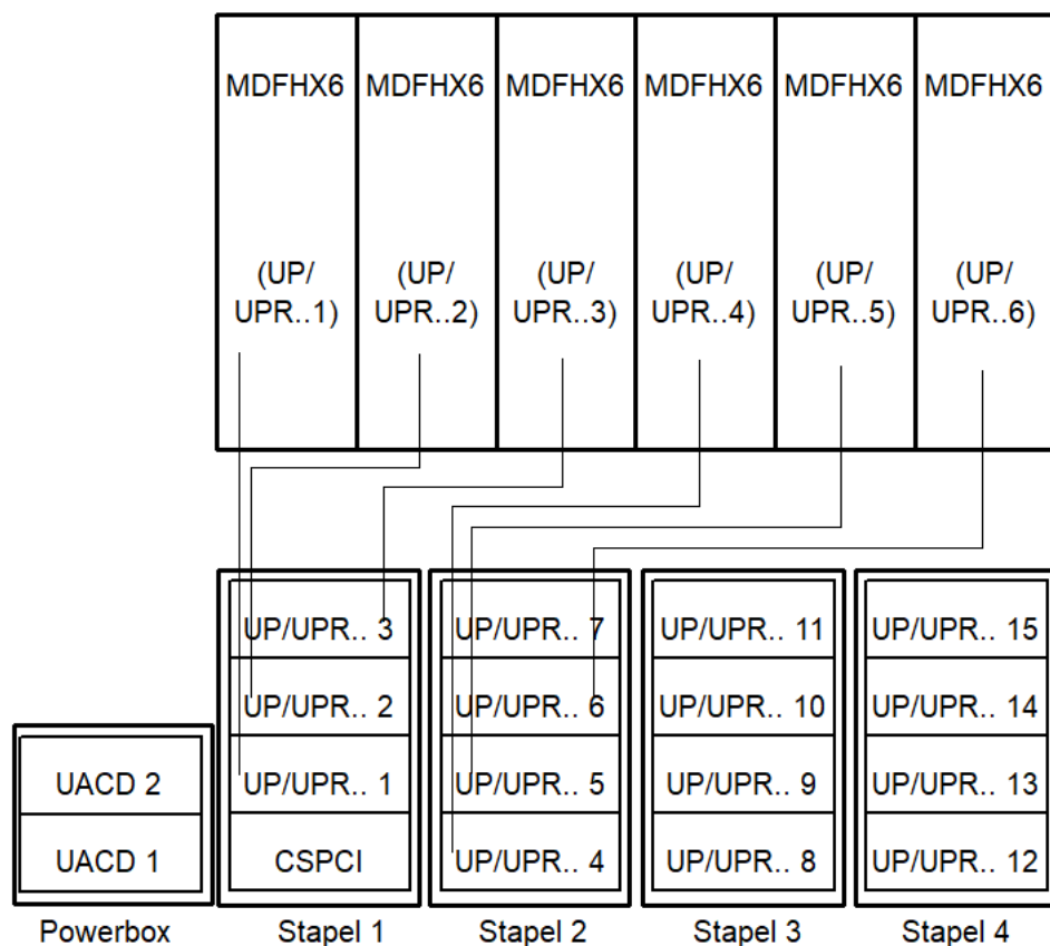
Abbildung 211: Erweiterter OpenScape 4000-Ausbau mit maximaler MDFHX6-Anzahl
