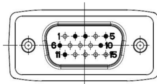
Abbildung 189: ALUM PIN-Belegung
