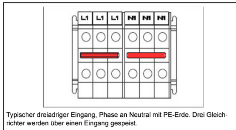
Abbildung 148: AC-Eingangsoption 1 (Einphasig)
