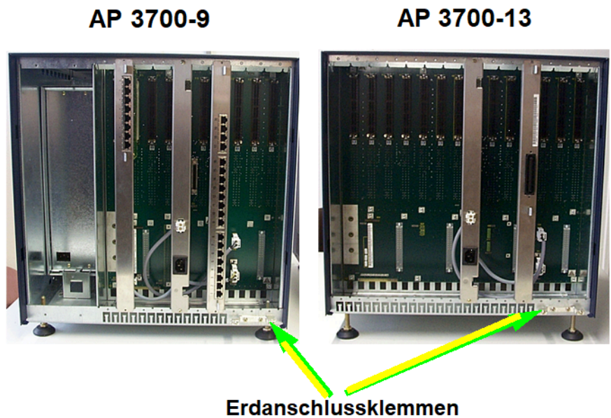
Abbildung 83: Erdanschlussklemmen AP 3700-9/AP 3700-13
