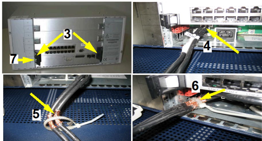
Abbildung 109: DC-Leitung an CSPCI-Box anschließen
