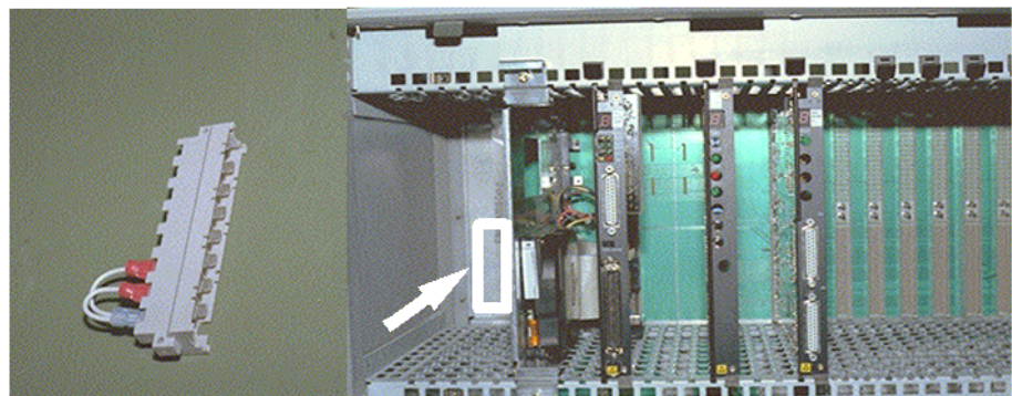
Abbildung 110: Brückenstecker (Jumper) OpenScape 4000
