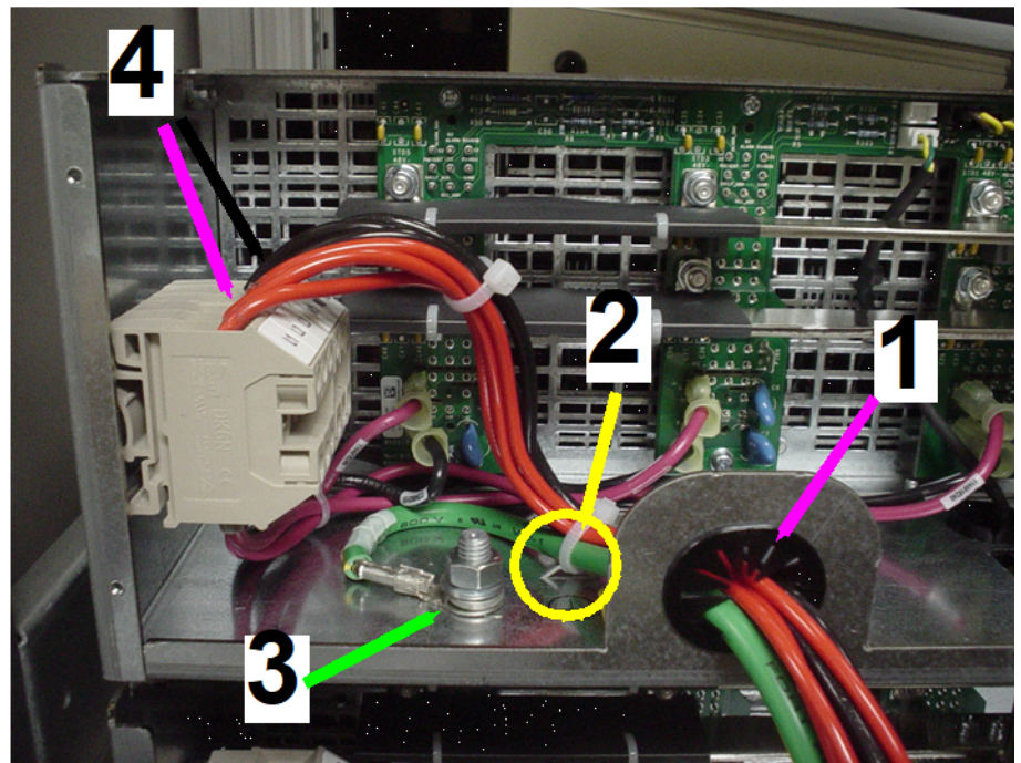
Abbildung 152: AC-Kabel verlegen
