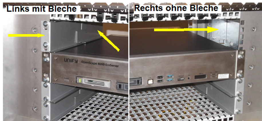
Abbildung 25: Luftleitbleche über EcoServer bei Simplex Betrieb
