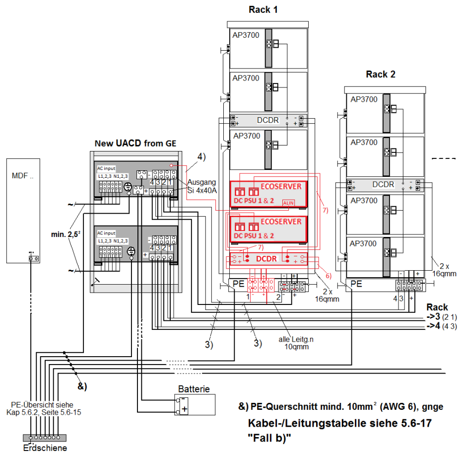
Abbildung 161: AC/DC-Anschaltung SAPP Boxes (von HP4 V2.0) mit "NEW" im 19" Schrank
