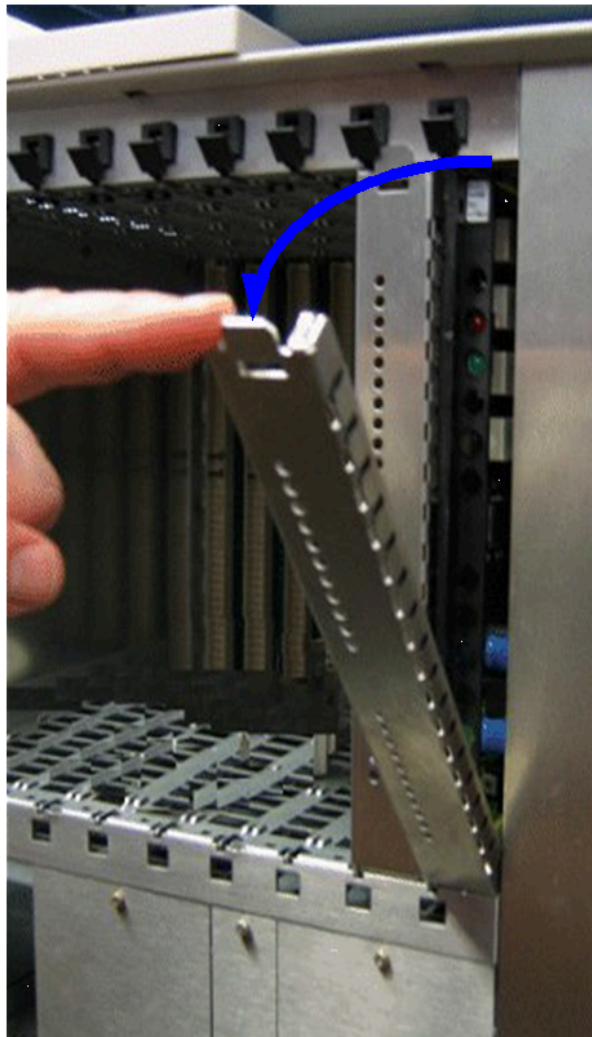
Abbildung 31: Abschirmblende montieren
