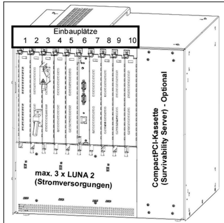
Abbildung 65: AP 3700-9 Vorderansicht
