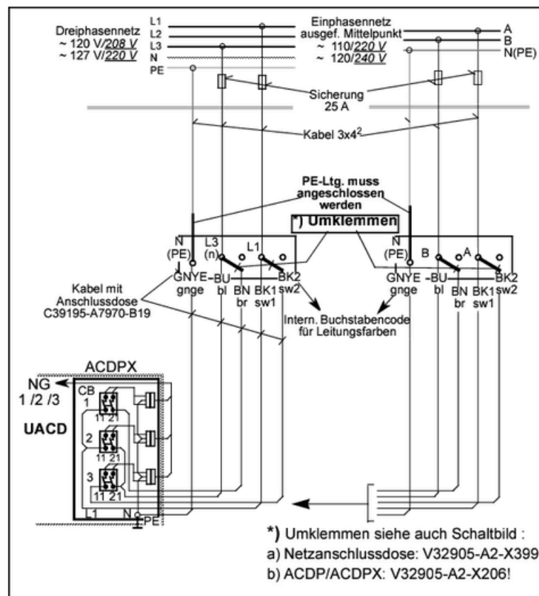
Abbildung 98: Dreiphasen-/Einphasenanschluss für zwei Netzgeräte
