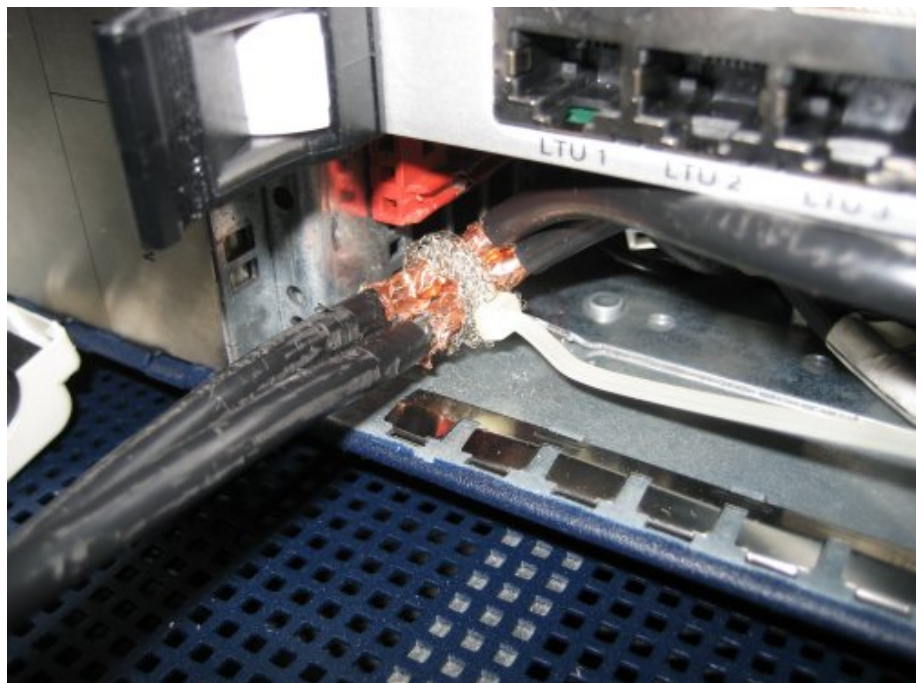
Abbildung 42: Schirmung der DC-Leitung an Gehäuse
