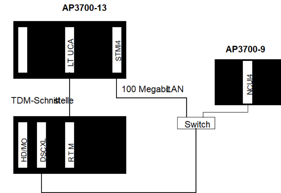
Baugruppe STMI4, Systemdiagramm
