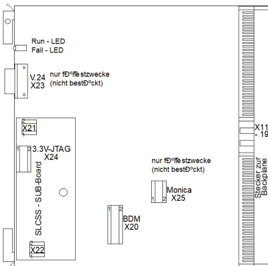
Baugruppenansicht X200
