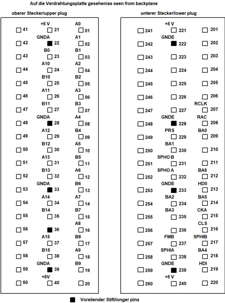
Steckerbelegung STMD
