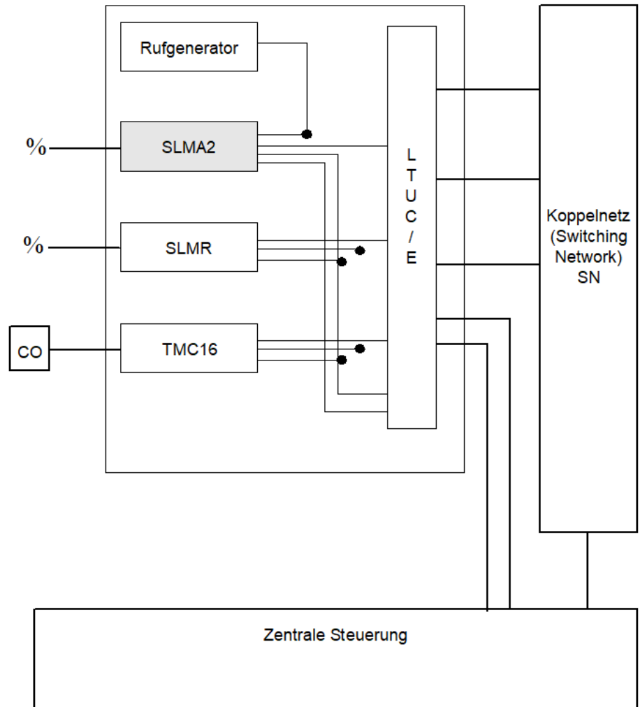
SLMA2, Systemarchitektur
