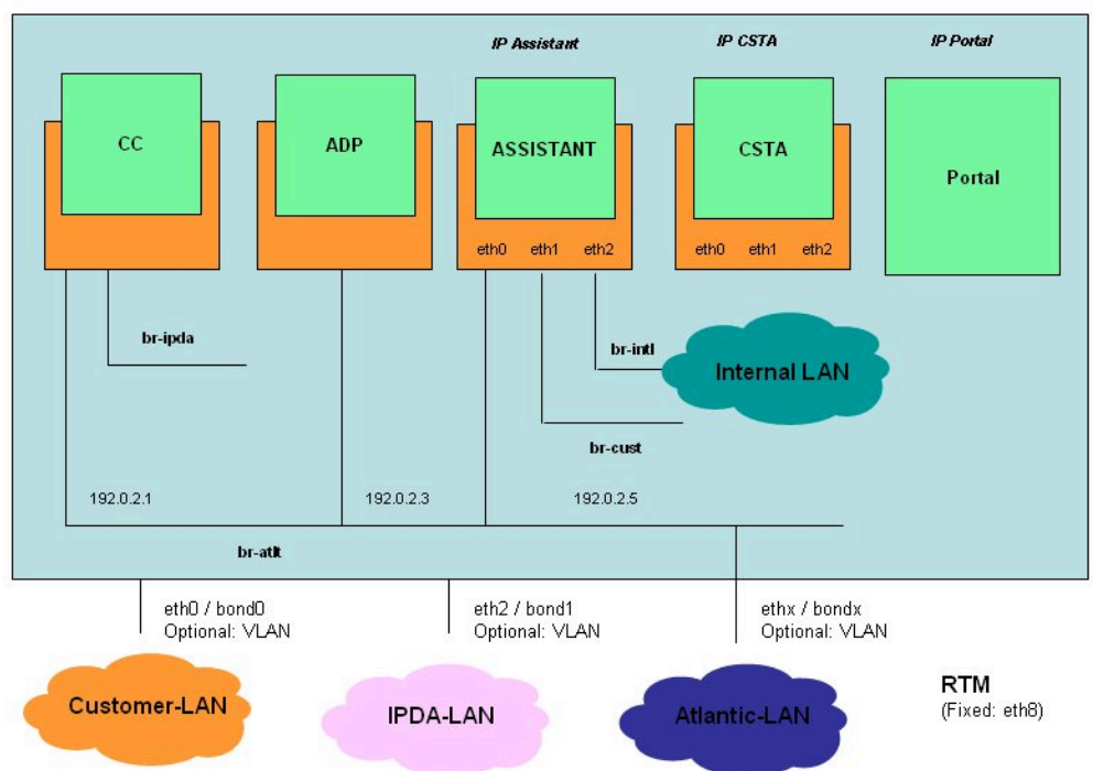
LAN-Schnittstellen
