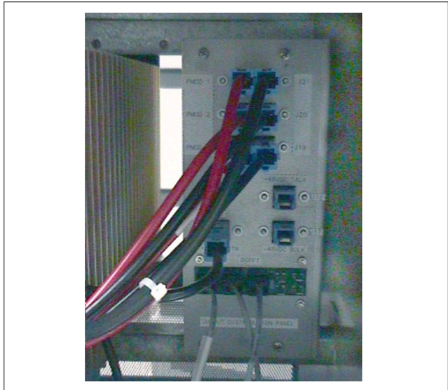
ODP, Rückansicht
