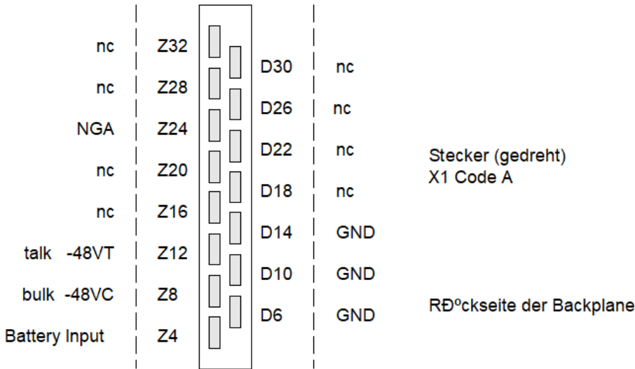
Steckerbelegung "ERNI H15"
