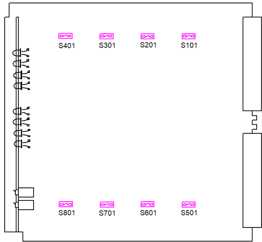
Baugruppe TMCOW
