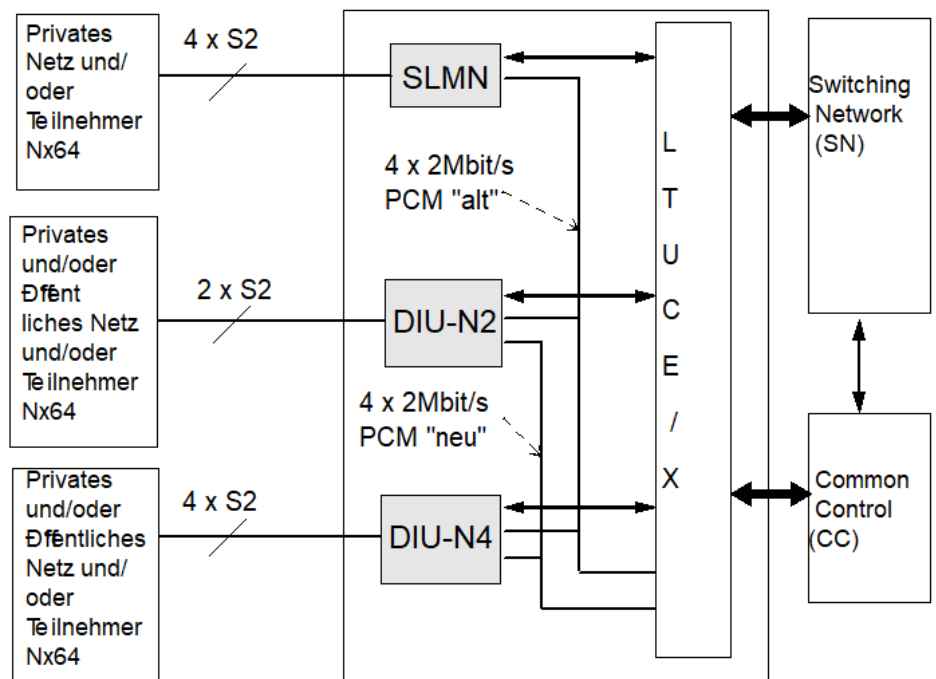
Figure 73: Funktionsschema zur Baugruppe DIUN2/DIUN4
