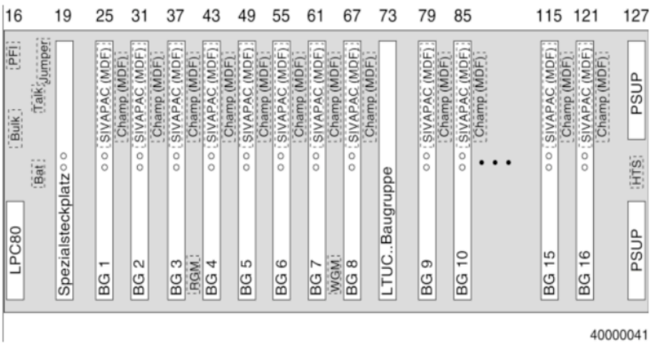
Figure 61: L80XF-Rückwandplatine
