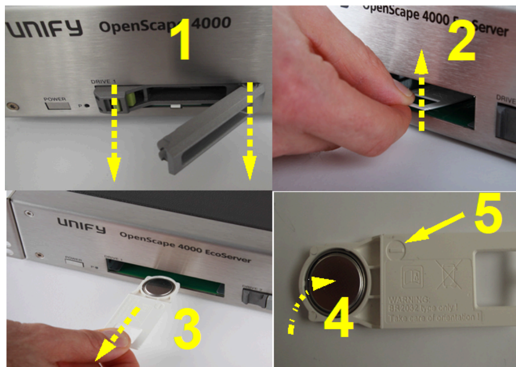
Figure 12: EcoServer: RTC-Batterie ersetzen
