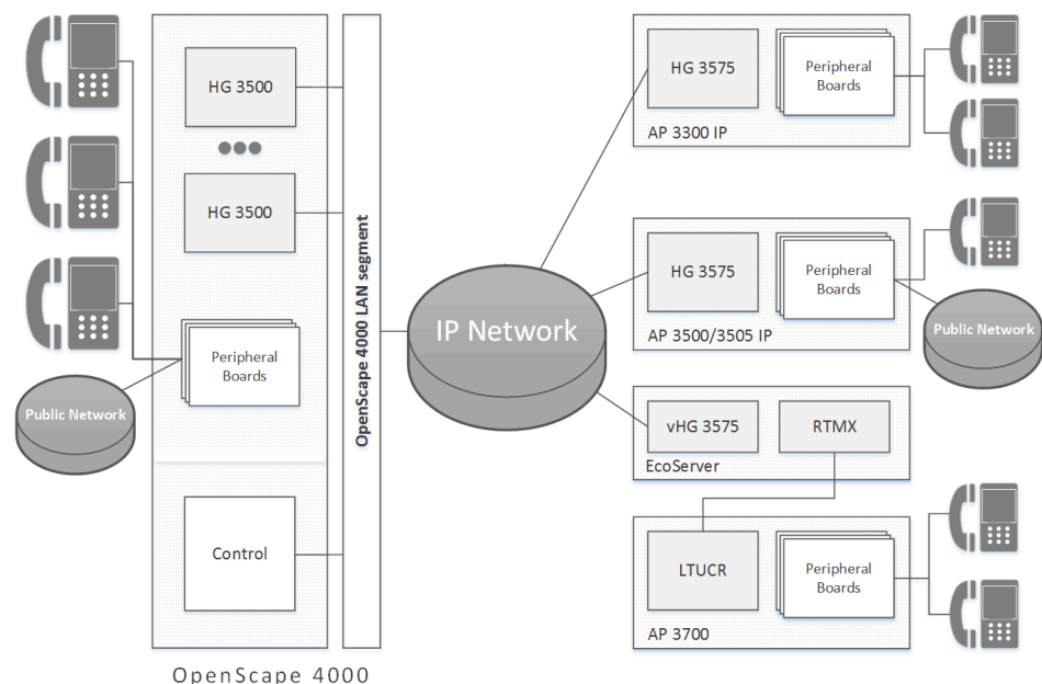
Figure 63: Systemarchitektur – Überblick
