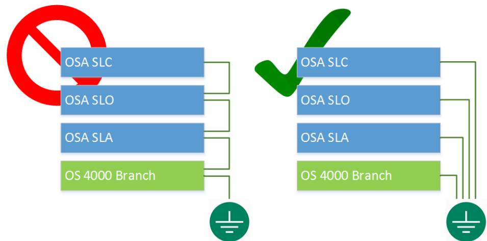
Figure 17: Das Erdungskonzept für die OpenScape 4000 Branch
