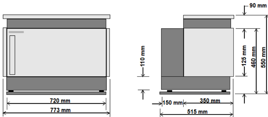
Figura 59: Sistema de uma caixa
