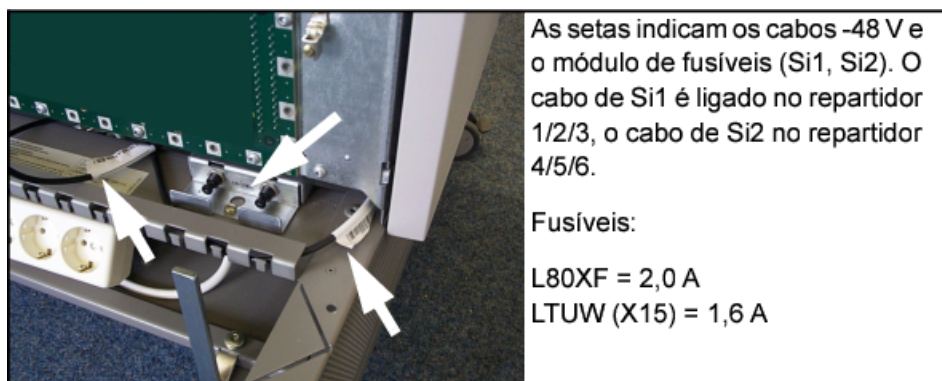
Figura 152: Módulo de fusíveis -48 V para repartidor (não-redundante)
