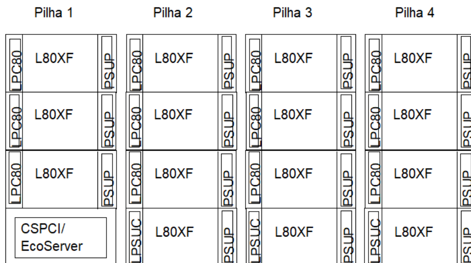
Figura 1: OpenScape 4000, configuração de rede não-redundante
