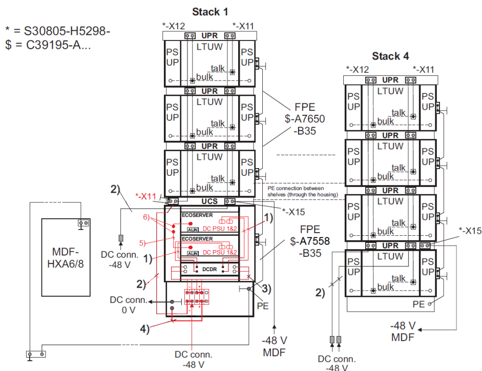
Figura 148: Ligação DC com módulo UPR/LTUW redundante (versão IM - internacional)
