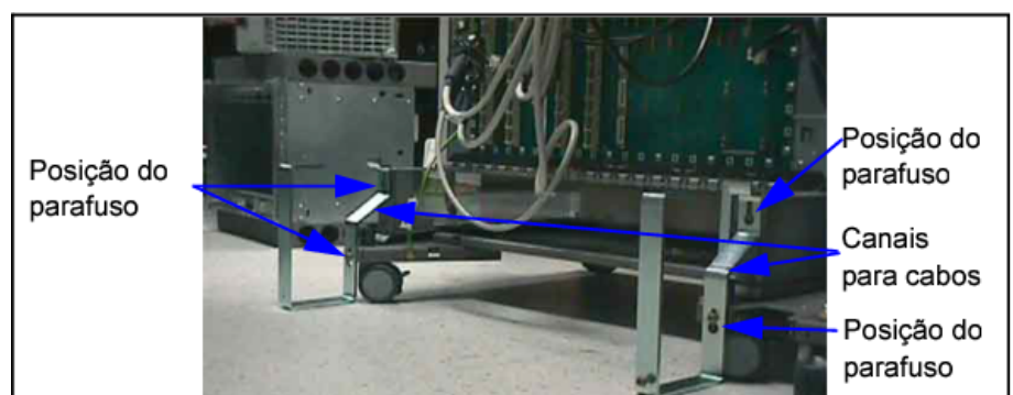
Figura 23: Canais para cabos
