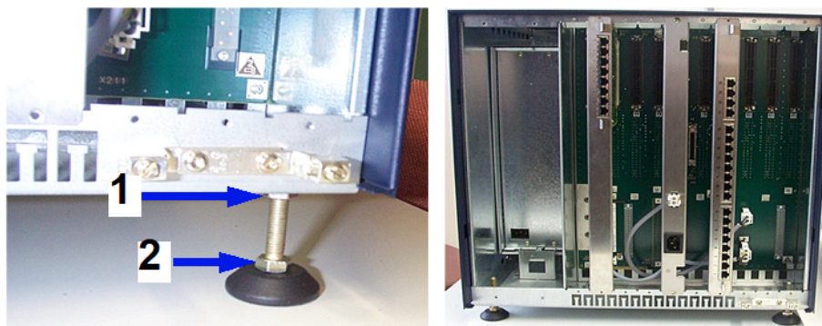
Figura 11: Ajuste da altura dos pés de apoio
