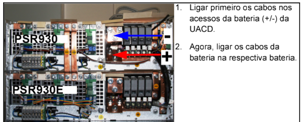
Figura 201: Ligação da bateria na UACD (PSR930/PSR930E)
