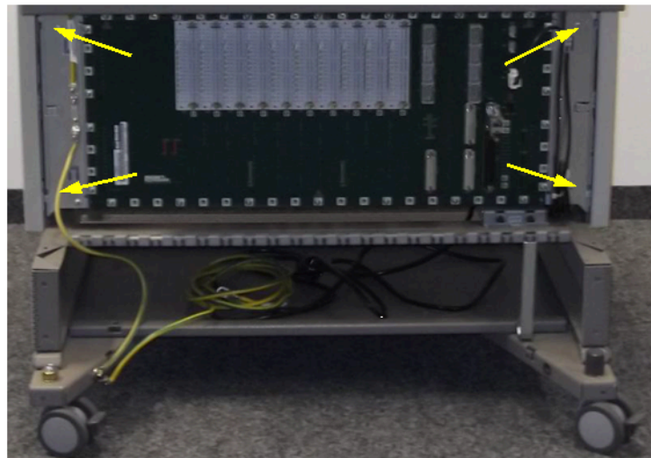
Figura 35: Remover a fixação CCDAX
