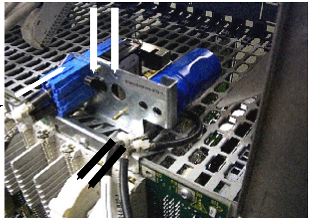
Figure 177: Unité de raccordement -48 V pour REP (redondante)
