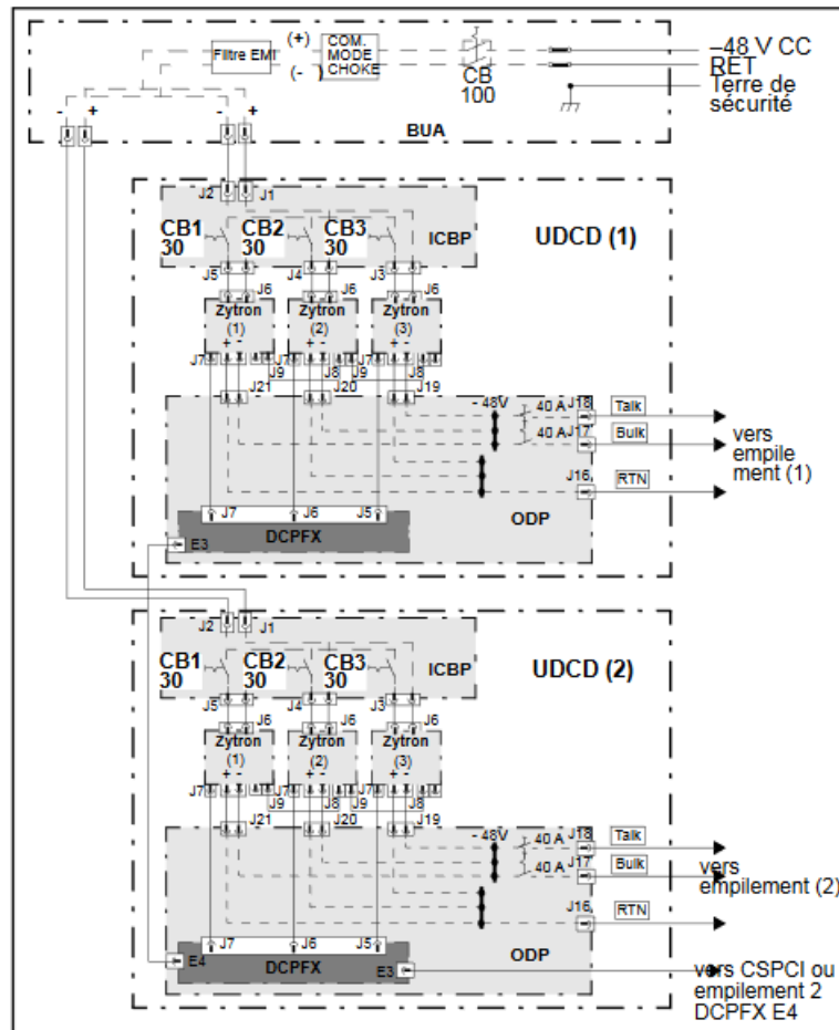
Figure 174: Vue d'ensemble des raccordements Empilement UDCD 1
