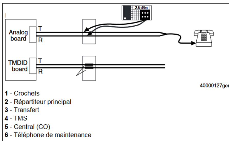
Figure 209: Banc de contrôle pour les mesures ERL/SRL sur les canaux de lignes SDA
