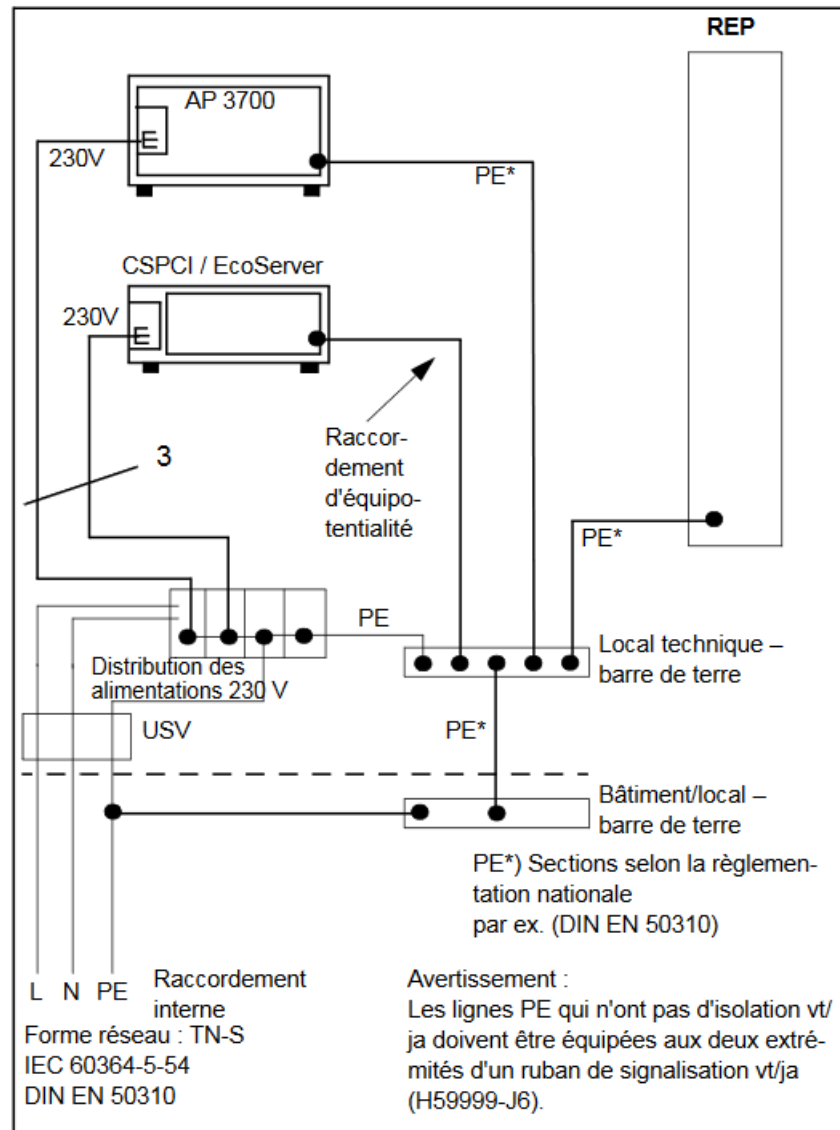
Figure 86: Configuration de terre pour raccordement CA autonome
