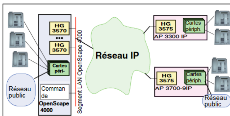
Figure 200: Vue d'ensemble de l'architecture
