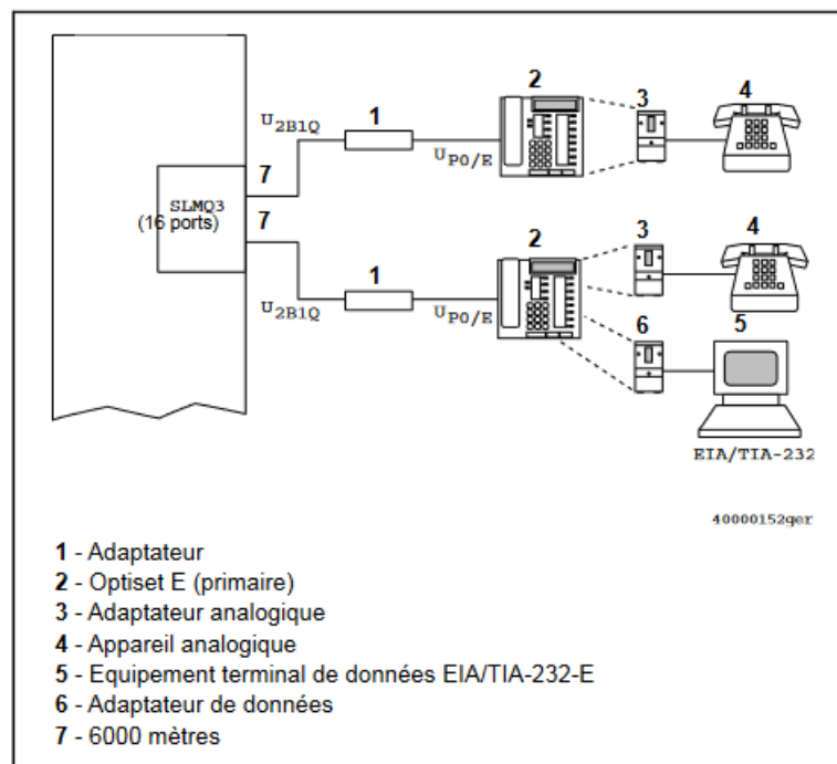
Figure 198: Possibilité de raccordement de l'adaptateur distant
