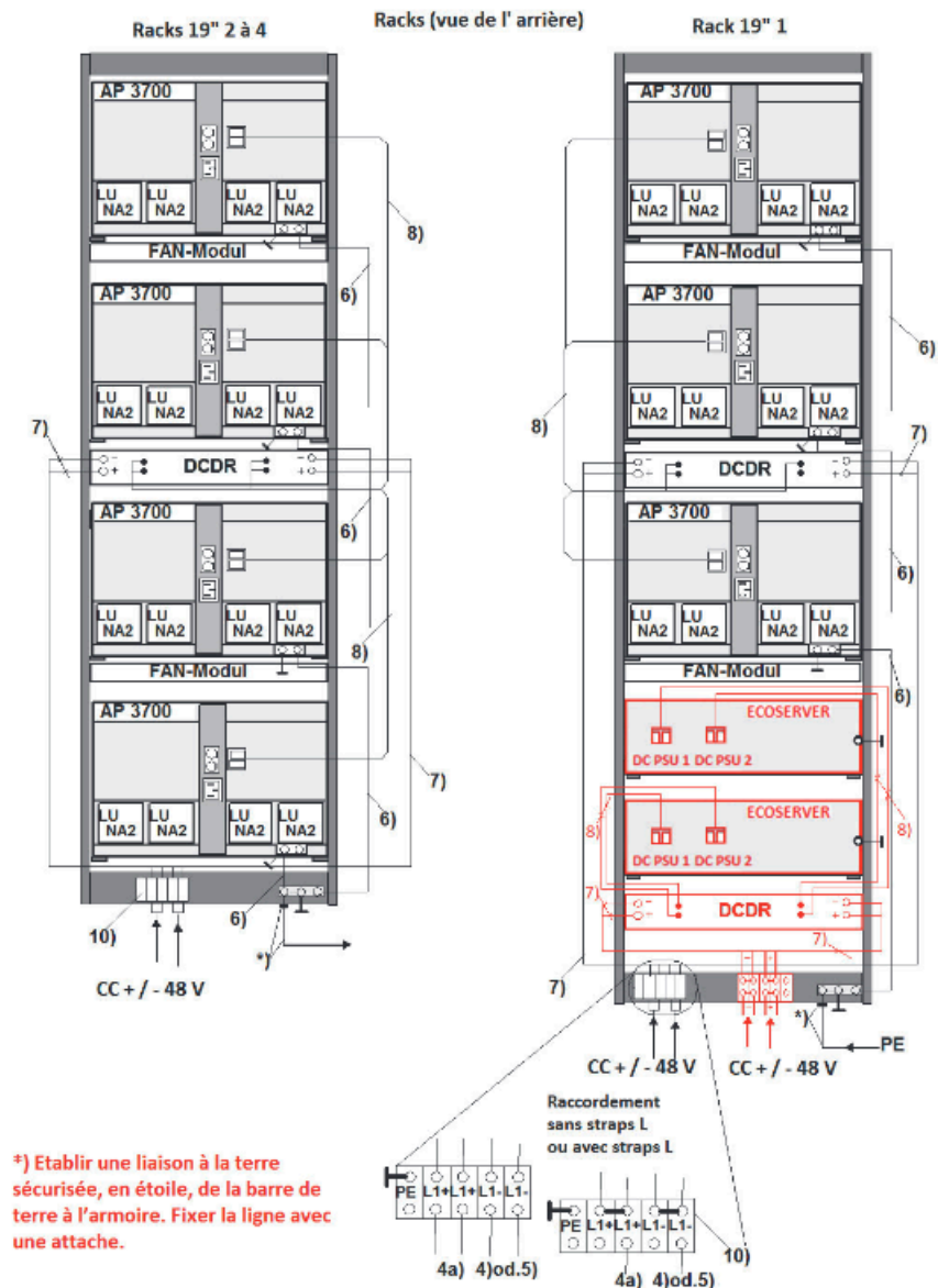
Figure 123: Raccordement CC AP 3700 avec DCDR (unité coupe-circuit)
