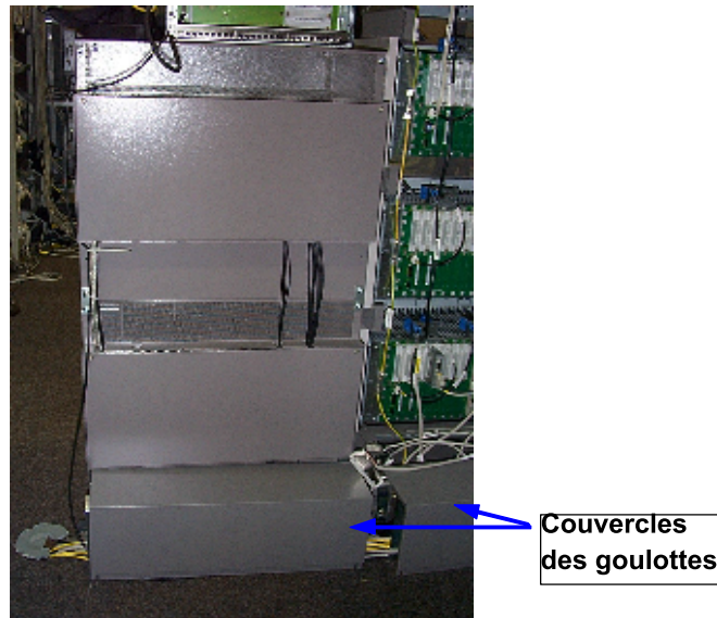
Figure 207: Placer les couvercles des goulottes de câbles
