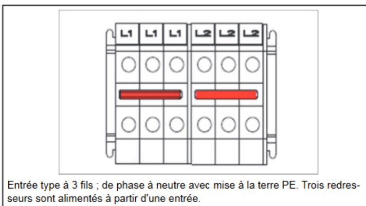
Figure 149: Entrée CA – option 1 (biphasé)
