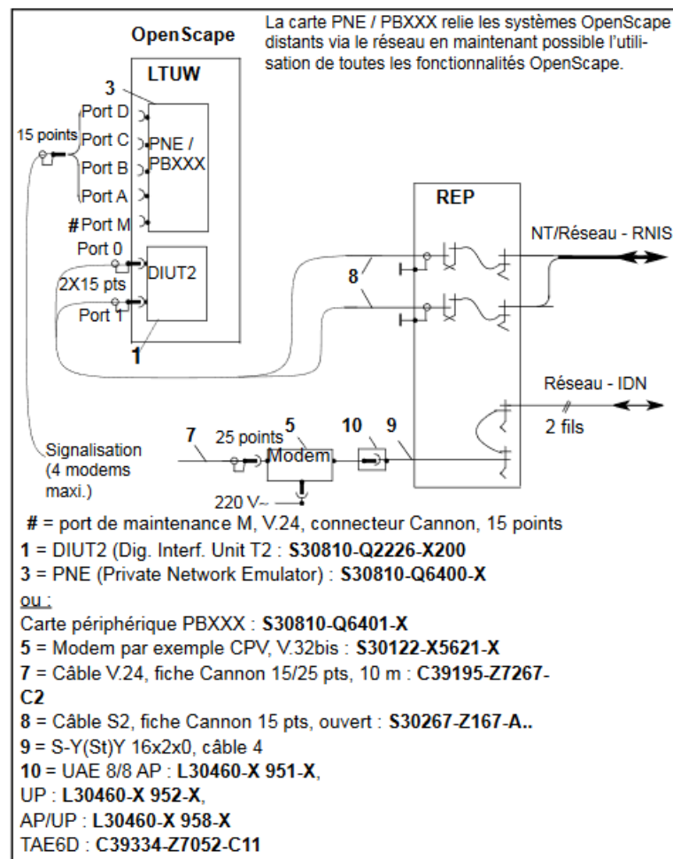
Figure 195: PNE / PBXXX dos à dos avec modem en émulation DIUS2 avec DIUT2
