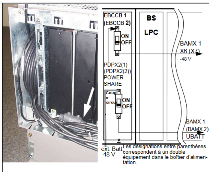
Figure 116: Raccordement de la batterie externe au boîtier d'alimentation (vue de dos)
