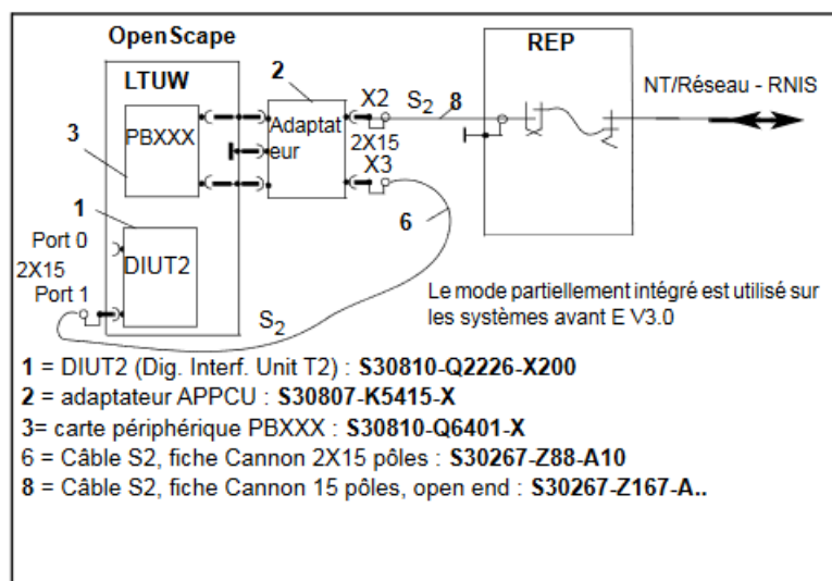
Figure 197: PBXXX avec DIUT2 comme passerelle, partiellement intégré
