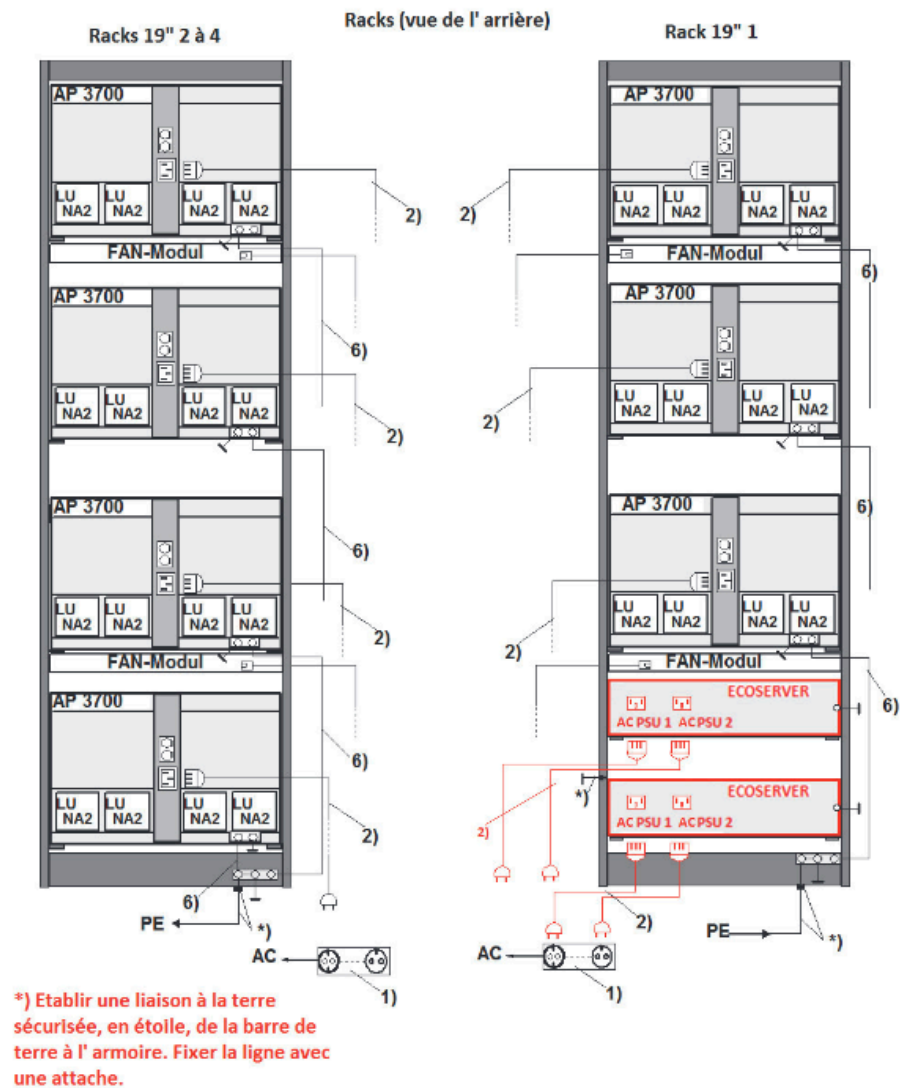
Figure 122: Raccordement CA AP 3700 dans l'armoire 19"
