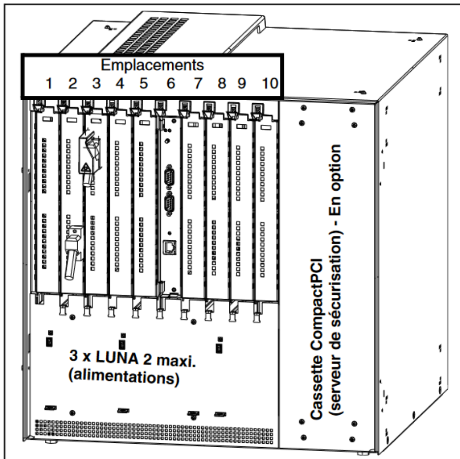
Figure 64: Vue avant AP 3700-9
