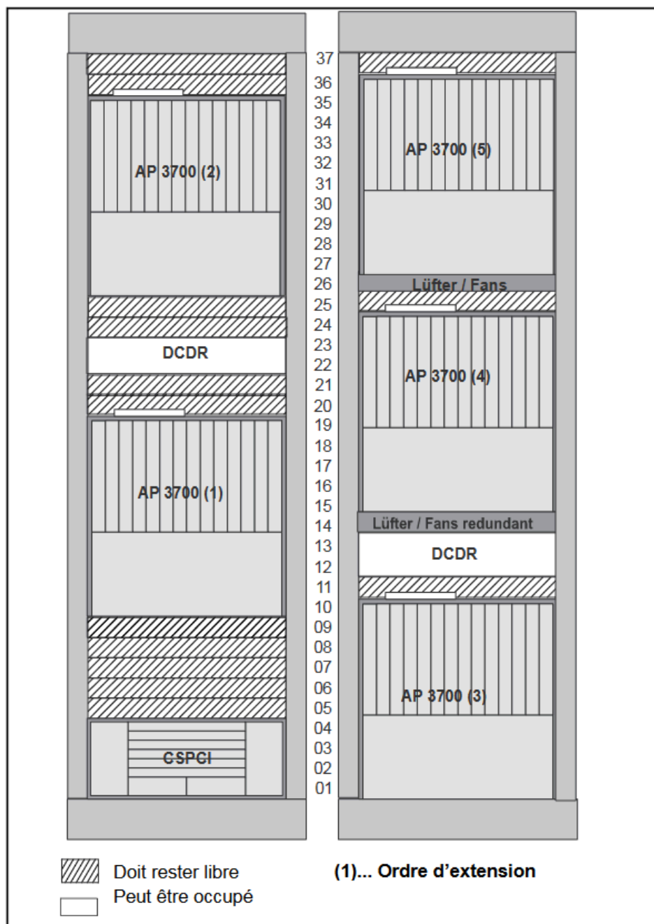
Figure 72: Montage de CSPCI avec AP 3700 dans une armoire de 37 unités
