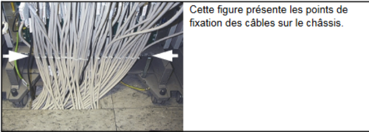
Figure 184: Fixation des câbles sur OpenScape 4000
