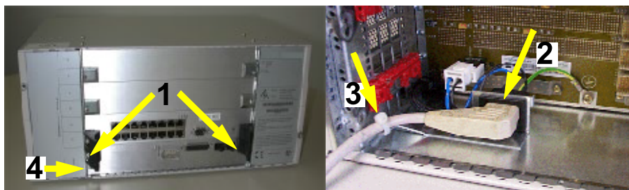
Figure 101: Raccorder le câble d'alimentation au boîtier CSPCI
