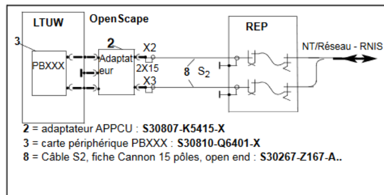
Figure 196: PBXXX comme passerelle, entièrement intégré
