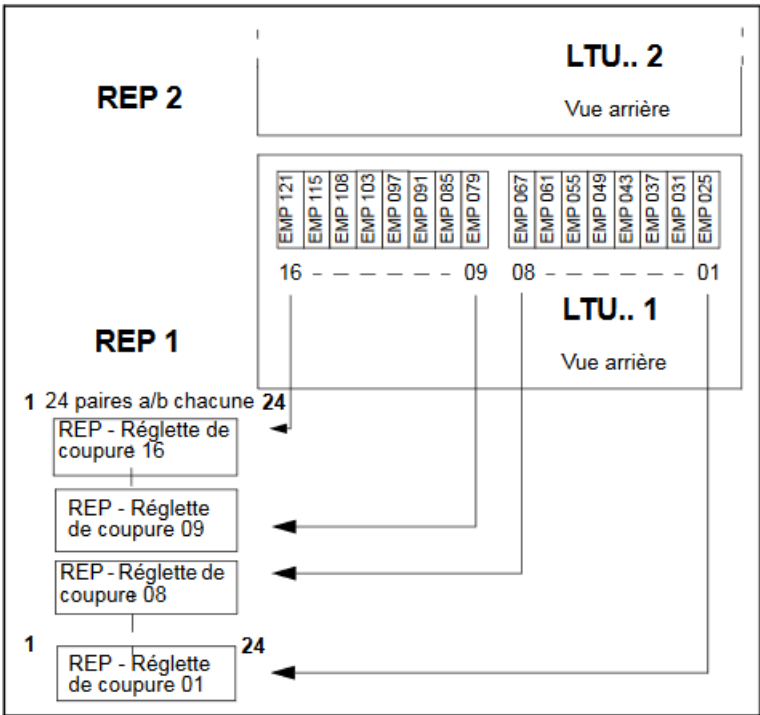
Figure 186: Passage de câble entre LTU et REP
