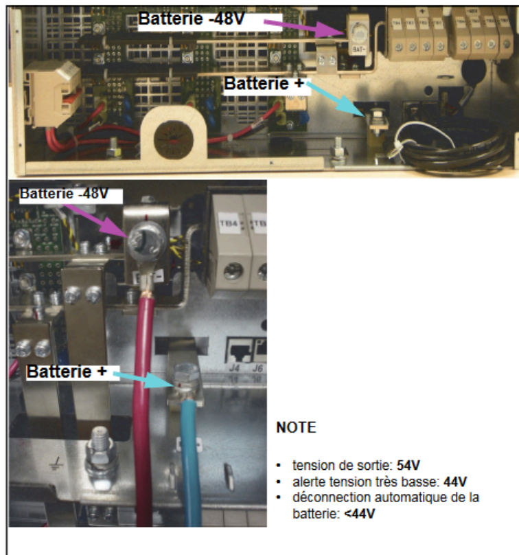
Figure 153: Raccordement de la batterie aux jeux de barres
