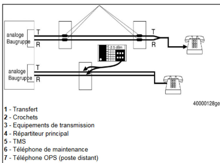
Figure 210: Banc de contrôle pour les mesures ERL/SRL sur lignes OPS
