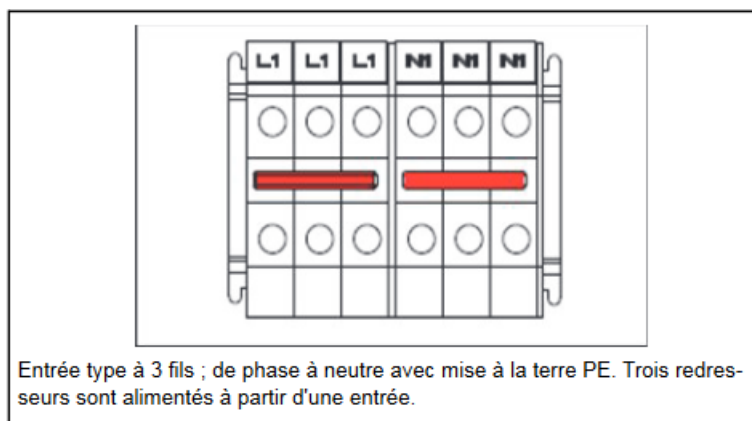
Figure 148: Entrée CA – option 1 (monophasé)
