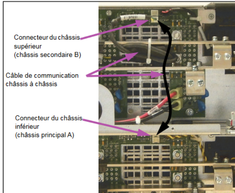
Figure 137: Communication châssis à châssis (vue arrière)
