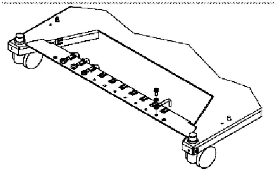
Figure 91: Raccordement à la terre de la barre de terre à la barre 0V dans l'armoire 30"
