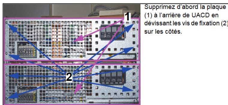
Figure 158: Retrait des caches de l'UACD
