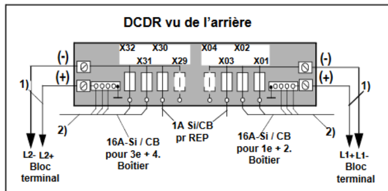
Figure 125: Raccordement DCDR vu de l'arrière
