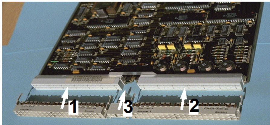
Figure 29: Installation de l'adaptateur SIVAPAC-SIPAC 1 (1 de 2)
