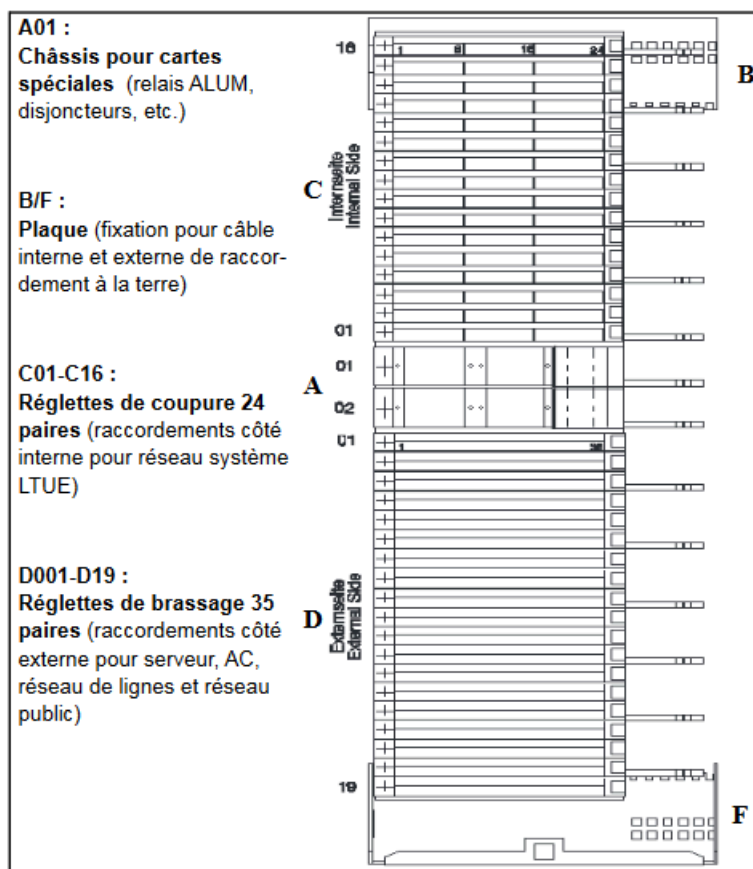
Figure 185: Montage du répartiteur principal MDFHX6
