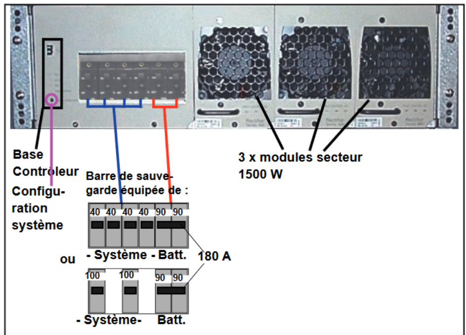
Figure 157: Boîtier de base UACD PSR930 (vue avant)
