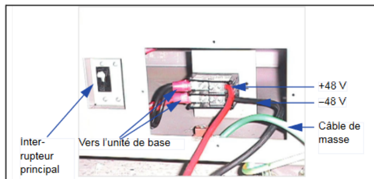
Figure 204: Interrupteur principal du système OpenScape 4000, vue arrière
