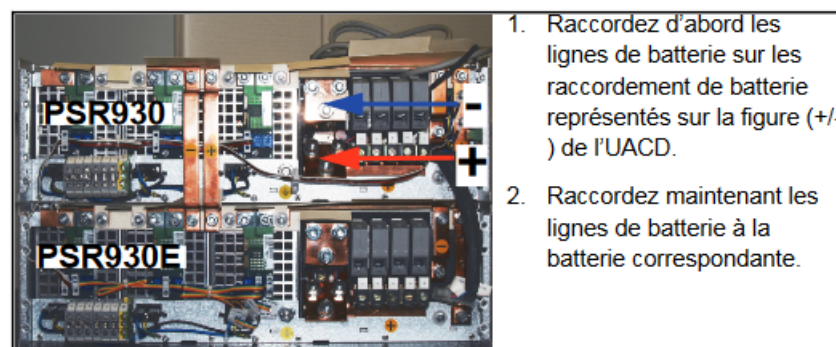
Figure 167: Raccordement de la batterie sur UACD (PSR930/PSR930E)
