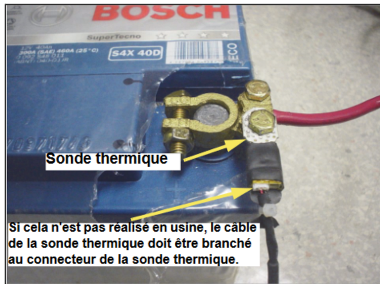
Figure 142: Raccordement de la sonde thermique
