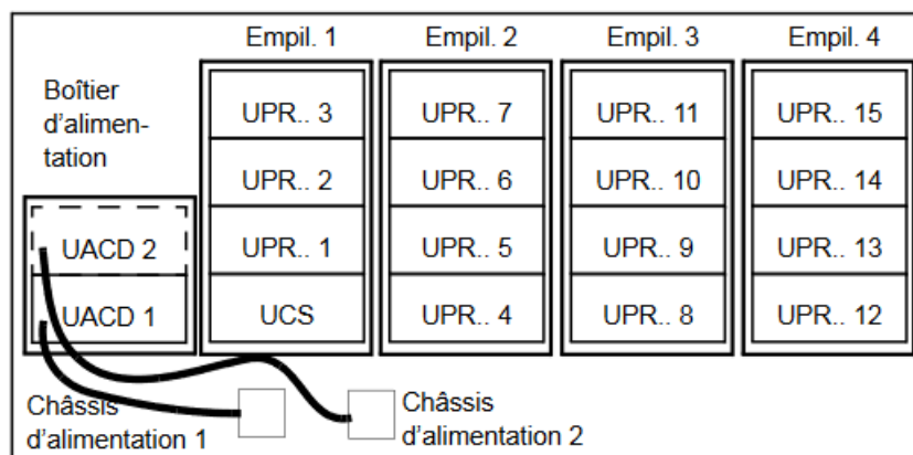
Figure 95: Raccordement au secteur par le boîtier d'alimentation
