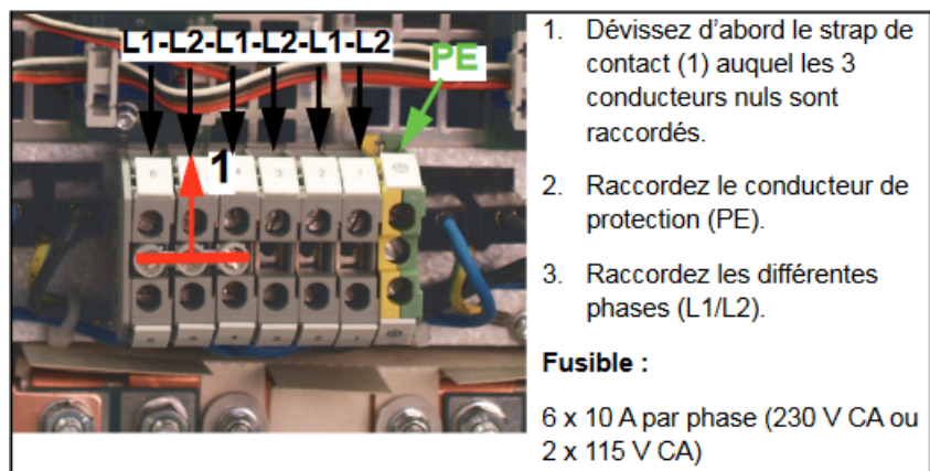
Figure 165: Raccordement à un réseau biphasé (PSR930/PSR930E)
