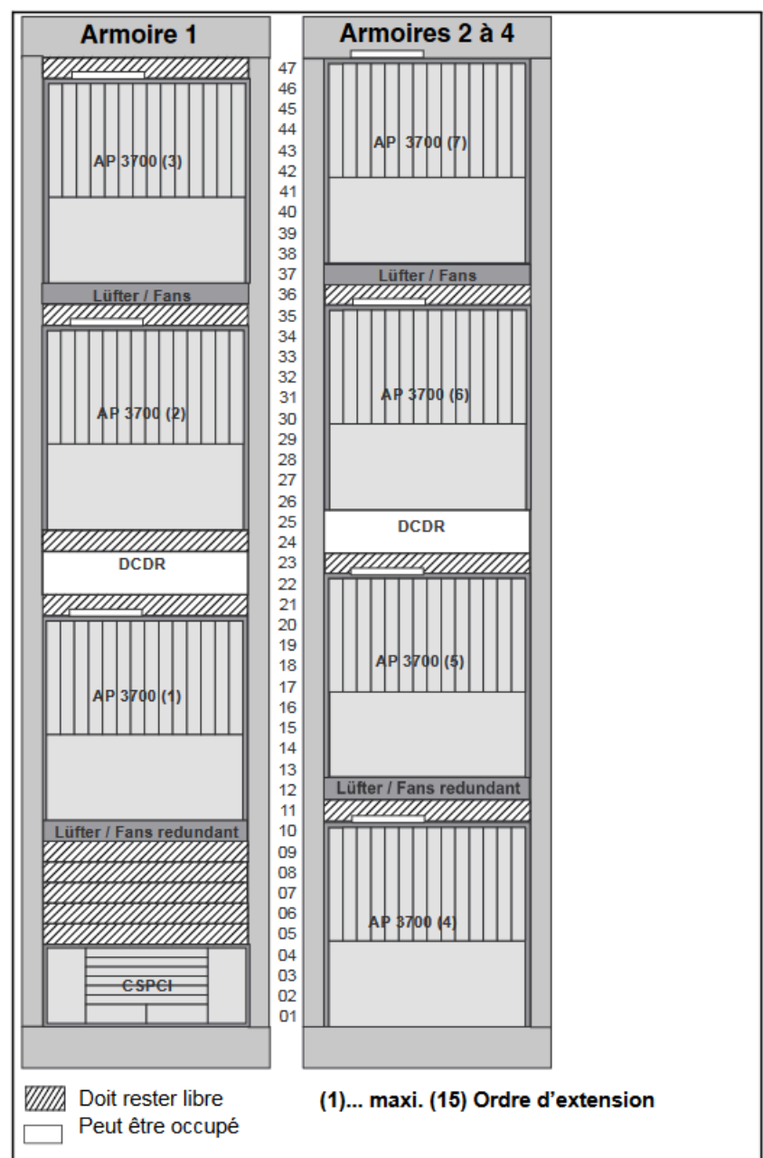
Figure 74: Montage de CSPCI avec AP 3700 dans une armoire de 47 unités
