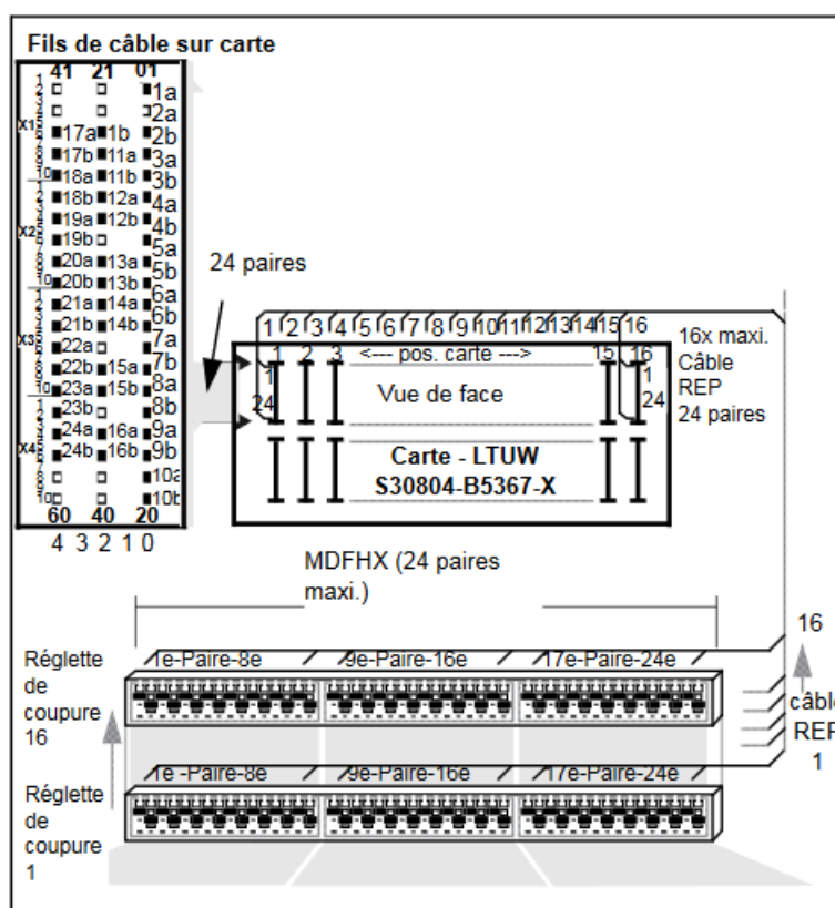
Figure 190: Raccordement de cartes d'abonnés / de joncteurs de lignes
