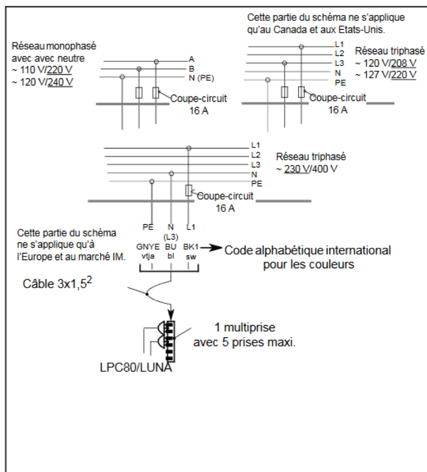
Figure 92: Raccordement au secteur LPC80/LUNA
