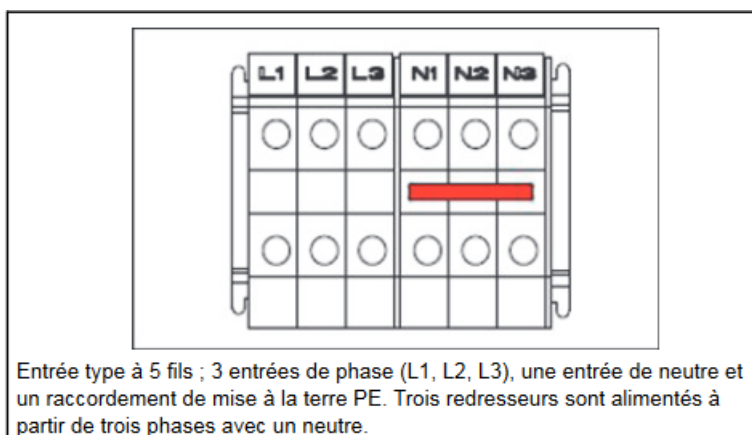
Figure 150: Entrée CA – option 2 (raccordement triphasé en étoile)
