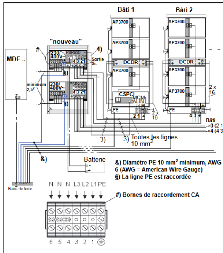
Figure 160: Raccordement CA/CC avec UACD (PSR930/PSR930E) dans l'armoire 19" avec AP3700
