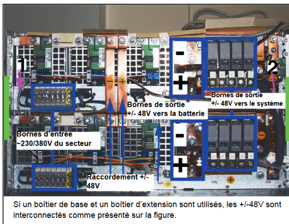
Figure 159: Boîtier d'alimentation UACD PSR930/PSR930E (vue arrière)
