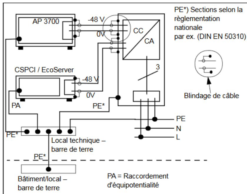
Figure 89: Configuration de terre pour raccordement CA autonome
