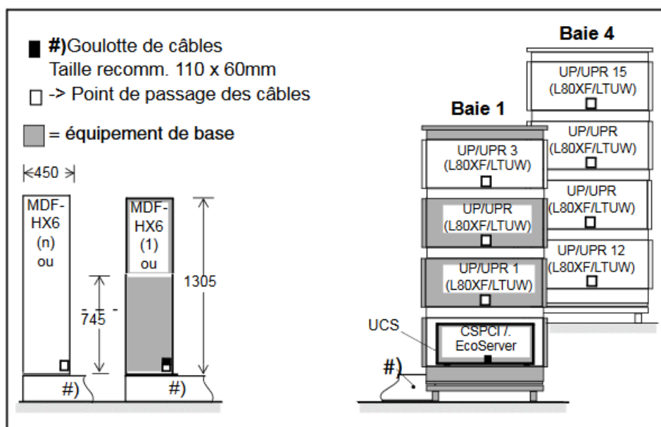
Figure 52: Boîtier CSCI dans le châssis UCS, baie 1
