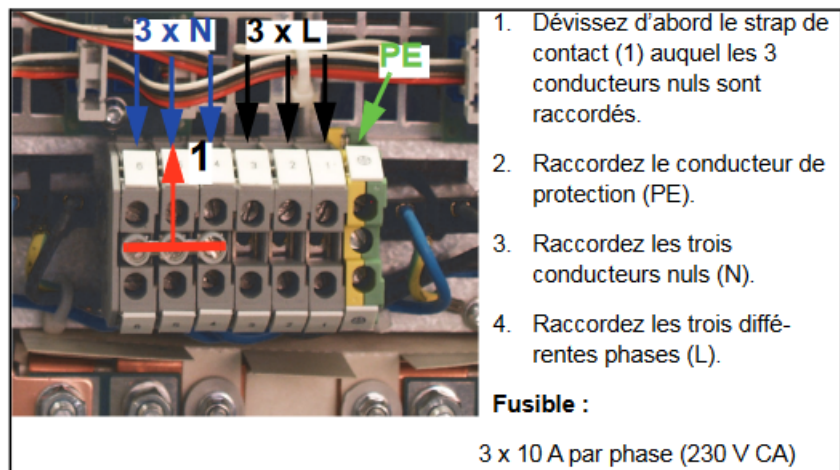
Figure 164: Raccordement à un réseau monophasé (PSR930/PSR930E)
