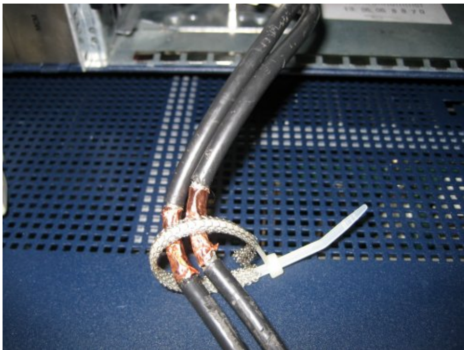
Figure 40: Attache de câble avec gaine en métal
