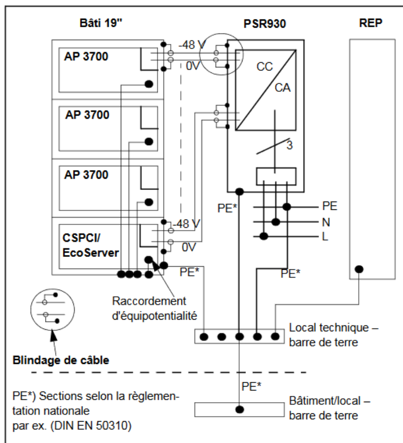
Figure 85: Configuration de terre pour le raccordement CC 19"
