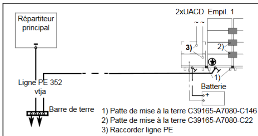
Figure 90: Schéma de mise à la terre du système OpenScape 4000
