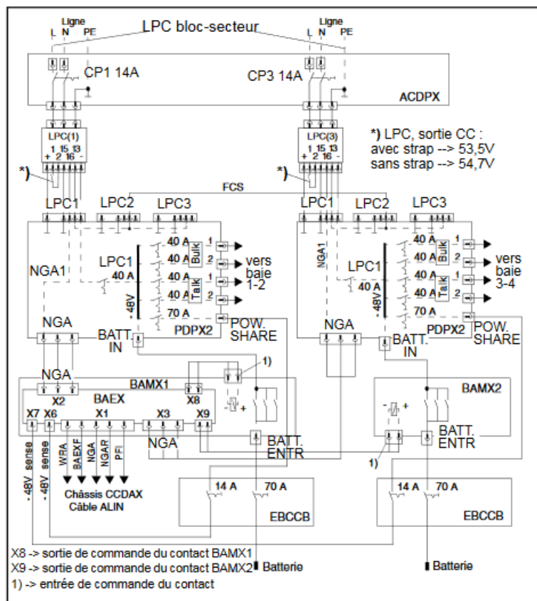
Figure 172: Gestionnaire de batterie, vue d'ensemble des raccordements
