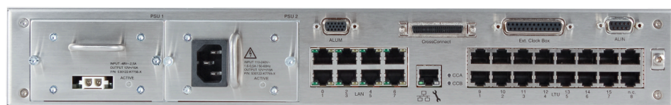
Figure 3: Vue arrière de l'OpenScape 4000 EcoServer
