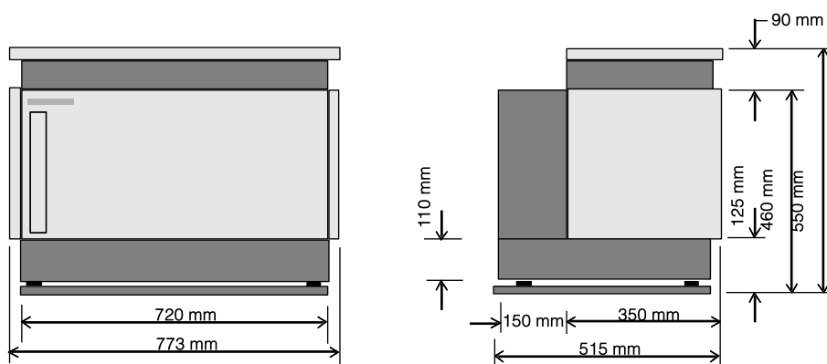
Figure 48: Système à un boîtier
