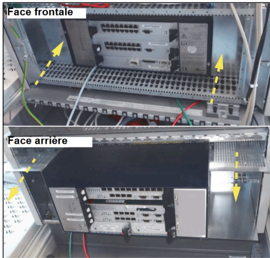
Figure 32: Retrait par l'avant du châssis CSPCI
