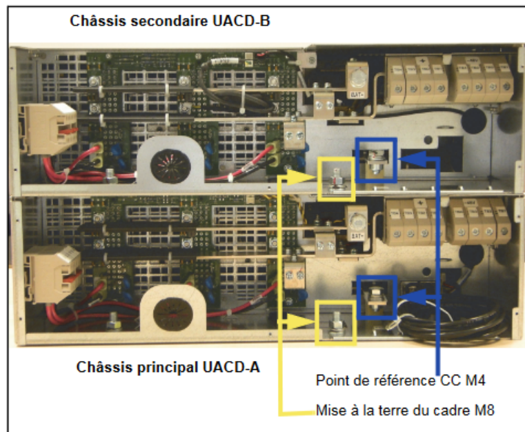
Figure 133: Point de référence CC et mise à la terre du cadre
