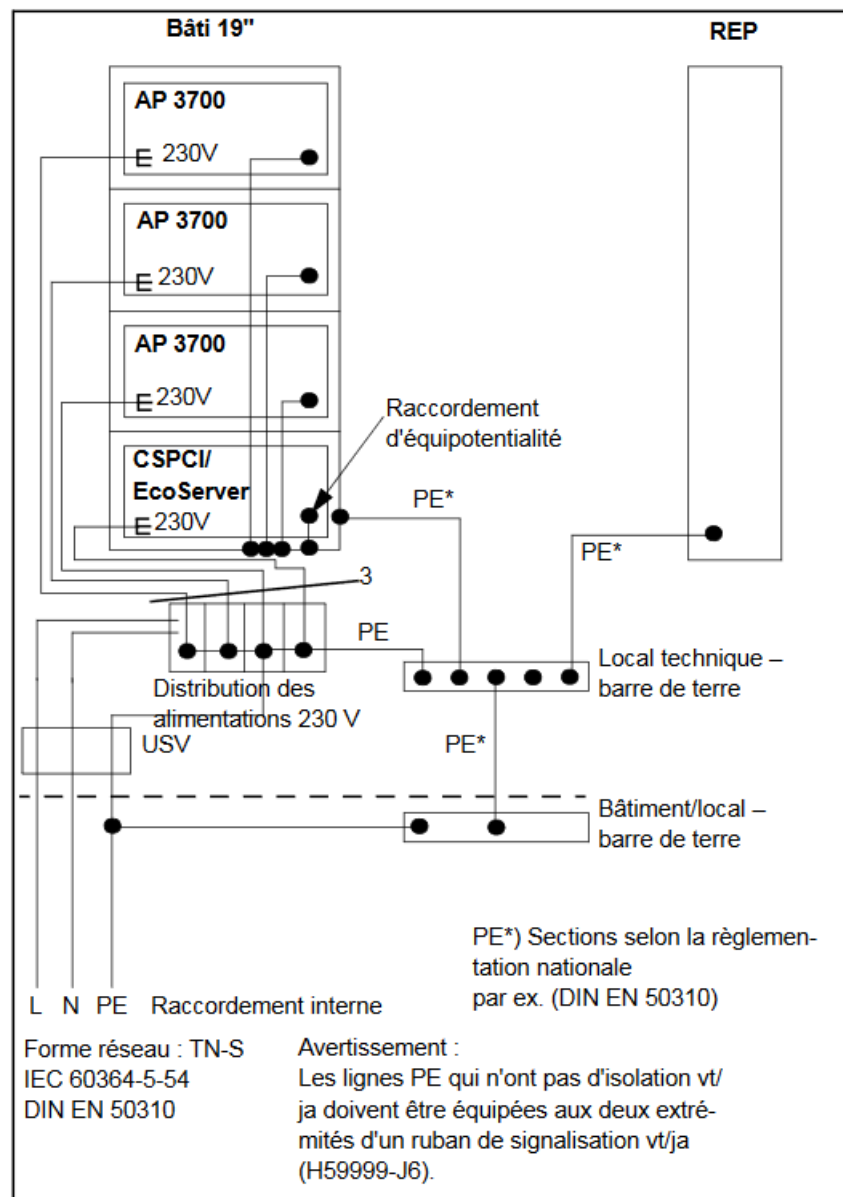
Figure 84: Configuration de terre pour le raccordement CA 19"
