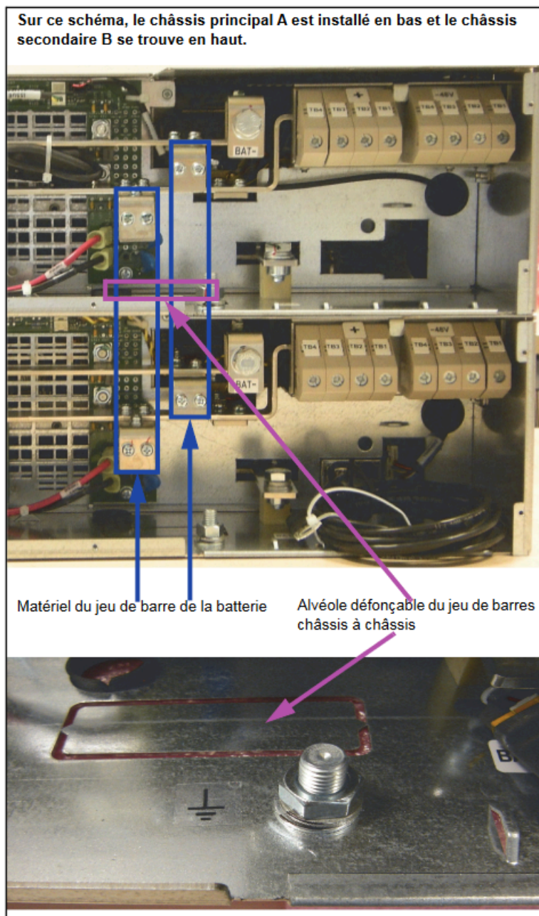
Figure 135: Montage des jeux de barres châssis à châssis
