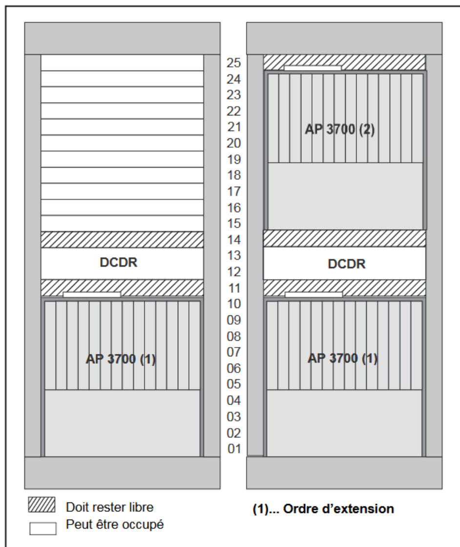
Figure 71: Montage de AP 3700/AP 3700 IP dans une armoire de 25 unités
