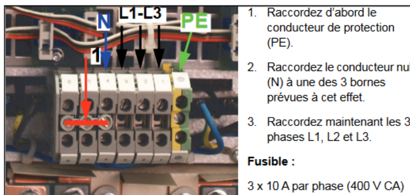
Figure 163: Exemple de raccordement sur un réseau triphasé (PSR930/PSR930E)
