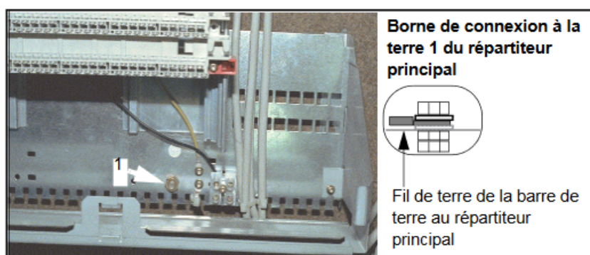
Figure 77: Mise à la terre du système OpenScape 4000
