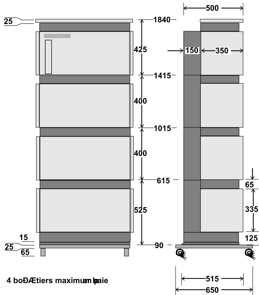
Figure 49: Système à plusieurs boîtiers
