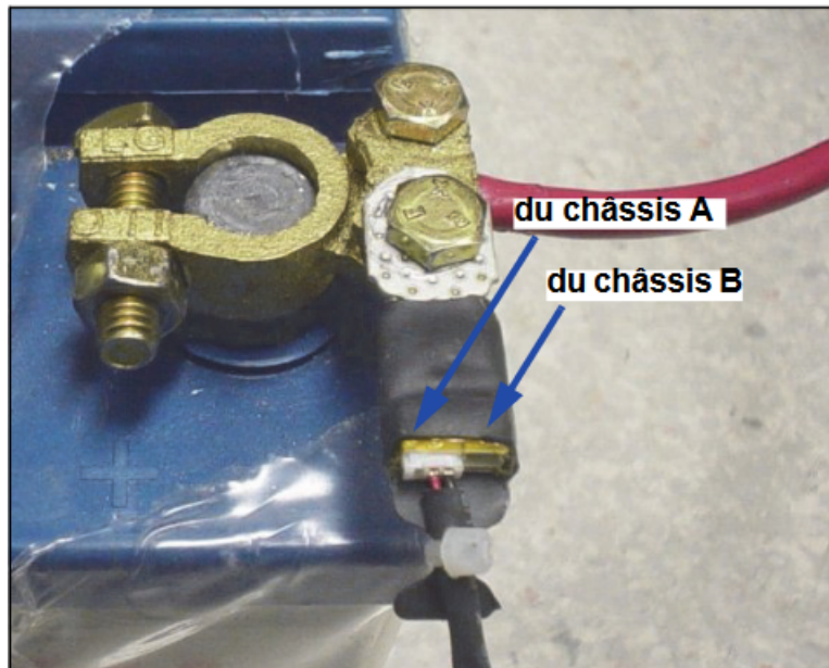
Figure 144: Raccordement de la sonde thermique à la batterie
