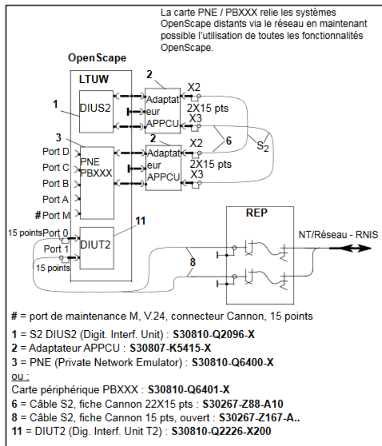
Figure 194: PNE / PBXXX dos à dos sans modem et avec DIUT2
