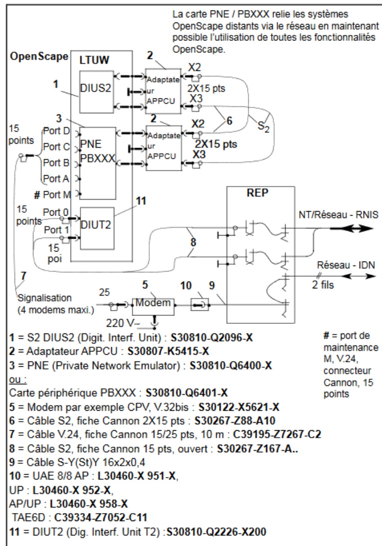
Figure 193: PNE / PBXXX dos à dos avec modem et DIUT2
