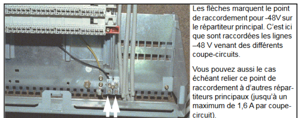
Figure 118: Carte coupe-circuit -48 V pour REP (non redondant)
