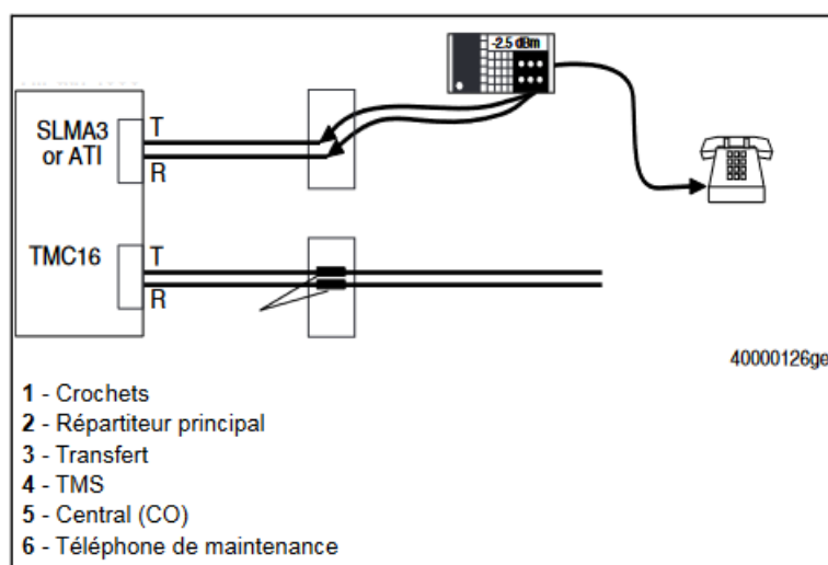
Figure 208: Banc de contrôle pour les mesures ERL/SRL sur les canaux de commutation.
