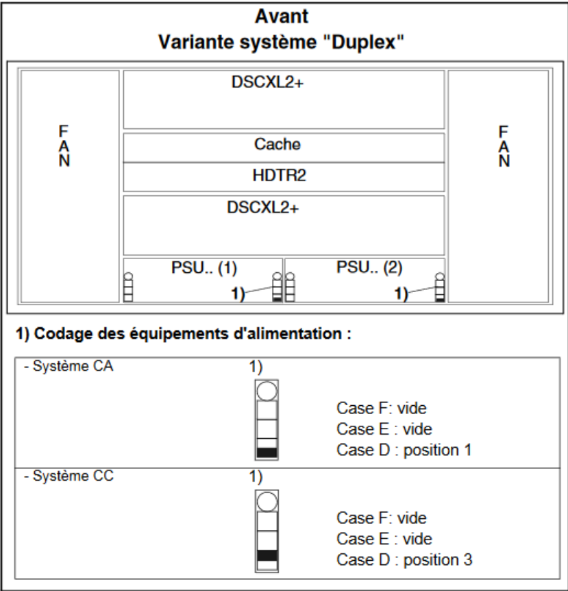
Figure 108: Codage pour variantes d'alimentation ACPCI/DCPCI
