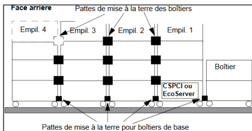
Figure 78: Pattes de mise à la terre OpenScape 4000 (armoires 30")
