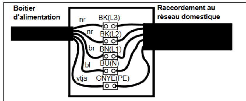
Figure 97: Câblage de la boîte de distribution UACD
