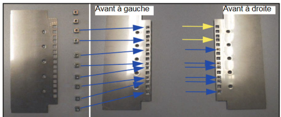
Figure 18: Prémontage des supports en tôle frontaux
