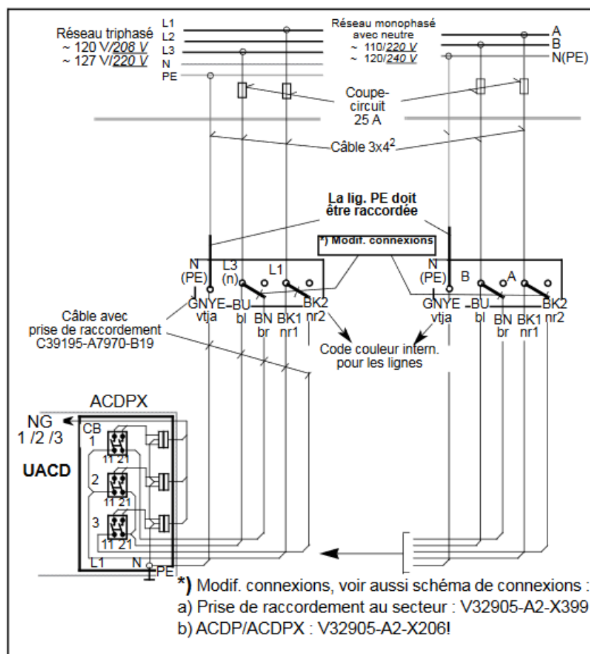
Figure 99: Réseau triphasé/monophasé avec neutre
