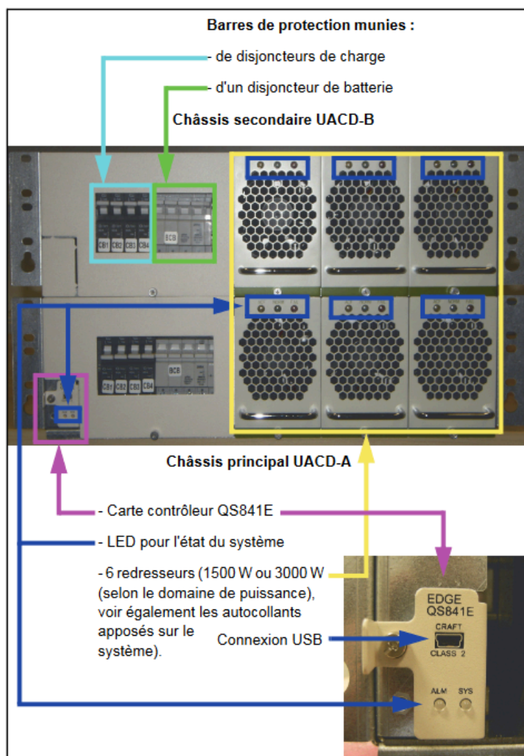
Figure 129: UACD-A&B – Vue avant (détails)
