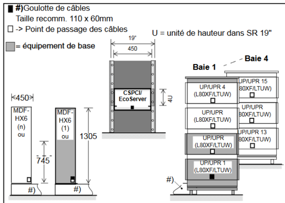
Figure 53: Boîtier CPCI dans l'armoire 19" externe
