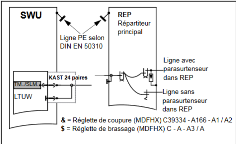
Figure 188: Installation d'une protection primaire supplémentaire
