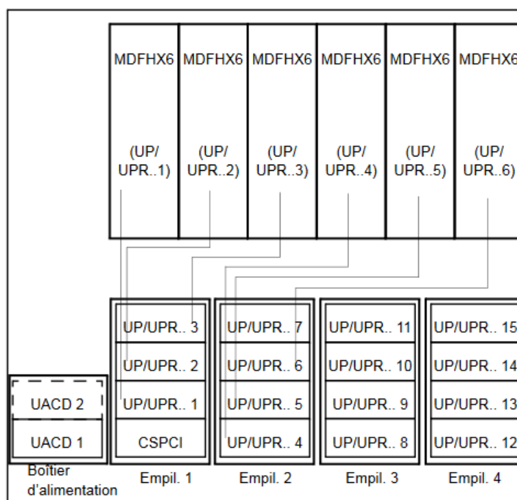
Figure 211: Configuration étendue du OpenScape 4000 avec un nombre maximum de MDFHX6
