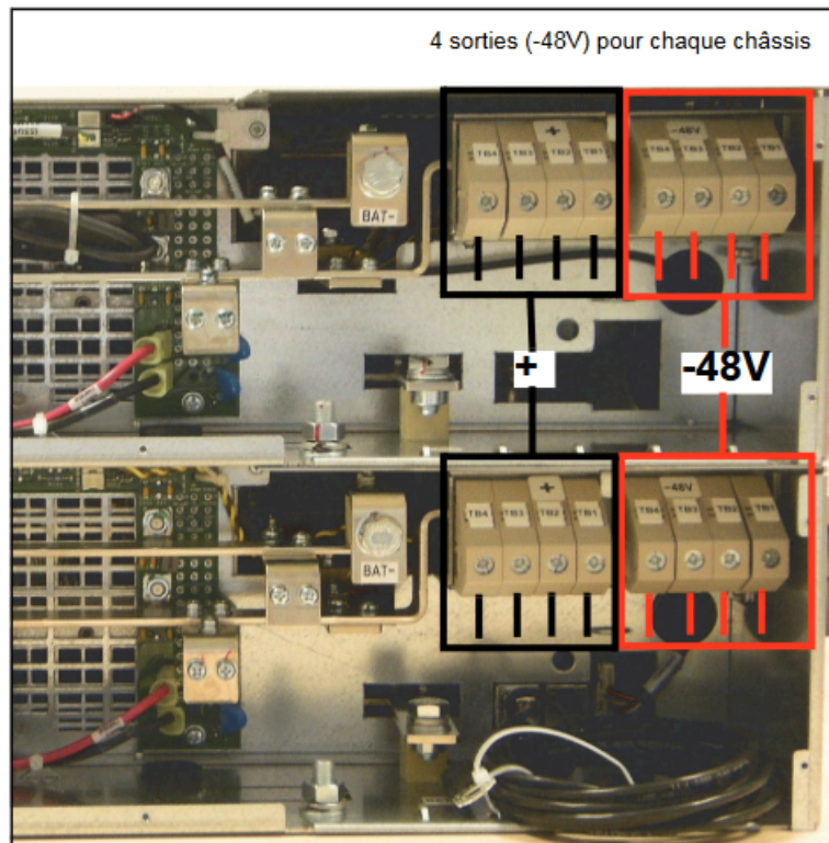
Figure 138: Bornes de sortie de l'UACD (vue arrière)
