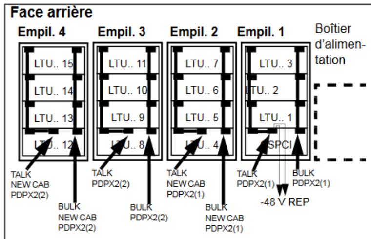
Figure 176: Liaisons -48 V redondantes entre PDPX2 et châssis
