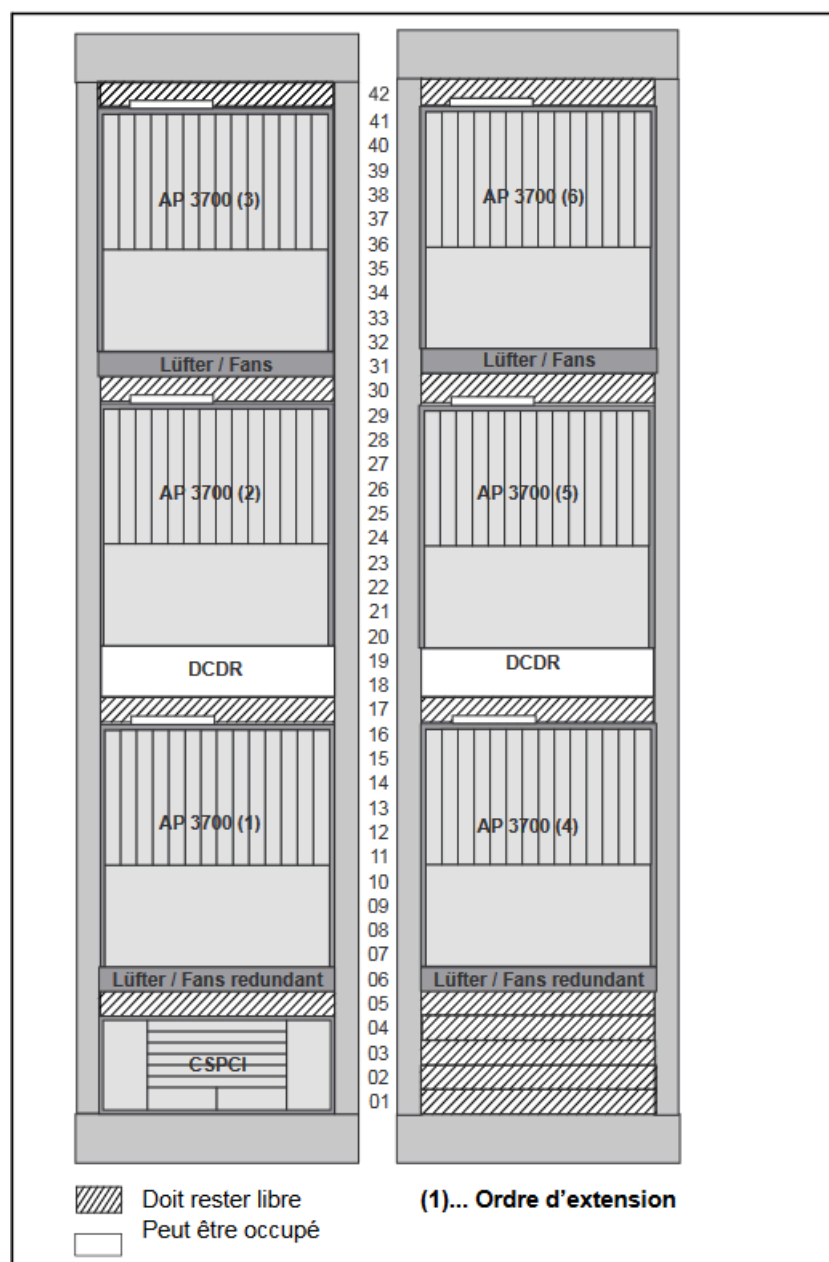
Figure 73: Montage de CSPCI avec AP 3700 dans une armoire de 42 unités
