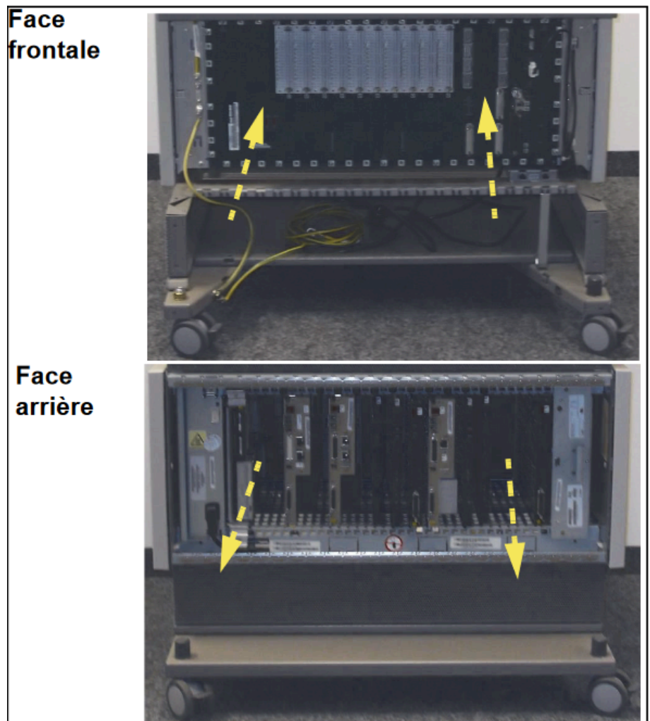
Figure 34: Retrait par l'avant du châssis CCDAX
