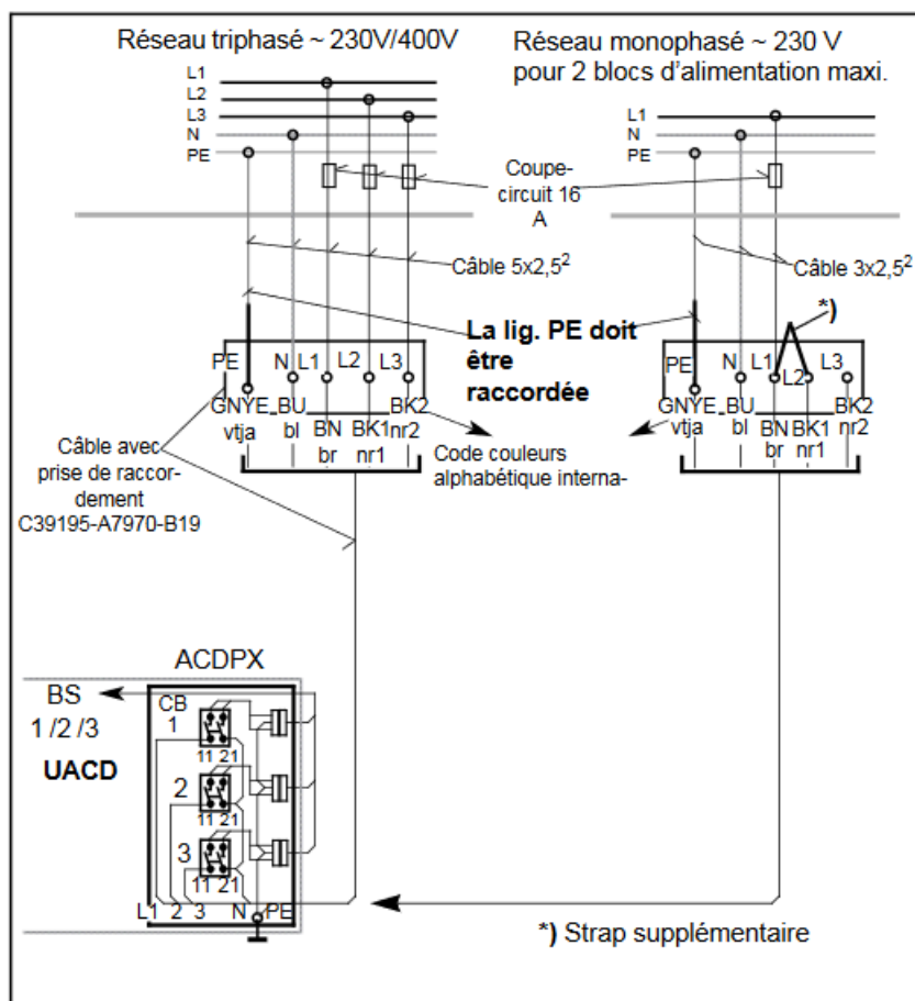
Figure 98: Raccordement au réseau triphasé/monophasé pour deux blocs d'alimentation
