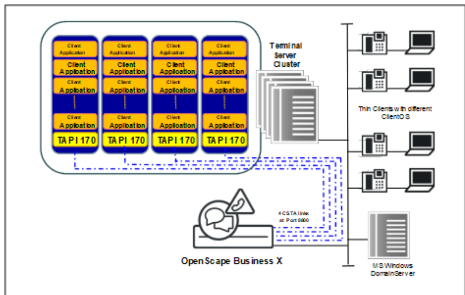
Abbildung 13: Client basierte TAPI Applikation auf Terminal-Server an OpenScape Business
