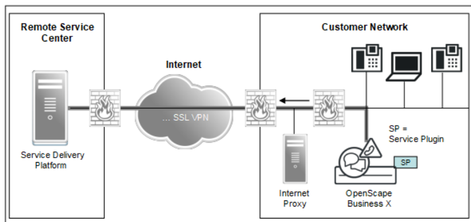
Abbildung 15: RSP - Übersicht für OpenScape Business X
