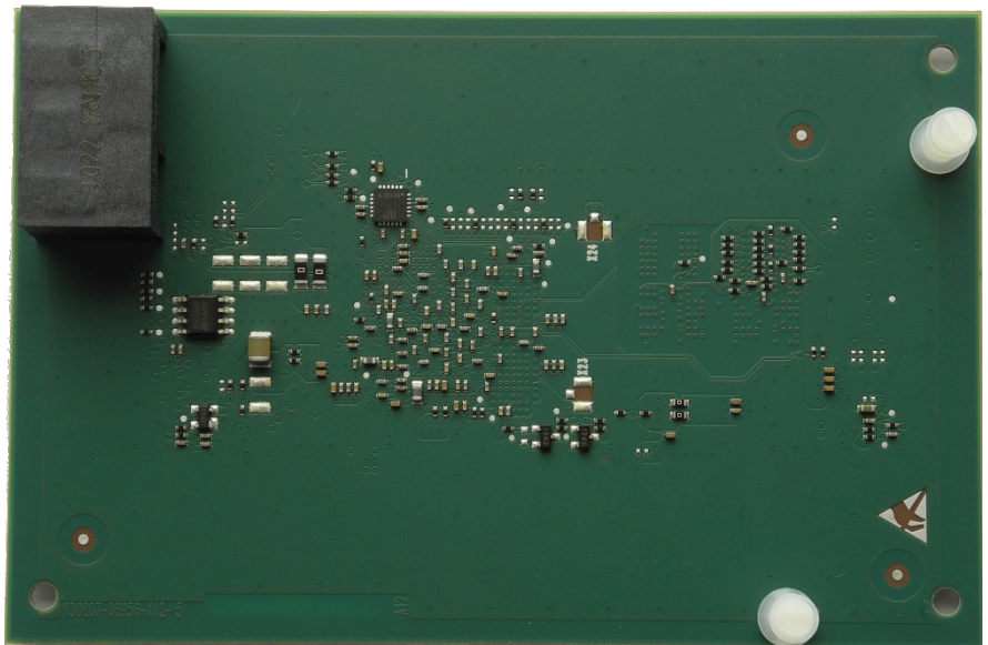
Figura 17: Exemplo OCCBL - Parte traseira com parafusos de espaçamento inseridos
