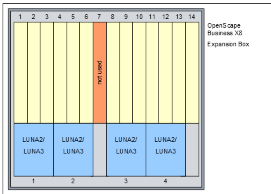
Abbildung 17: OpenScape Business X8 – Baugruppen-Steckplätze in der Erweiterungsbox
