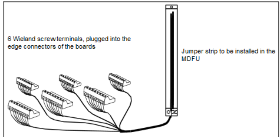
Abbildung 26: CABLU S30269-Z41-A30
