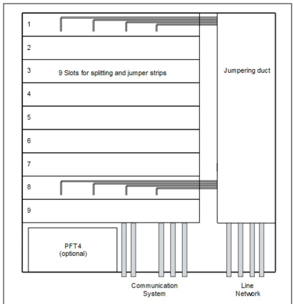
Abbildung 24: Hauptverteiler MDFU
