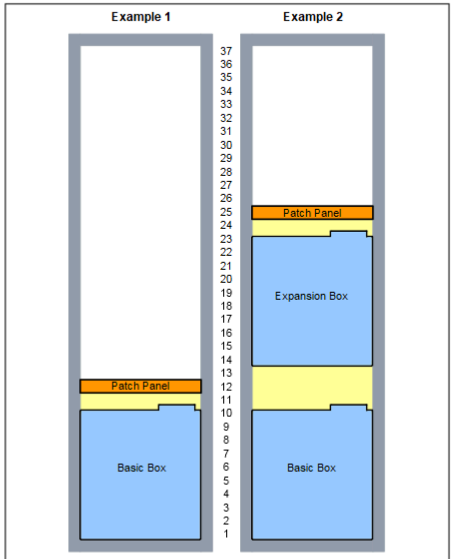
Abbildung 1: OpenScape Business X8 – Beispiele für eine 19"-Schrankschöhe von 1,92 m (37 Höheneinheiten)
