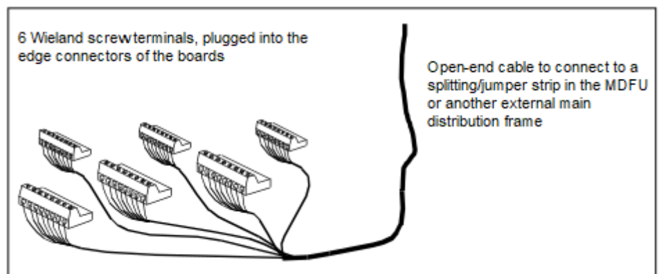
Abbildung 27: Open-End-Kabel S30267-Z322-Axxx
