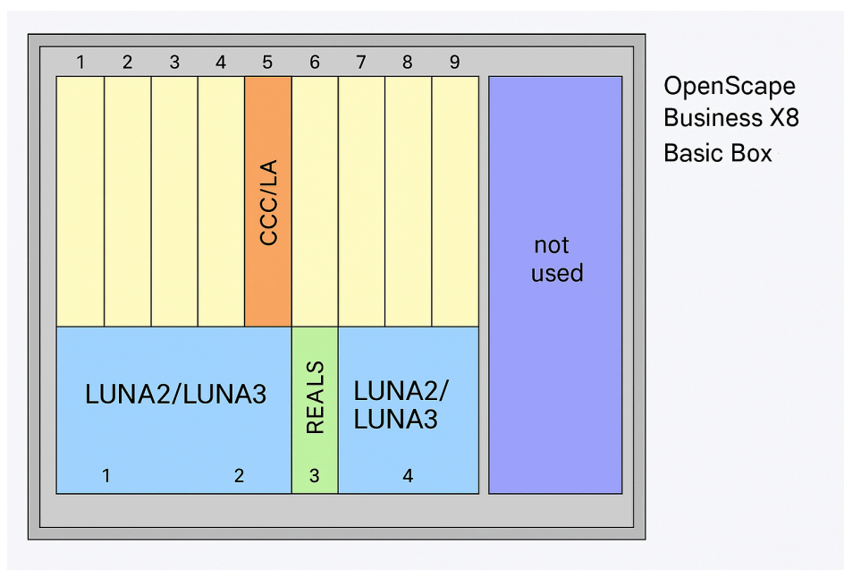
Abbildung 16: OpenScape Business X8 – Baugruppensteckplätze in der Basisbox
