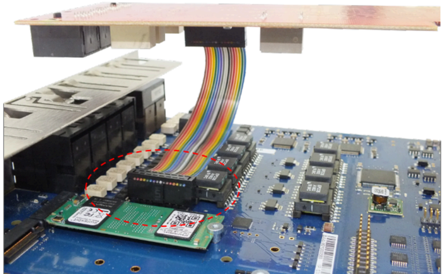
Abbildung 59: Position des an das Mainboard OCCMAR oder OCCMBR angeschlossenen Verbindungskabels
