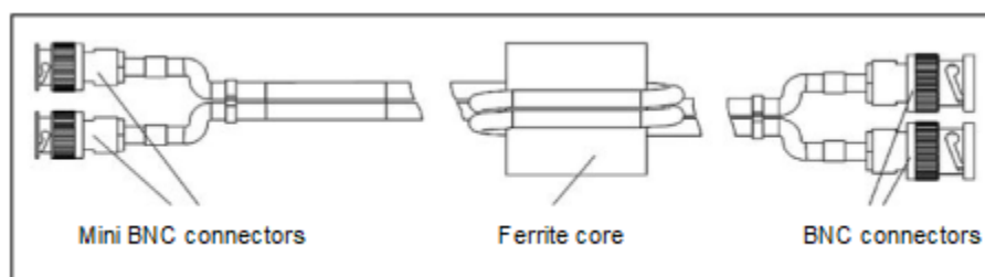
Abbildung 63: TCASR-2 – CAS-Kabel C39195-A7700-B13
