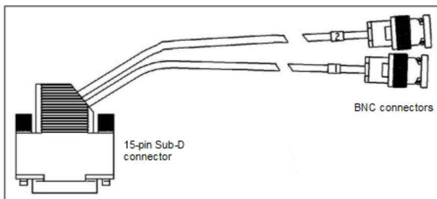
Abbildung 70: TMCAS2 – CAS-Kabel C39195-A7700-B14
