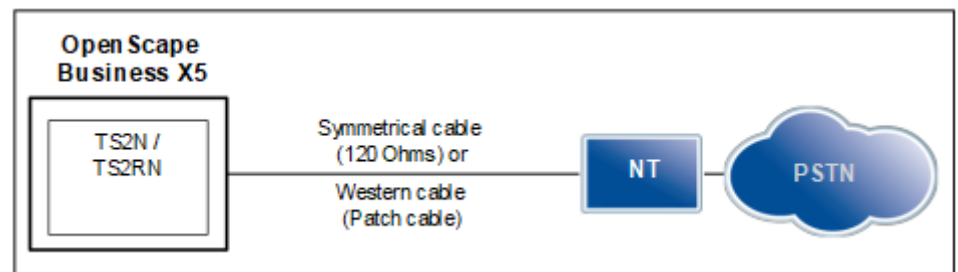
Abbildung 79: TS2N, TS2RN – ISDN-Amtsanschluss
