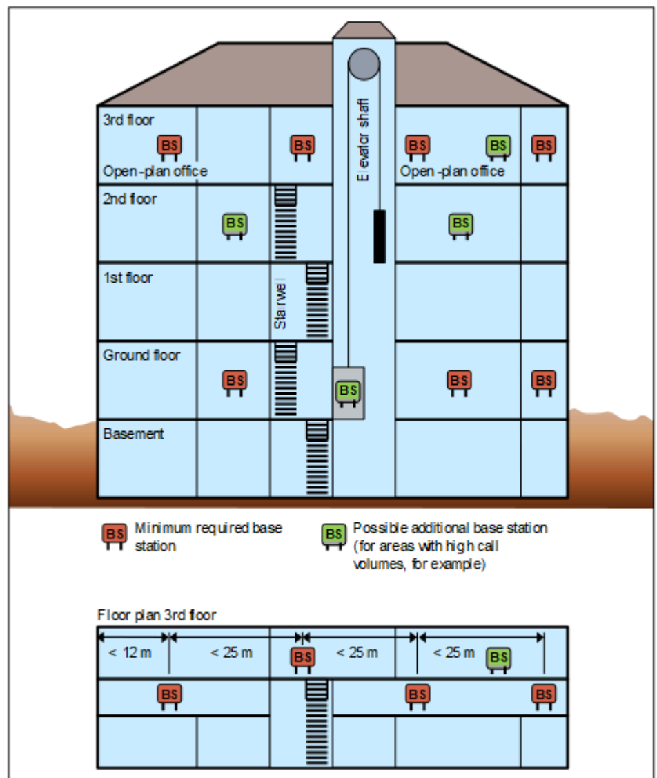
Abbildung 89: Beispiel für die Positionierung von Basisstationen in Stahlbetongebäuden mit Beton- und Stahltrennwänden
