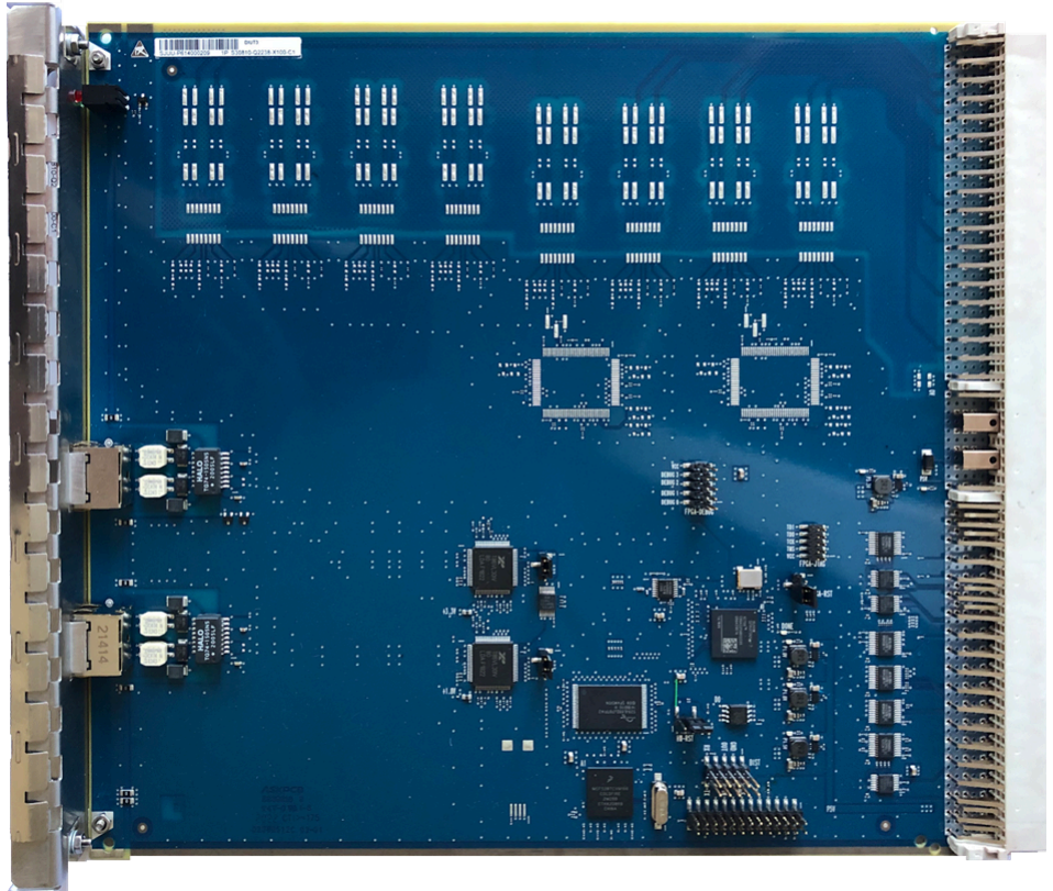
Abbildung 11: DIUT3-Baugruppe
