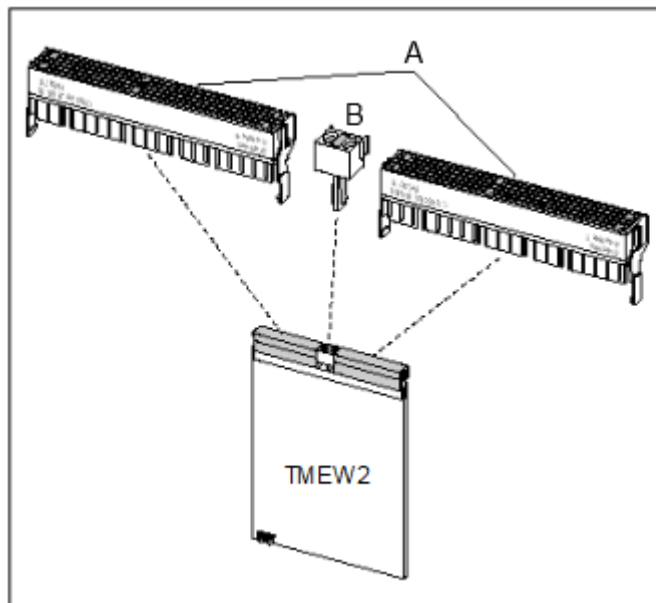
Abbildung 75: SIVAPAC-SIPAC-Baugruppenadapter
