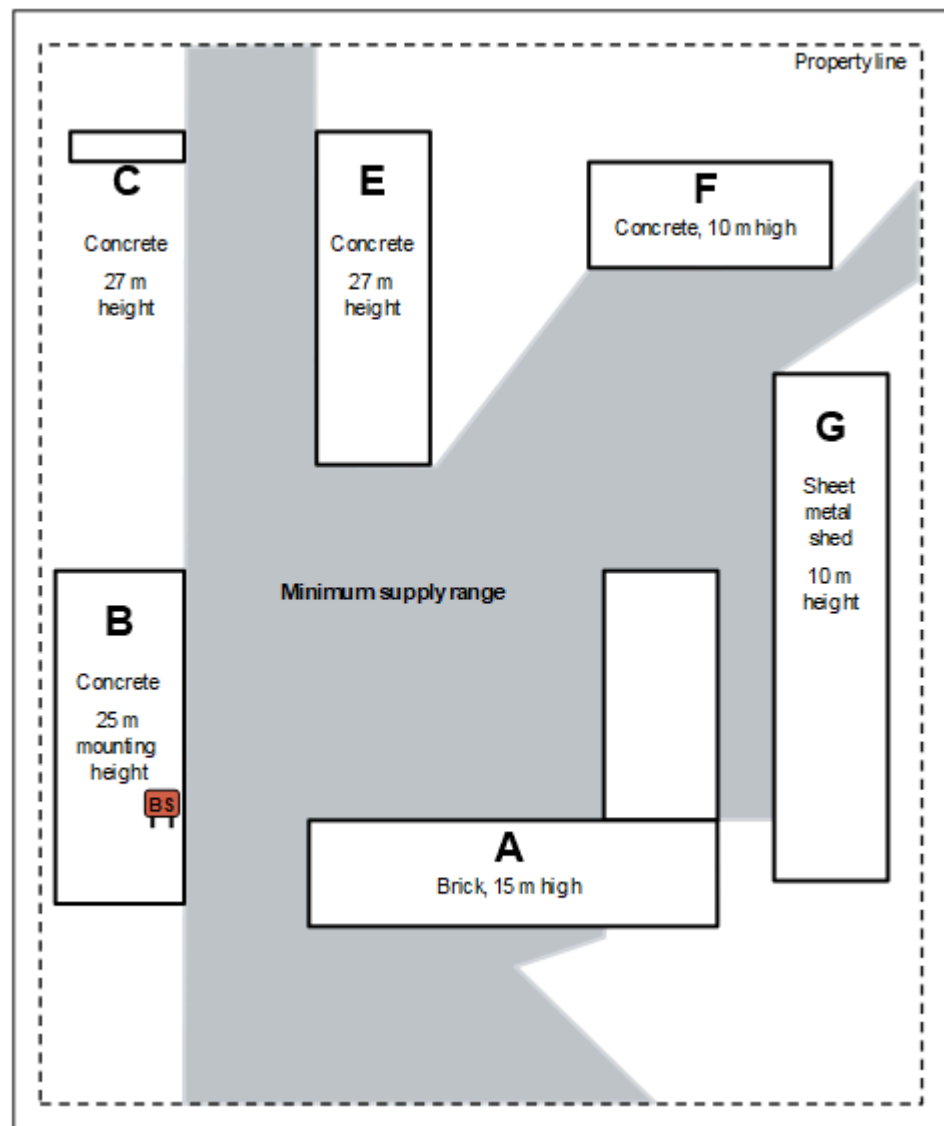
Abbildung 91: Beispiel für die Positionierung einer Basisstation zur Funkabdeckung eines Werksgeländes
