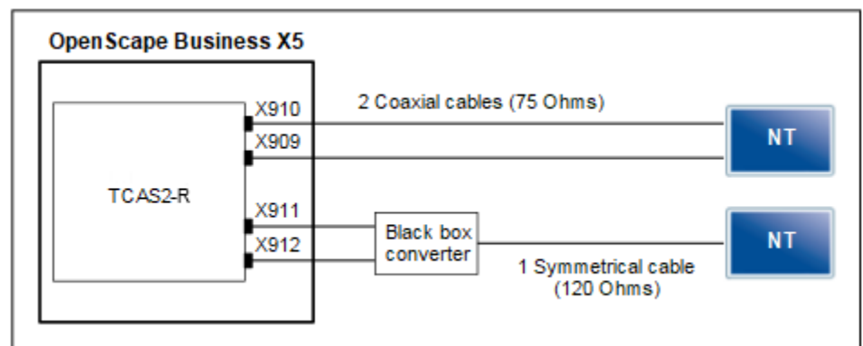
Abbildung 62: TCAS-2, TCASR-2 – Möglichkeiten für die Verbindung zum Network Terminator NT
