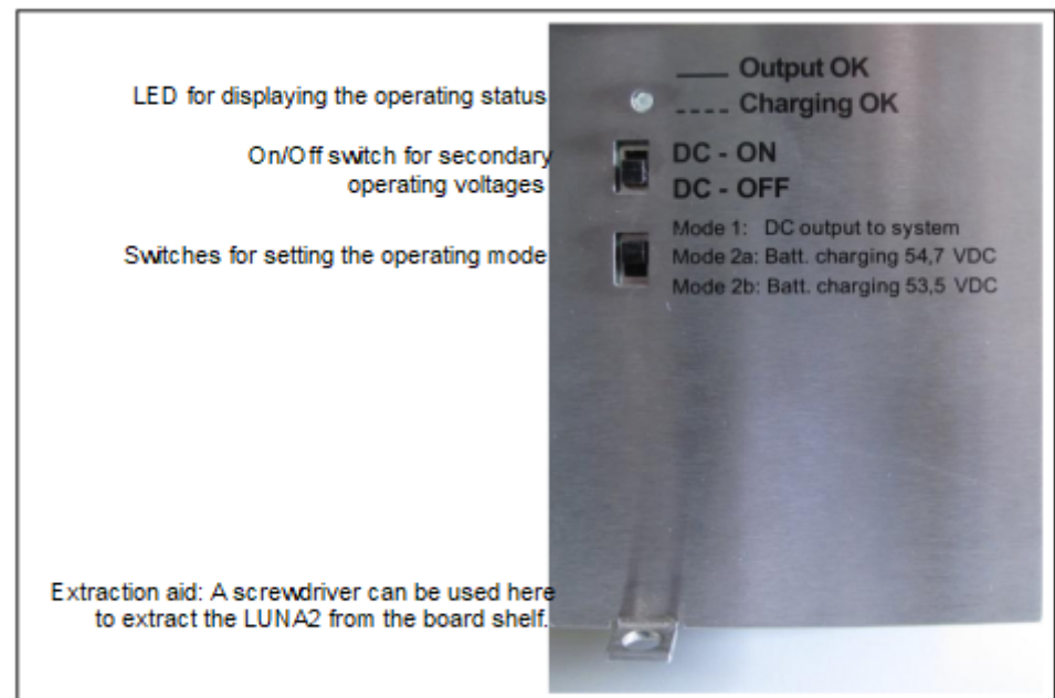
Abbildung 17: LUNA2 – Frontblende
