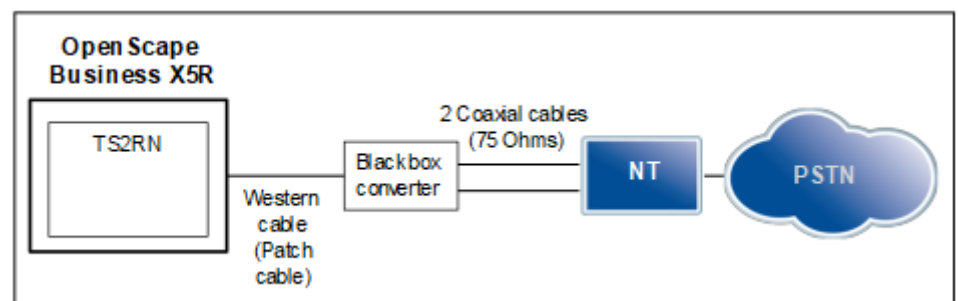
Abbildung 80: TS2RN – ISDN-Amtsanschluss für Portugal und Spanien
