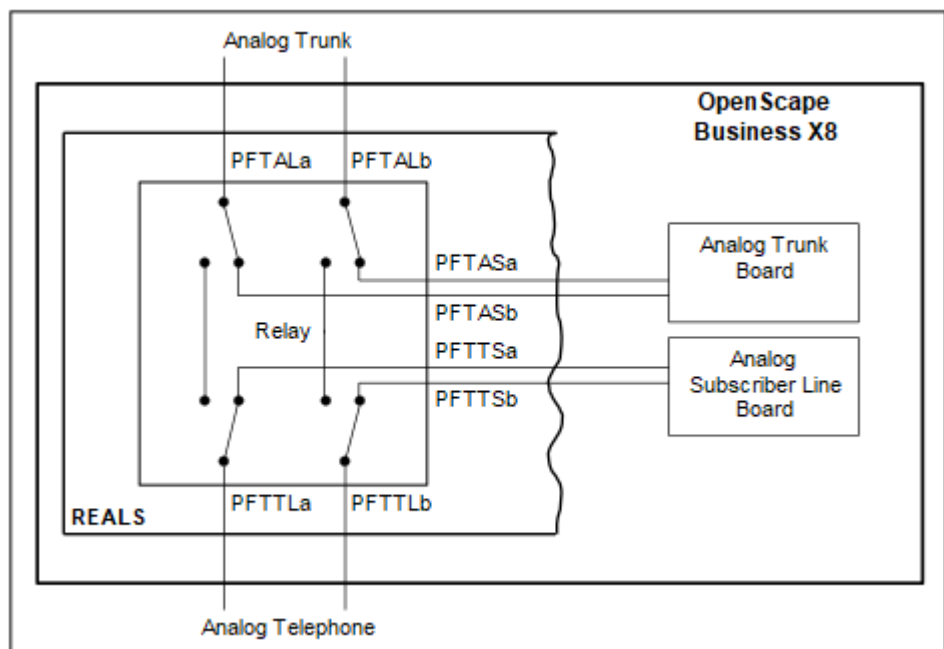
Abbildung 35: REALS – Prinzipschaltbild (Kommunikationssystem im Normalbetrieb)
