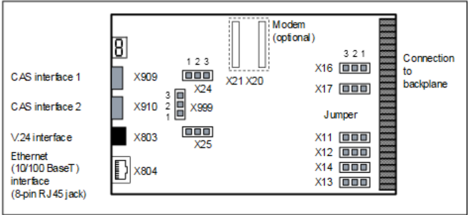
Abbildung 69: TMCAS2
