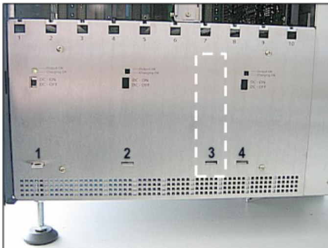
Abbildung 36: REALS – Steckplatz 3 in der Basisbox
