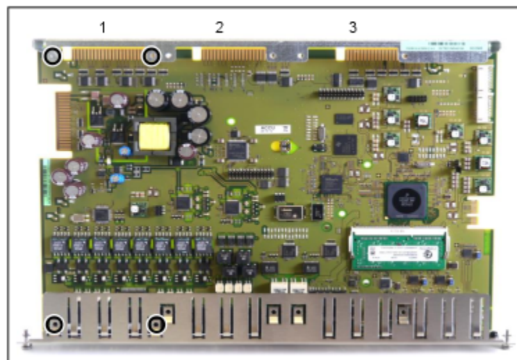
Abbildung 51: OCCMR – Position der Befestigungsschrauben für STRBR
