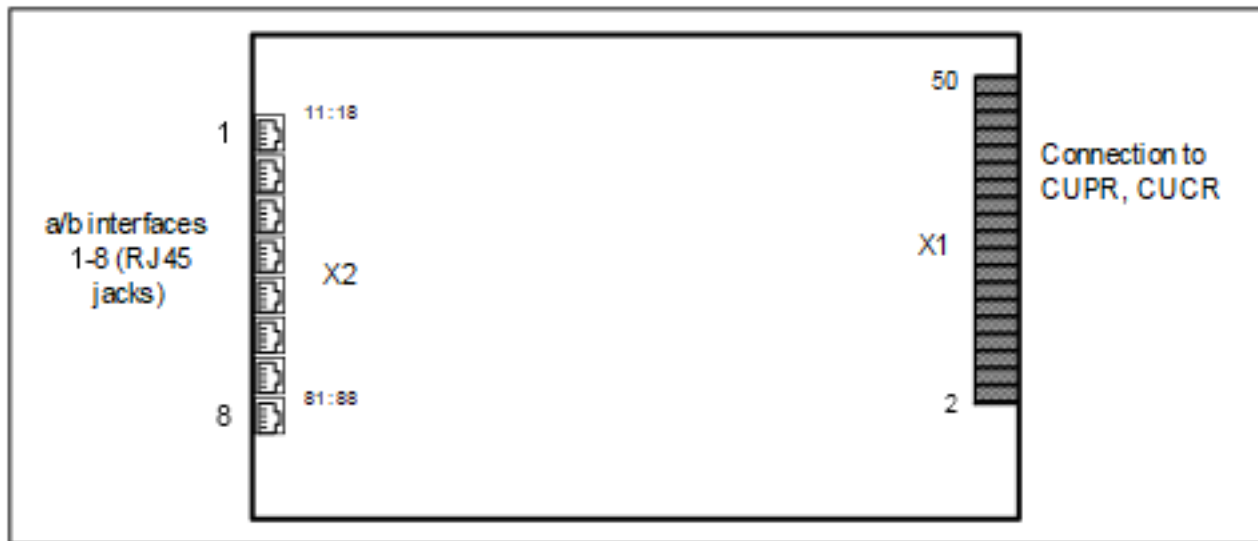
Abbildung 37: SLAV8R
