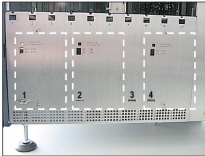
Abbildung 19: LUNA2 – Steckplätze 1, 2 und 4 in der Basisbox
