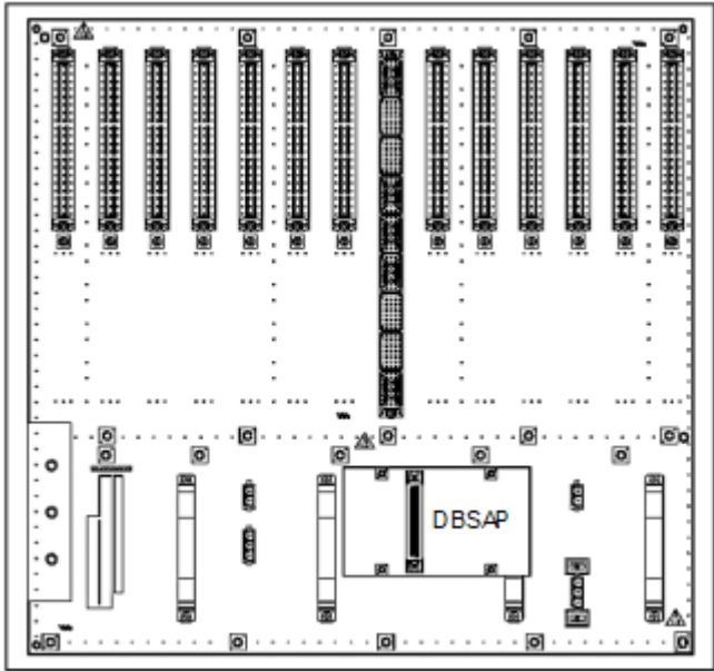
Abbildung 9: DBSAP – Montage auf der Backplane der Erweiterungsbox
