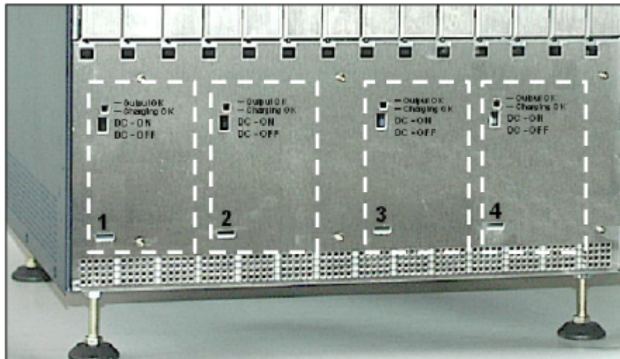
Abbildung 20: LUNA2 – Steckplätze 1, 2, und 4 in der Erweiterungsbox
