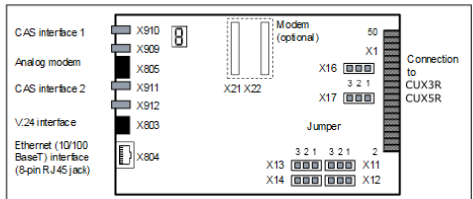
Abbildung 61: TCASR-2 – Anschlüsse und Jumper
