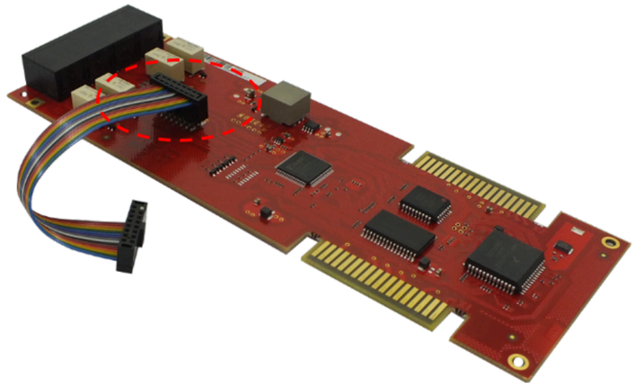
Abbildung 58: STRBR mit gestecktem Kabel
