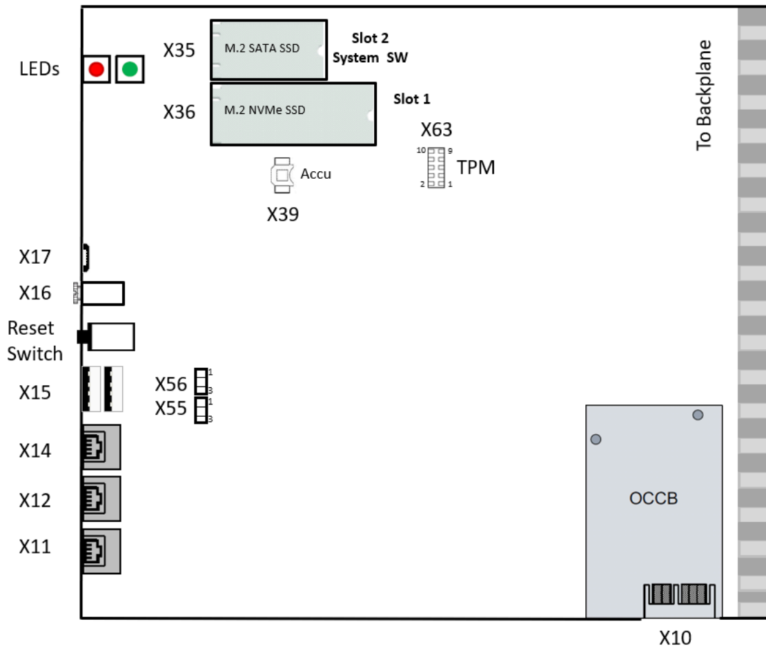
Abbildung 28: OCCLA Anschlüsse
