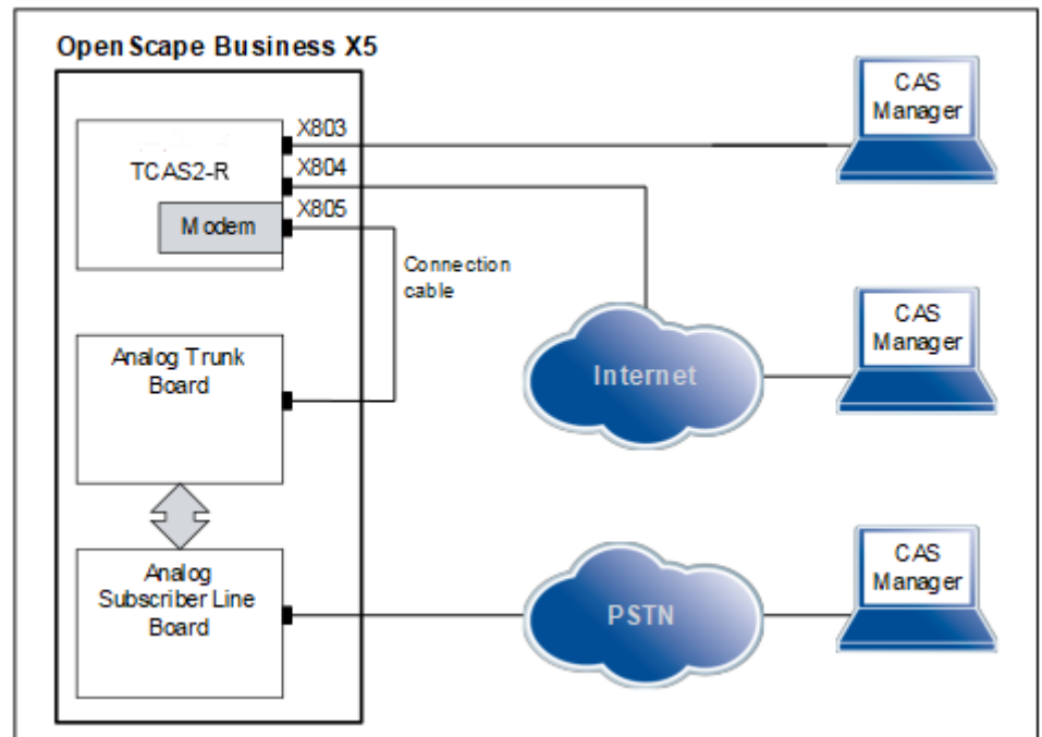
Abbildung 66: TCASR-2 – Zugriffsmöglichkeiten auf die Karten
