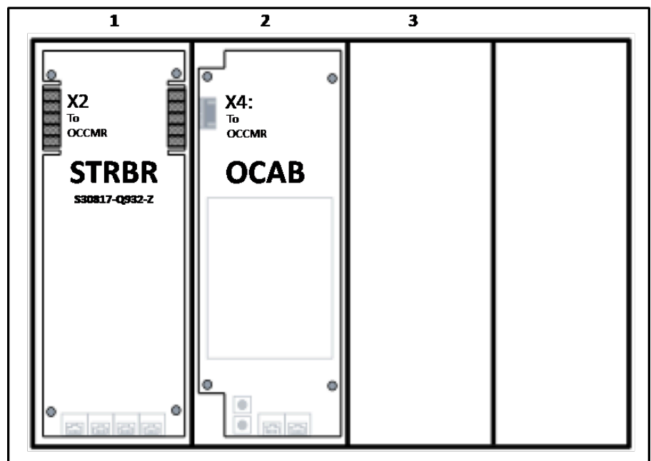
Abbildung 50: STRBR in Option 1 auf Steckplatzebene 3/5 in OpenScape Business X3R/X5R mit OCCMR Mainboard
