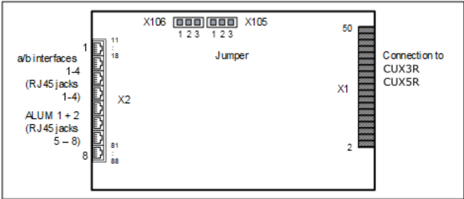
Abbildung 67: TLANI4R
