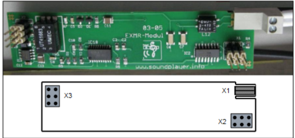
Abbildung 16: EXMR
