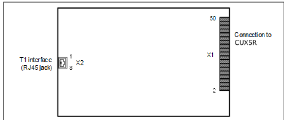
Abbildung 81: TST1R
