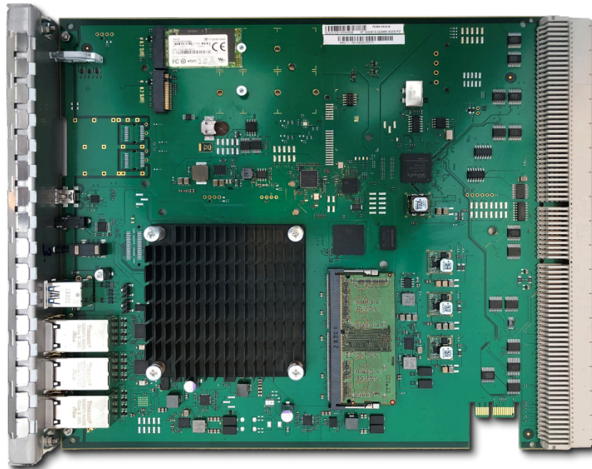
Abbildung 26: OCCLA
