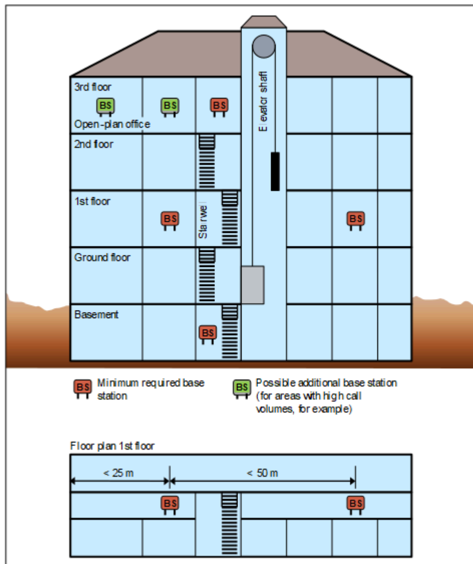
Abbildung 87: Beispiel für die Positionierung von Basisstationen in Gebäuden in Ziegel- und Leichtbauweise
