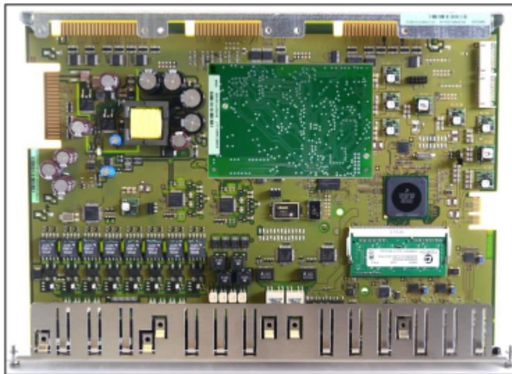
Abbildung 6: CMAe montiert auf OCCMR
