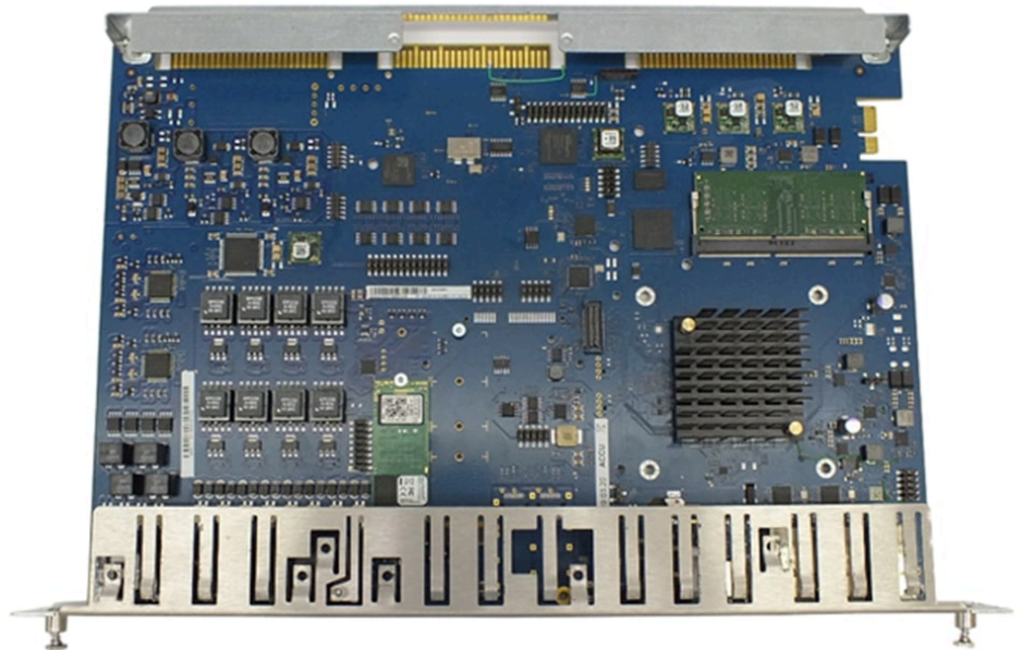
Abbildung 29: OCCMBR
