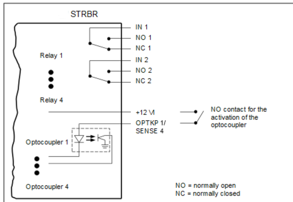
Abbildung 56: STRB, STRBR – Prinzipschaltbild
