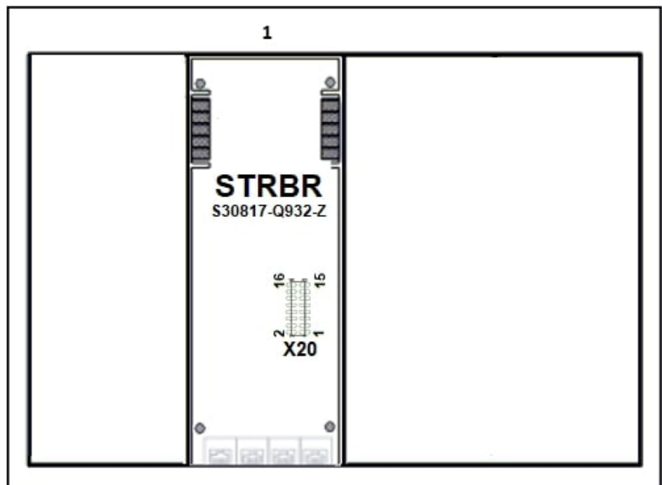
Abbildung 54: STRBR in Option 1 auf Steckplatzebene 3/5 in OpenScape Business X3R/X5R mit OCCMBR/OCCMAR Mainboard
