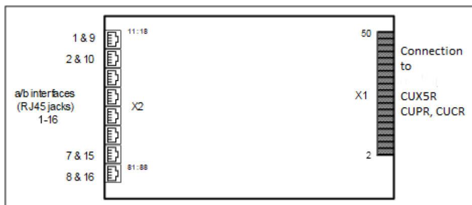
Abbildung 38: SLAV16R
