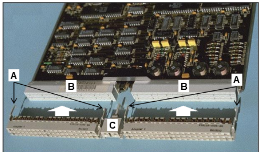
Abbildung 76: Montage des SIVAPAC-SIPAC-Baugruppenadapters
