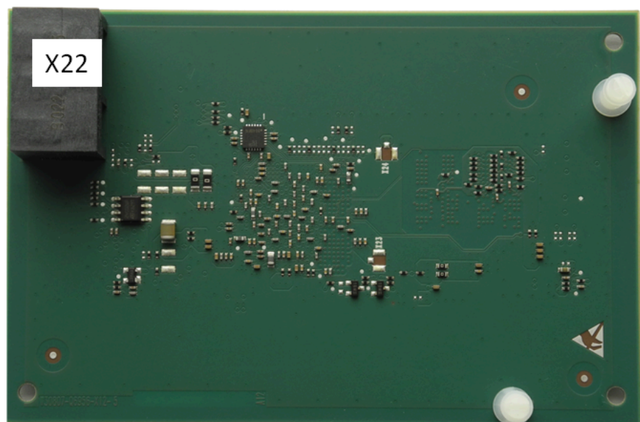
Abbildung 24: Beispiel OCCBL - Rückseite mit gesteckten Abstandsbolzen
