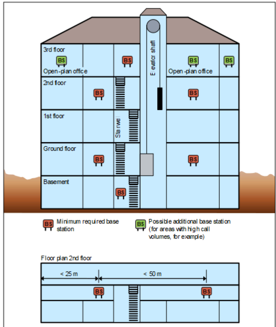
Abbildung 88: Beispiel für die Positionierung von Basisstationen in Stahlbetongebäuden mit einem Innenausbau in Ziegel- und Leichtbauweise
