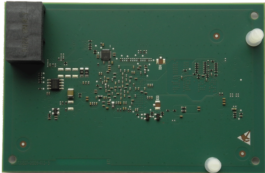
Abbildung 21: Beispiel OCCBL- Rückseite mit gesteckten Abstandsbolzen
