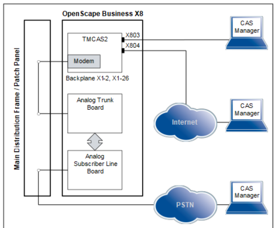
Abbildung 72: TMCAS2 – Möglichkeiten für den Zugriff auf die Baugruppe
