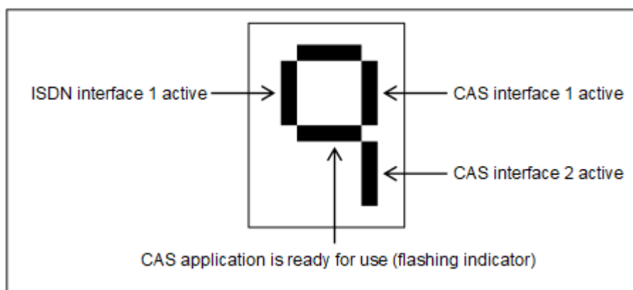
Abbildung 65: TCAS-2, TCASR-2 – Zustände der Schnittstellen und der CAS-Applikation
