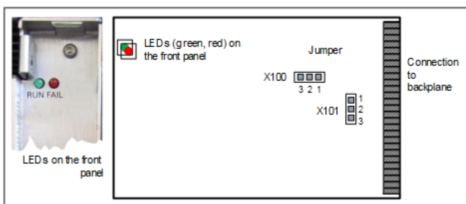
Abbildung 68: TMANI
