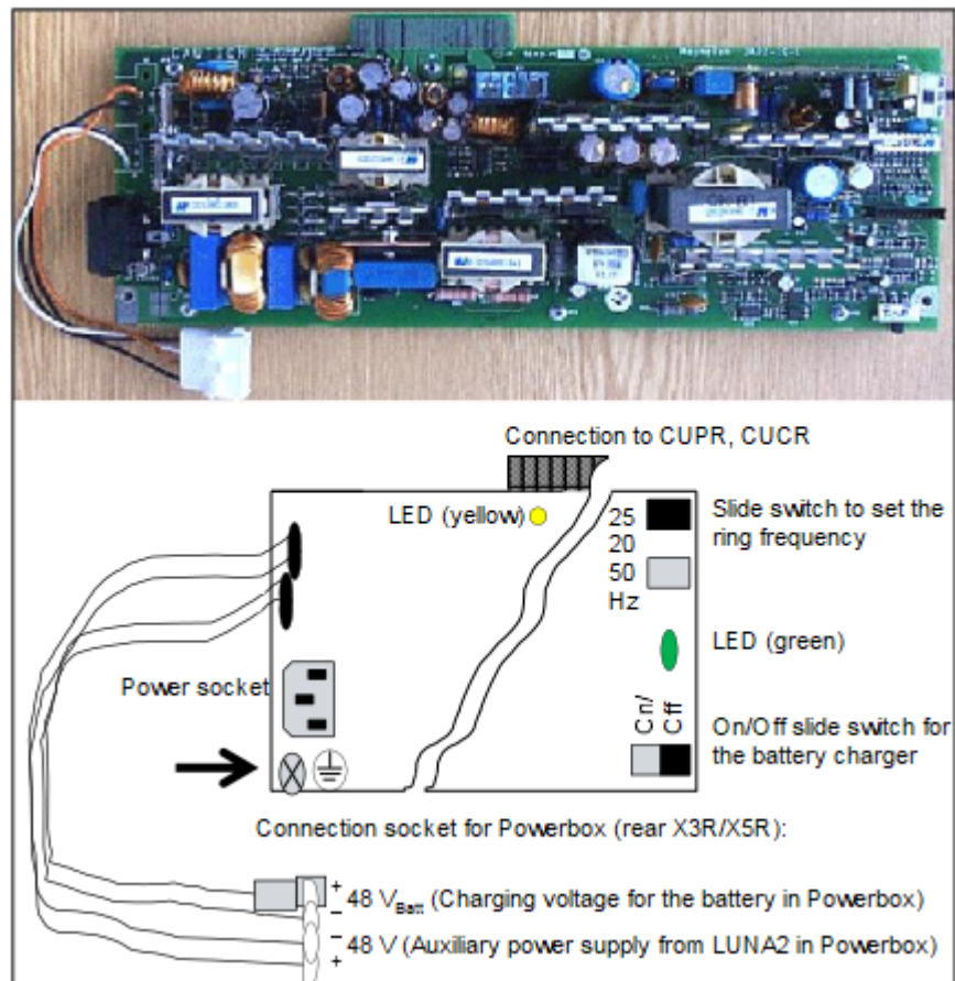
Abbildung 82: UPSC-DR
