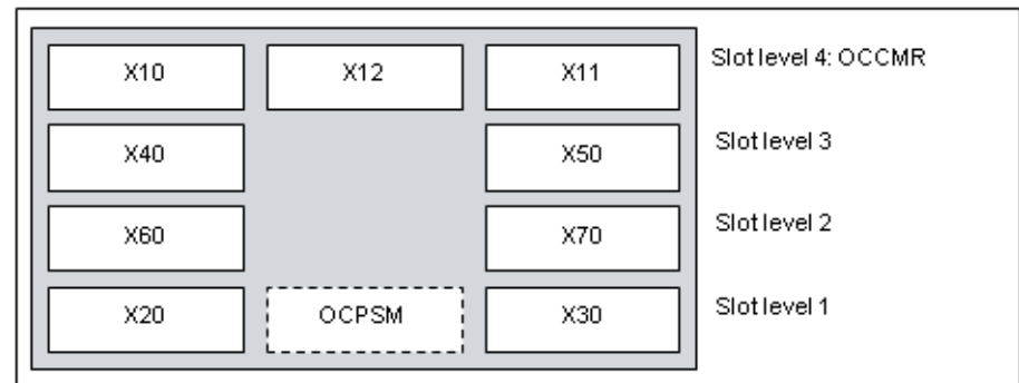
Abbildung 7: CUX5R
