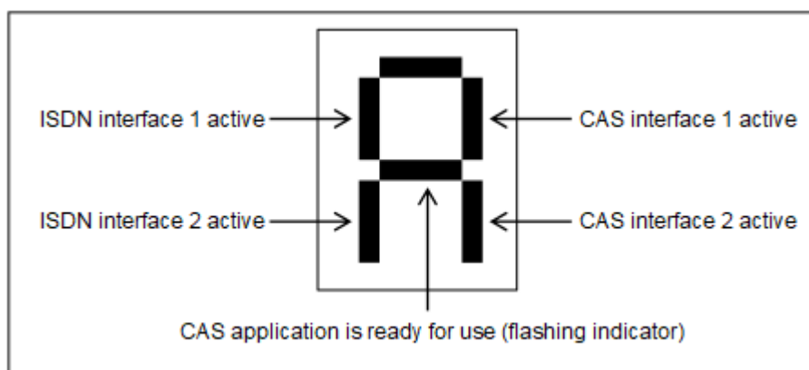
Abbildung 71: TMCAS2 – Zustände der Schnittstellen und der CAS-Applikation
