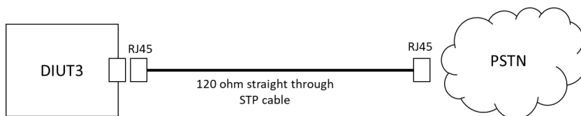
Abbildung 12: Direkter Anschluss per 1:1-Kabel zum PSTN
