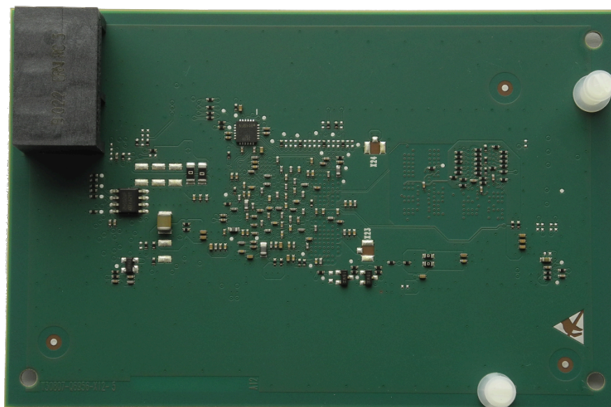
Figura 17: Ejemplo con OCCBL: parte trasera con pernos separadores insertados
