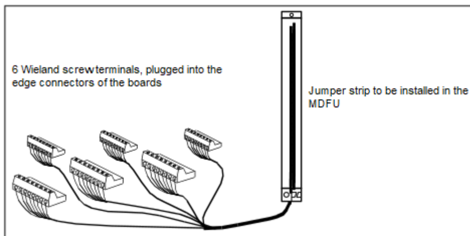
Illustration 26 : CABLU S30269-Z41-A30
