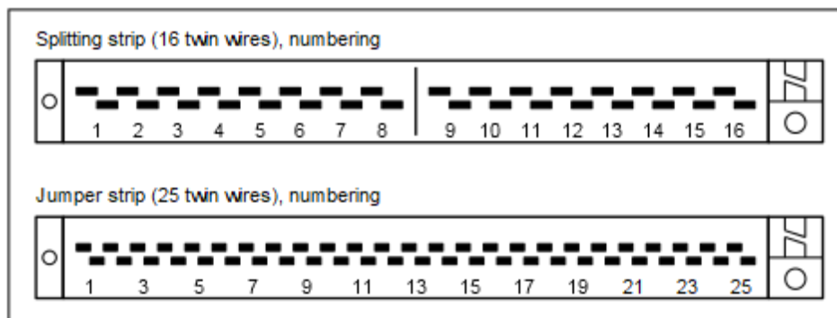
Illustration 25 : Réglette à coupure/réglette de connexion – Numérotation des raccords
