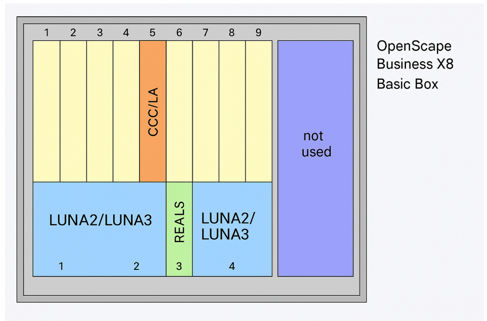
Illustration 16 : OpenScape Business X8 – Emplacements de modules au sein du boîtier de base
