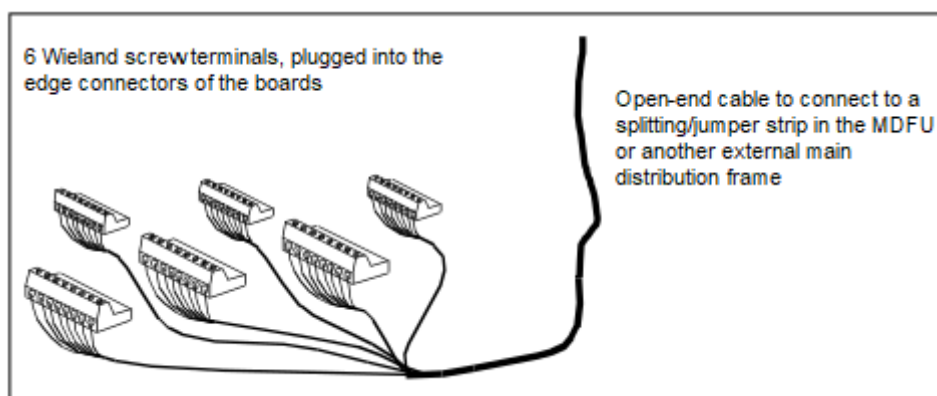
Illustration 27 : Câble open-end S30267-Z322-Axxx
